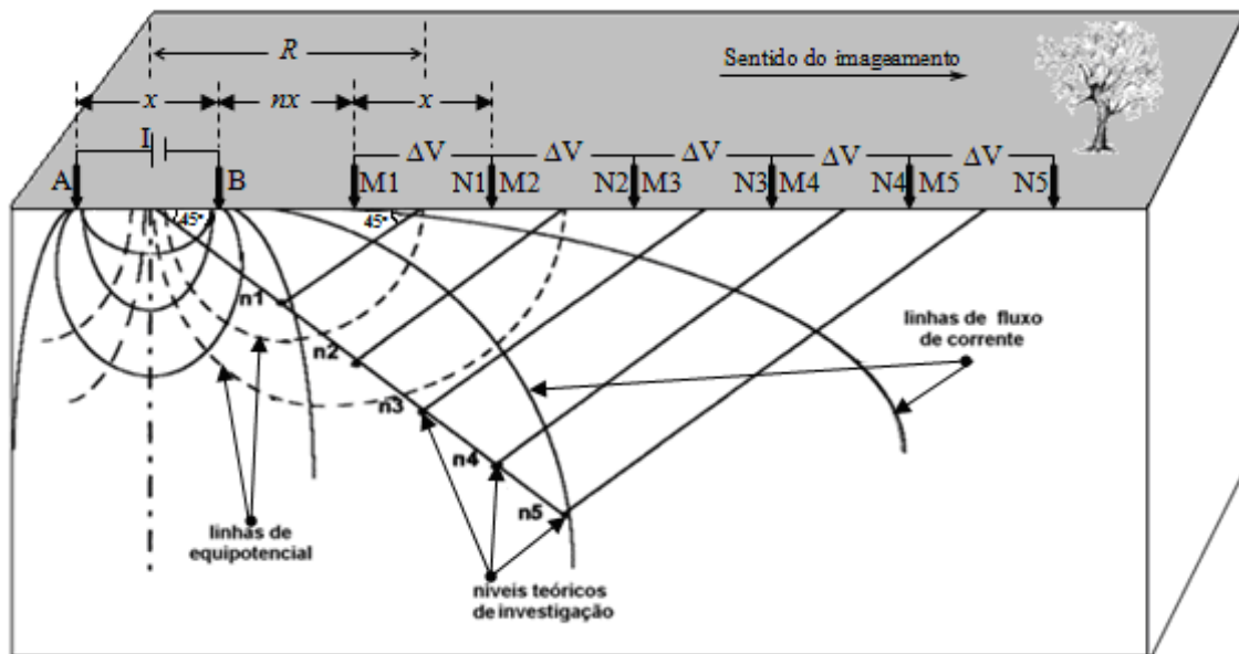
Figura 4.11: Disposição do arranjo dipolo-dipolo (modificado de ELIS, 1998)
