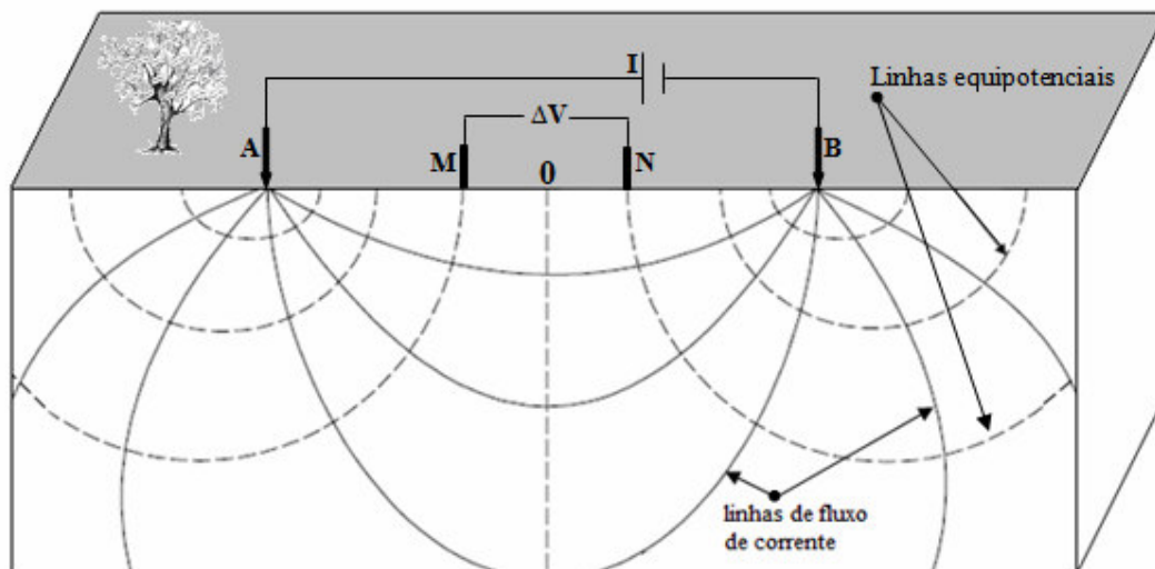
Figura 4.9: Disposição do arranjo Schlumberger (modificado de ELIS, 1998)
