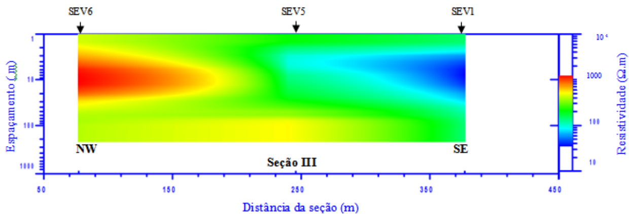
Figura 5.6: Seção de resistividade aparente, obtida a partir das SEVs 1, 5 e 6
