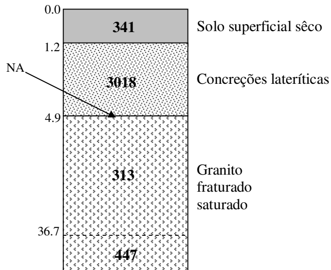
Figura 5.13: Modelo geoeétrico interpretado da SEV6
