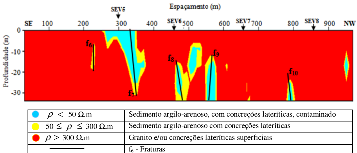
Figura 5.19: Modelo geoeletrico interpretado da linha IE2
