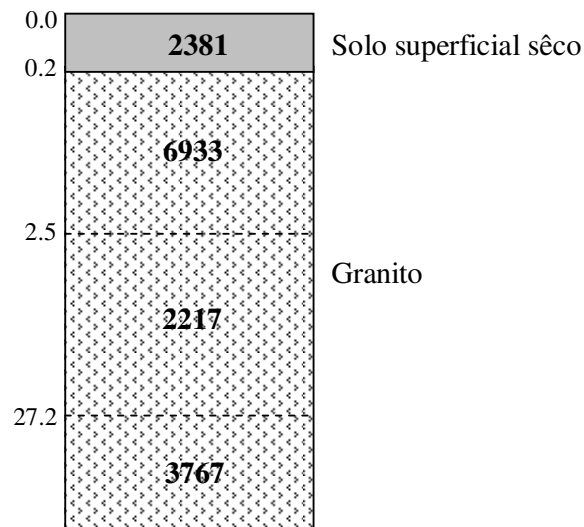
Figura 5.14: Modelo geoeétrico interpretado da SEV9
