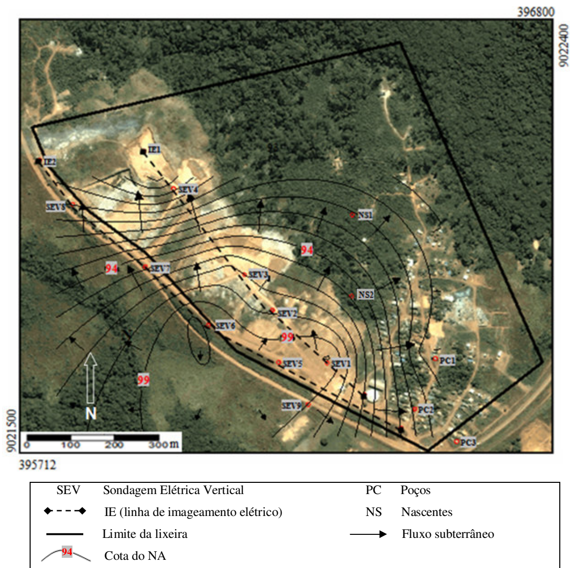
Figura 5.17: Mapa potenciométrico da área da lixeira
