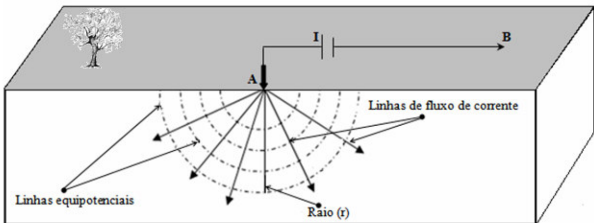
Figura 4.3: Fluxo de corrente de um eletrodo na superfície
