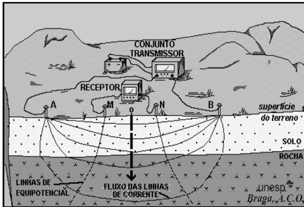
Figura 4.7: Esquema de campo da técnica da SEV (BRAGA, 2001)
