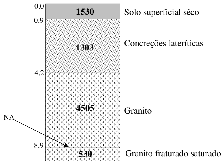
Figura 5.15: Modelo geoeletrico interpretado da SEV7
