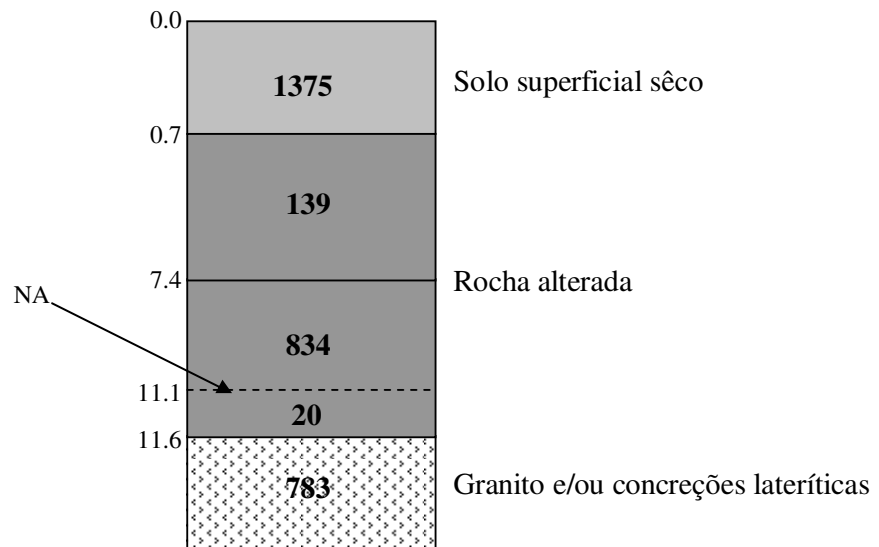
Figura 5.11: Modelo geoeétrico interpretado da SEV4
