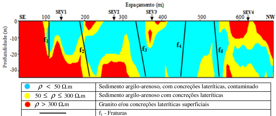
Figura 5.18: Modelo geoeletrico interpretado da linha IE1
