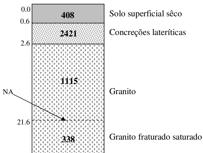
Figura 5.16: Modelo geoeletrico interpretado da SEV8
