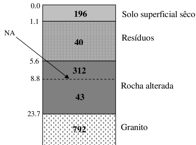
Figura 5.9: Modelo geoeletrico interpretado da SEV2
