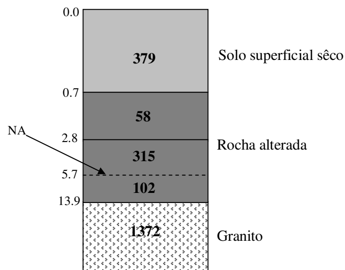
Figura 5.12: Modelo geoeétrico interpretado da SEV5
