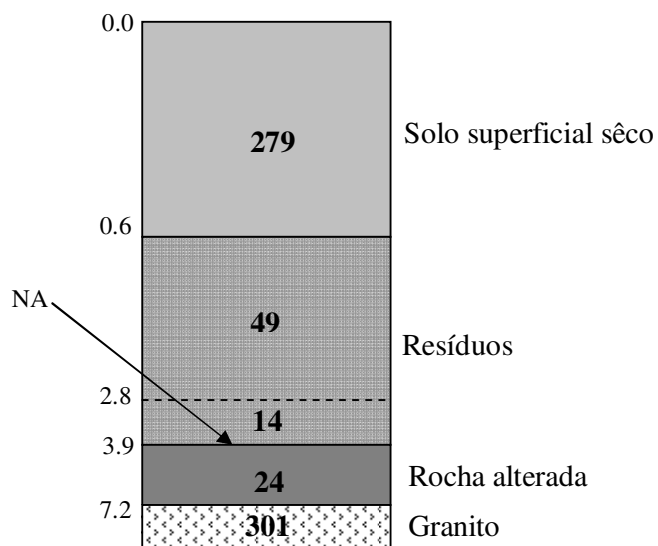
Figura 5.8: Modelo geoeletrico interpretado da SEV1
