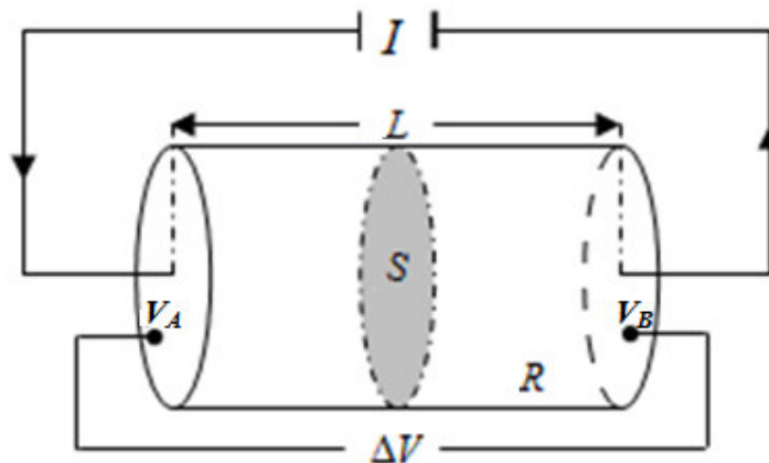
Figura 4.2: Cilindro condutor
