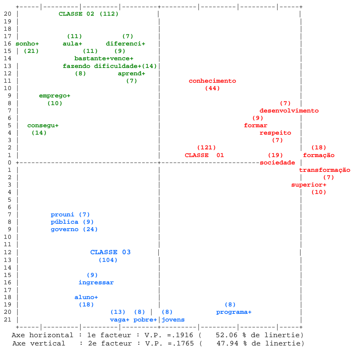
Fig. N° 06 - Projeção das palavras analisadas do arquivo REDAÇÃO VESTIBULAR no plano 1 2 (correlações)
