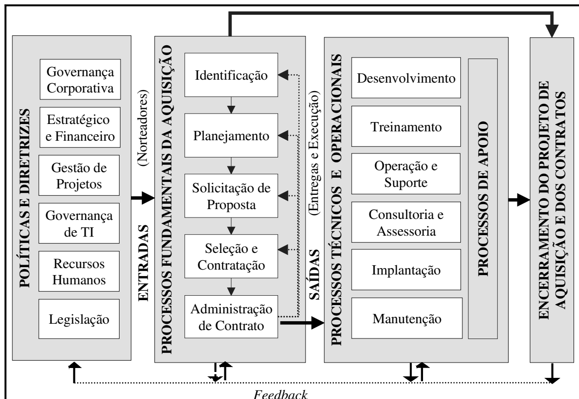
Figura 11 - Modelo para projetos de aquisição de software (versão 2). Fonte: Elaborado pelo autor.
