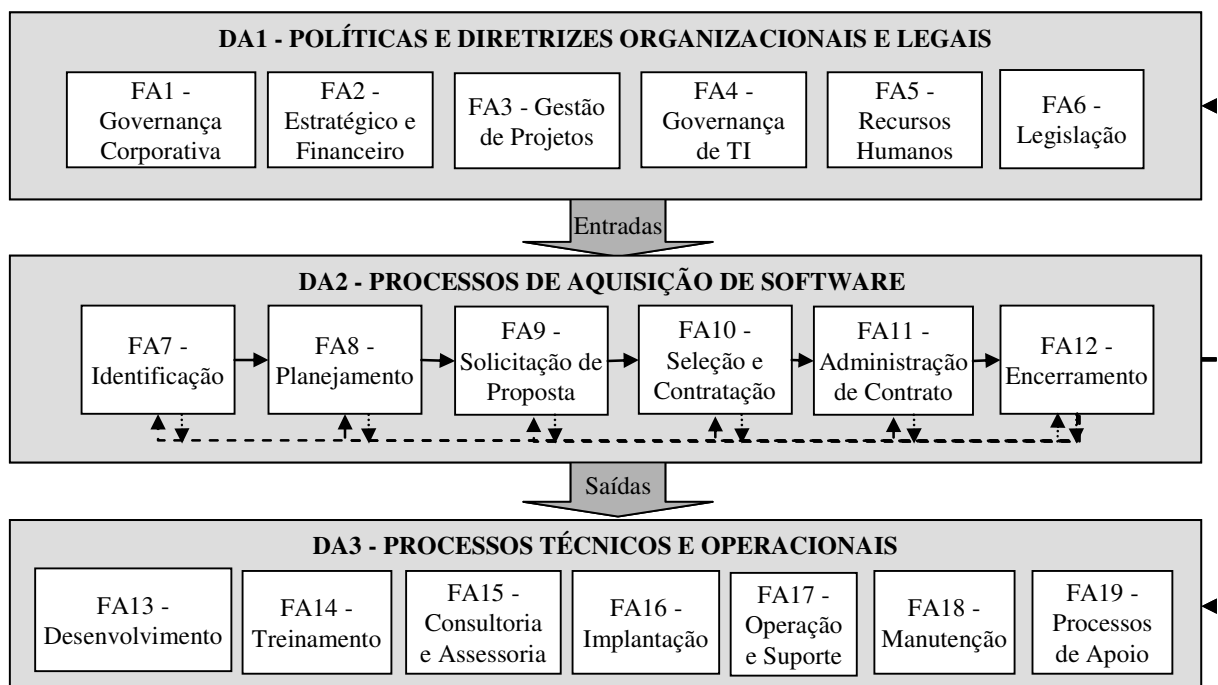
Figura 10 - Modelo para projetos de aquisição de software (versão 1).
