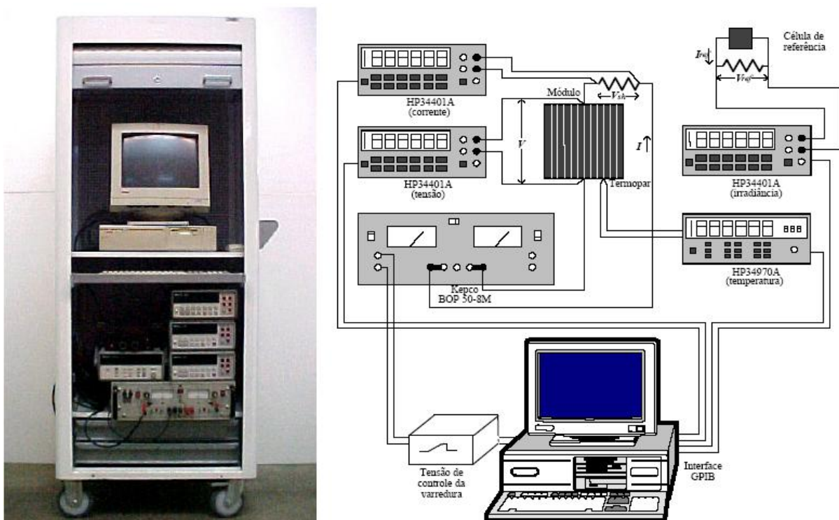
Figura 5.3 - Equipamento utilizado para o ensaio de módulos fotovoltaicos (Krenzinger e Prieb, 2005).
