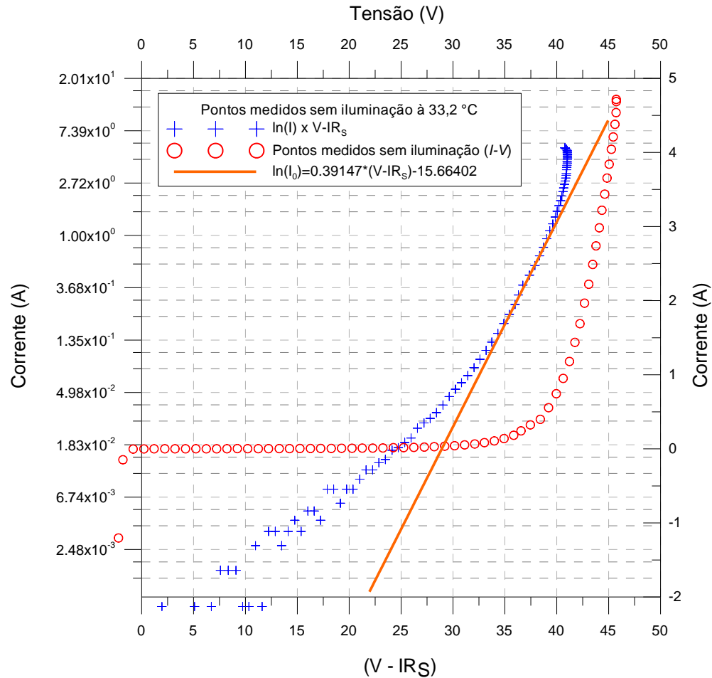
Figura 5.9 - Curvas determinadas a partir de ensaio sem iluminação a 33,2 °C.
