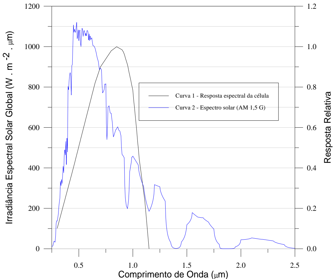
Figura 2.7 - Espectro solar e resposta espectral do silício (adaptado de Hecktheuer, 2001).
