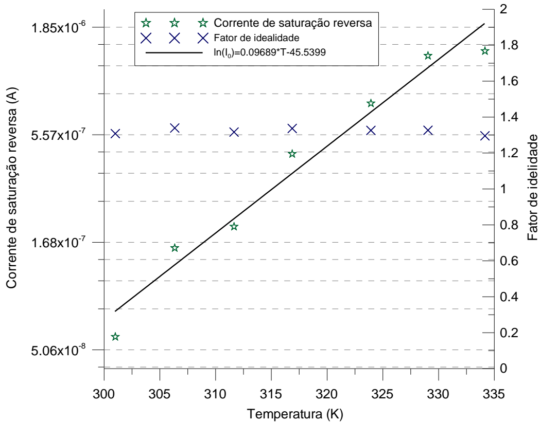
Figura 5.10 - Pontos medidos de \ln(I_0) e m para diferentes temperaturas de um módulo de 100 W de silício monocristalino.
