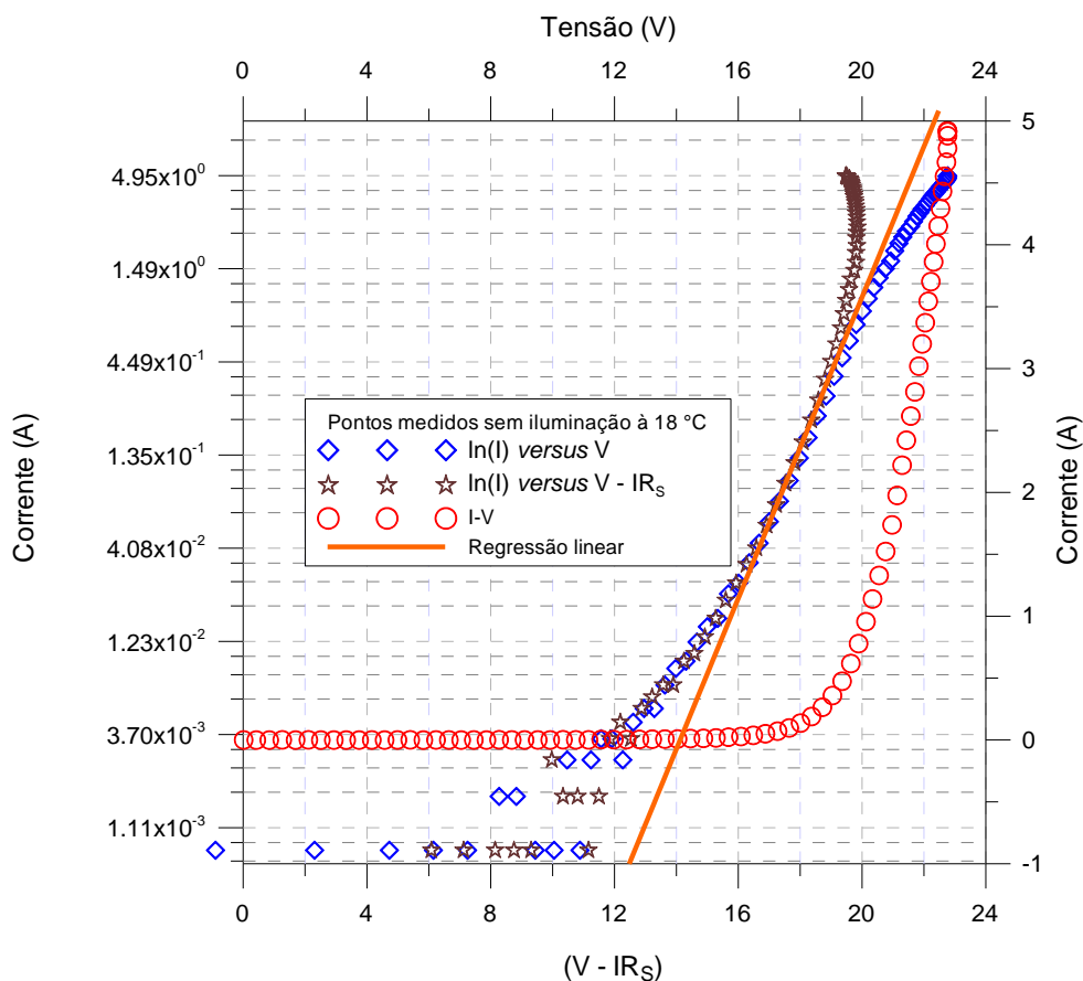
Figura 5.12 - Curvas determinadas a partir de ensaio sem iluminação a 18^\circ\text{C} .
