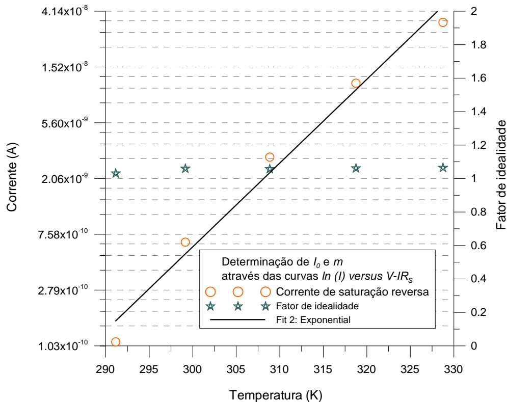
Figura 5.13 - Pontos medidos de \ln(I_0) e m para diferentes temperaturas de um módulo de 50 W de silício monocristalino.
