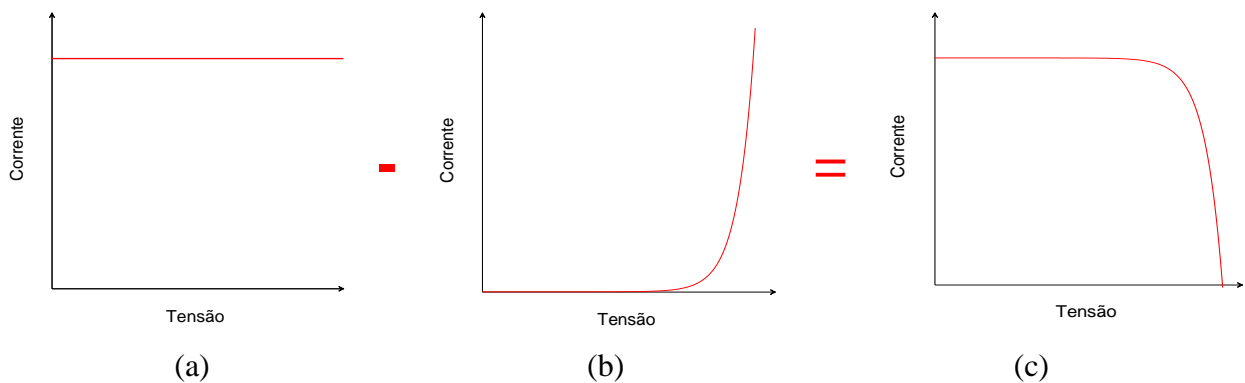
Figura 4.1- Representação da corrente fotogerada (a) curva I - V de um diodo no escuro (b) e da diferença das duas curvas (c).
