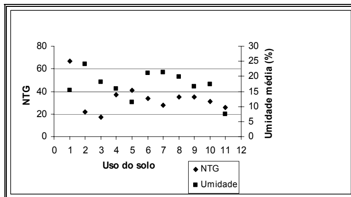
Figura 4.14 - Comportamento do NTG e umidade média no solo Retrabalhados arenosos da serra, com uso: cana de açúcar 1 a 5 .Pastagem 6 a 11,
