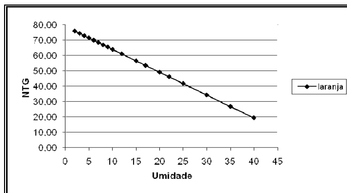
Figura 4.43 - Comportamento da resistência a penetração frente a praticas de pastagem para materiais inconsolidados Residuais da Fm. Serra geral.
