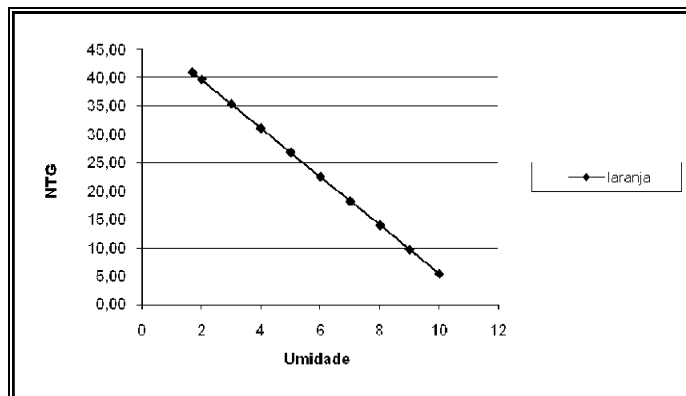
Figura 4.42 - Comportamento da resistência a penetração frente a praticas de laranja para materiais inconsolidados Retrabalhados arenosos com pedregulho.
