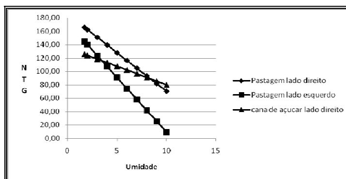
Figura 4.50 - Comportamento da resistência a penetração frente as práticas de cana e pastagem para materiais inconsolidados Retrabalhados em topo, na voçoroca em análise.
