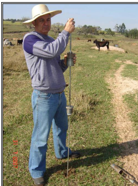
Figura 2.4 – Penetrômetro utilizado na execução dos ensaios in situ.
