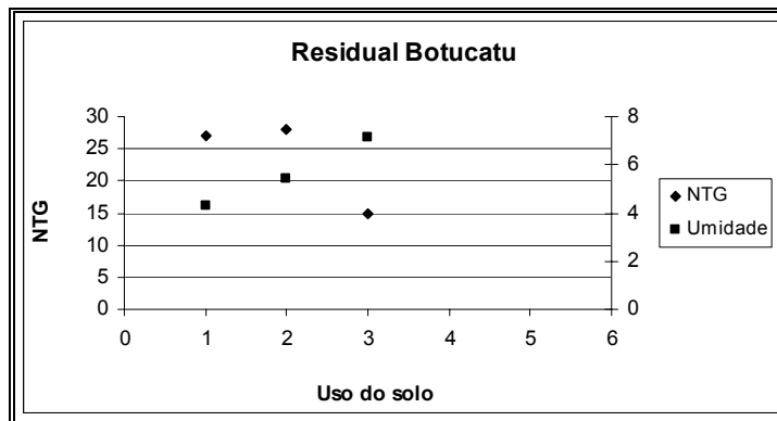
Figura 4.17 - Comportamento do NTG e umidade média no solo Residuais de Botucatu, com uso: pastagem 1 a 4.
