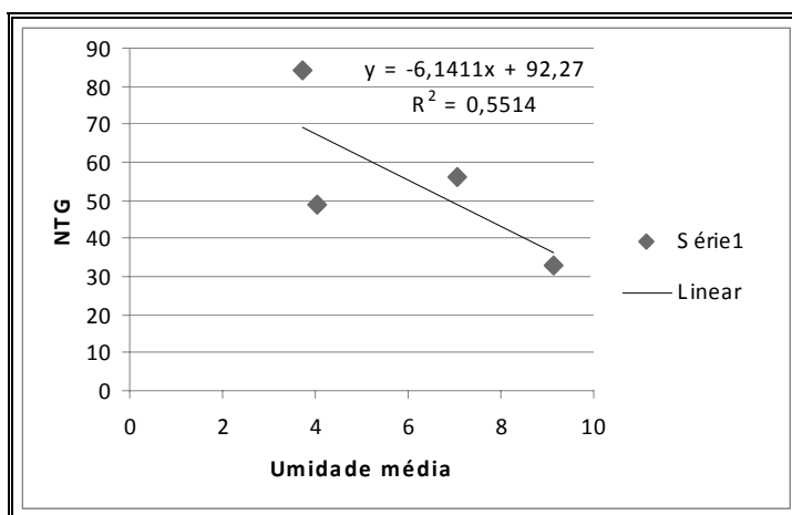
Figura 4.29- Correlação de NTG x Umidade média para as umidades de material, residuais da Fm. Pirambóia considerando o uso do solo: eucalipto.
