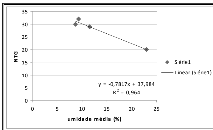
Figura 4.33 – Correlação de NTG x Umidade média para as umidades de material, residuais da Fm. Itaqueri, considerando o uso do solo: cultivo de cana de açúcar.
