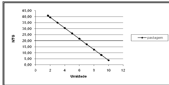
Figura 4.44 - Comportamento da resistência a penetração frente a práticas de pastagem para materiais inconsolidados Residuais da Fm. Botucatu.
