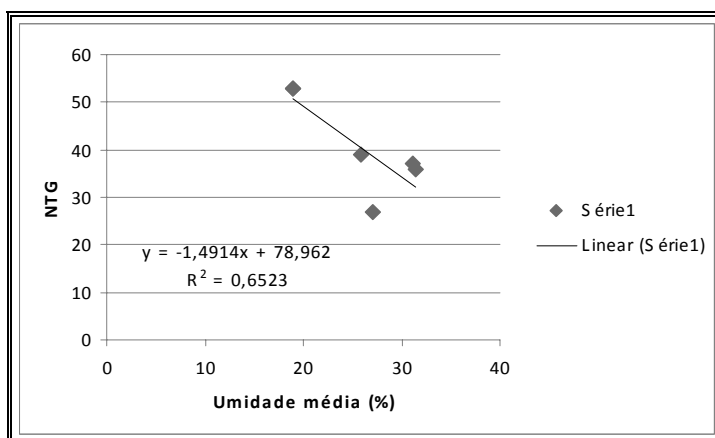
Figura 4.35 - Correlação de NTG x Umidade média para as umidades de material, residuais da Fm. Serra Geral, considerando o uso do solo: pastagem.
