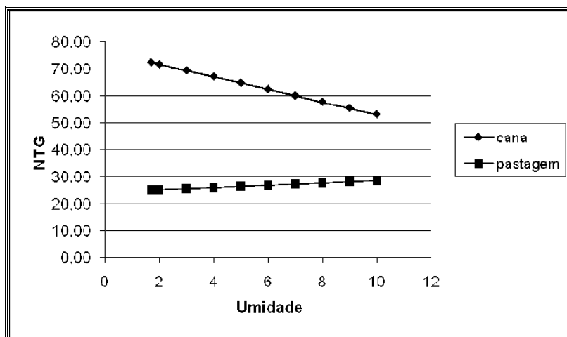
Figura 4.40 - Comportamento da resistência a penetração frente a pratica de cana de açúcar e pastagem, nos materiais inconsolidados Retrabalhados arenosos da serra.
