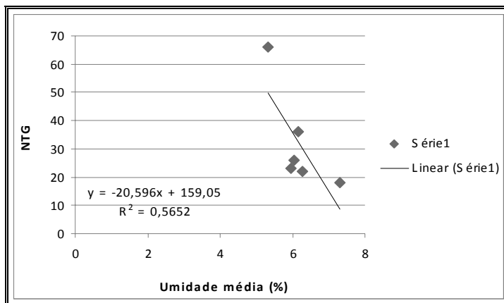
Figura 4.28 – Correlação de NTG x Umidade média para as umidades de material, residuais da Fm. Pirambóia considerando o uso do solo: cultivo de laranja.
