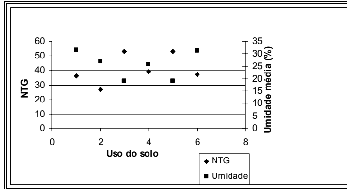
Figura 4.16 - Comportamento do NTG e umidade média no solo Residuais de Serra Geral, com uso: pastagem 1 a 6.
