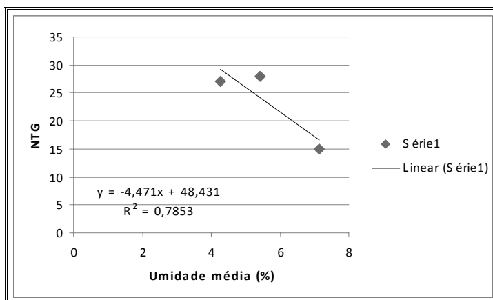
Figura 4.36 – Correlação de NTG x Umidade média para as umidades de material, residuais da Fm. Botucatu , considerando o uso do solo: pastagem.
