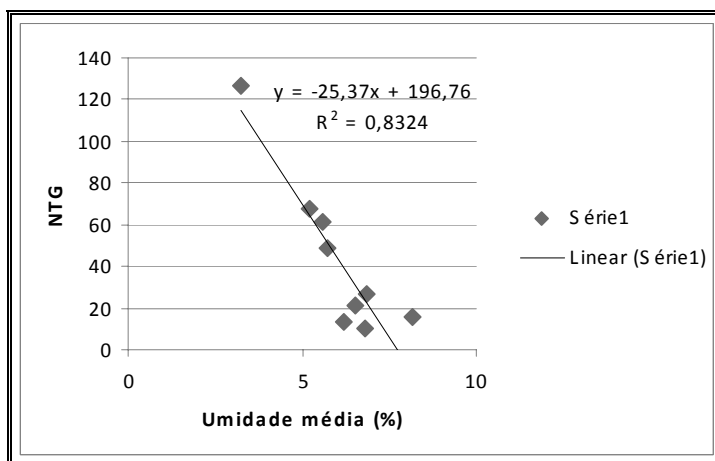
Figura 4.30 – Correlação de NTG x Umidade média para as umidades de material, residuais da Fm. Pirambóia considerando o uso do solo: manejo de pastagem.
