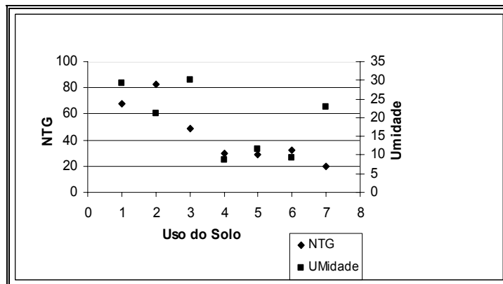
Figura 4.15 - Comportamento do NTG e umidade média no solo Residuais de Itaqueri, com uso: pastagem 1 a 3; Cana de açúcar 4 a 7.
