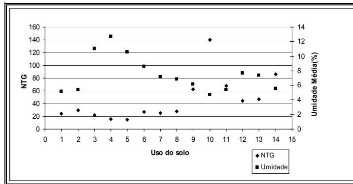
Figura 4.13 - Comportamento do NTG e umidade média no solo Retrabalhados arenoargilosos, com uso: pastagem 1 a 8 cana de açúcar 9 a 14.
