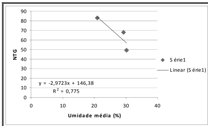
Figura 4.34 – Correlação de NTG x Umidade média para as umidades de material, residuais da Fm. Itaqueri , considerando o uso do solo: pastagem.
