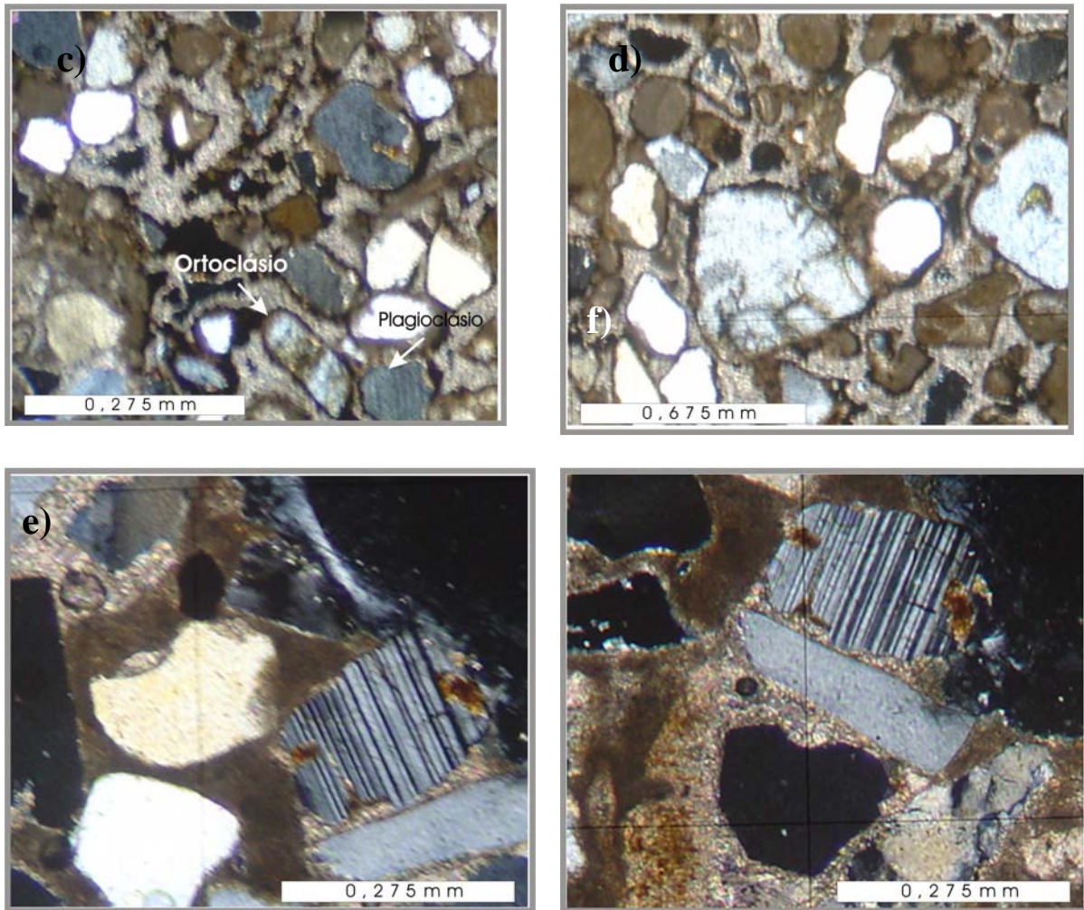
Figura 4.14 - Fotografias de lâminas da Estação Minhoto 2. a) Feldspato apresentando alteração no seu interior; b) Grãos de quartzo mostrando bordas arredondadas; c) Ortoclásio alterado e plagioclásio com geminação polissintética; d) visão mostrando locais com grão mal selecionados; e) Plagioclásio com geminação polissintética; f) Fragmento de rocha contendo quartzo, feldspato e frag. Rocha pré-existente. Fotos: Izaac Cabral Neto.
