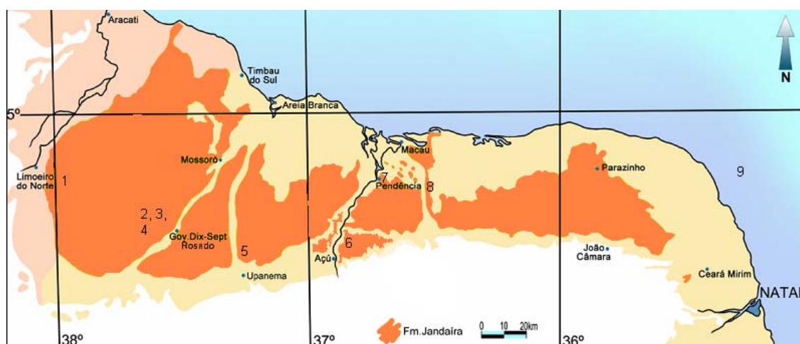
Figura 4.03 -. Localização das ocorrências de corais cretáceos na baía potiguar (1 a 8); ocorrência de estromatoporoides, 8; localização de corais holocenicicos, 9. Numeração de acordo com a tabela 4.1.
