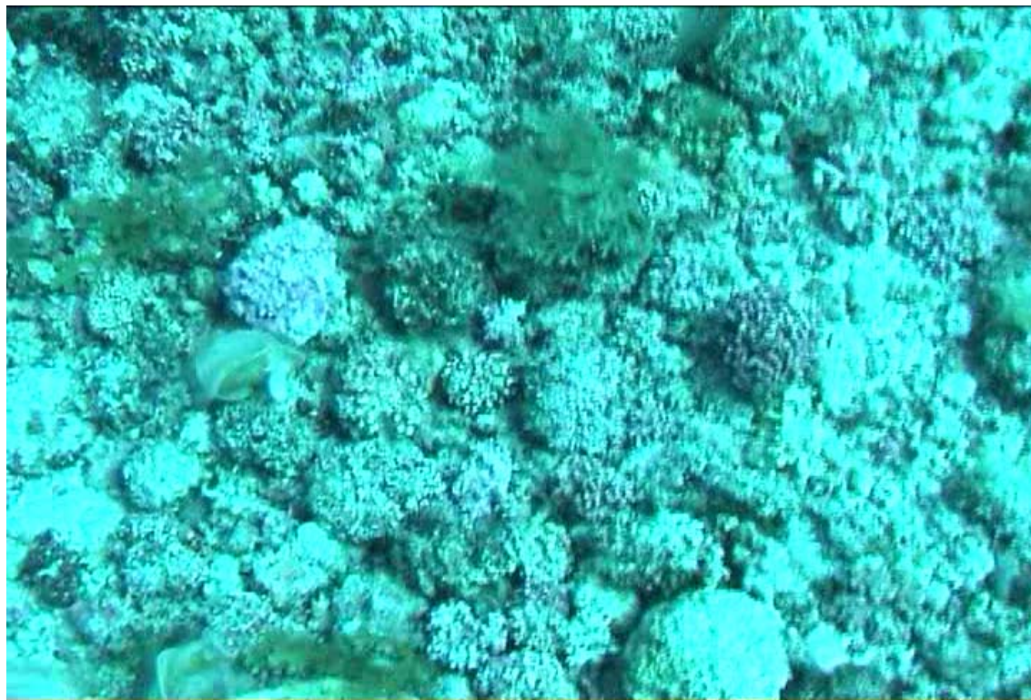
Figura 4.08 – Sedimentos bioclásticos compostos por rodolitos.
