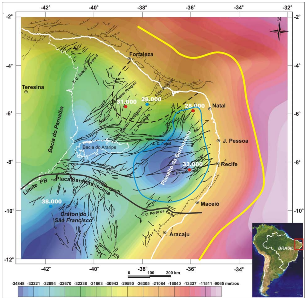
Figura 8.2: Espessuras da crosta da Província Borborema (PB), da margem continental adjacente e do norte do Cráton do São Francisco (CSF), com superposição das principais zonas de cisalhamentos e das falhas normais da margem continental. Imagem sombreada (Inc. = 35°, Dec. = 315°Az). O traço amarelo é o limite inferido para a interface crosta continental-crosta oceânica. O traço azul contínuo é o limite do Planalto da Borborema. O traço preto descontínuo é o limite da Depressão Sertaneja. A linha de sutura colisional entre a PB e a Placa Sanfranciscana está indicada.
