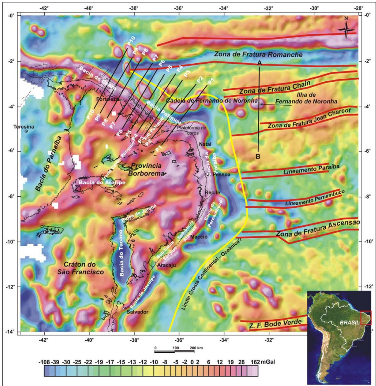
Figura 6.16: Anomalia ar-livre em malha interpolada com dimensão de 10 x 10 km pelo método de mínima curvatura a partir dos pontos da Figura 3.1. Imagem sombreada (Inc. = 35°, Dec. = 315°Az). Os traços pretos correspondem aos perfis de anomalia Ar-livre e topográficos empregados no cálculo da admitância gravitacional da Margem Continental Equatorial. Os dados dos perfis foram amostrados com um espaçamento de 10 km. As províncias, as bacias principais e as zonas de fraturas oceânicas estão indicadas. O traço amarelo é uma inferência do limite entre as crostas continental e oceânica. O Perfil A-B teve como objetivo investigar especificamente o monte submarino da Ilha Fernando Noronha.
