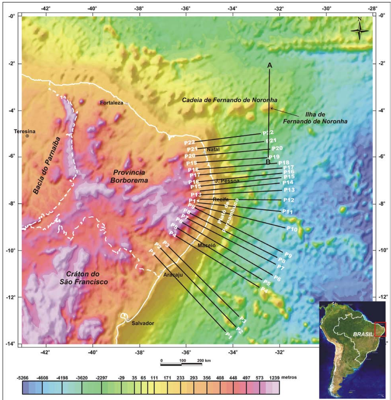
Figura 6.10: Superfície digital da elevação em malha interpolada com dimensão de 5 x 5 km pelo método de mínima curvatura a partir da junção dos dados SRTM no continente com os dados processados por Sandwell & Smith (1997) no oceano. Imagem sombreada (Inc. = 35°, Dec. = 315°Az). Os traços pretos correspondem aos perfis de anomalia ar-livre e topográficos/batimétricos empregados no cálculo da admitância gravitacional da Margem Continental Leste. Os dados dos perfis foram amostrados com um espaçamento de 10 km. O Perfil A-B teve como objetivo investigar especificamente o monte submarino da Ilha Fernando Noronha. A linha branca tracejada é o limite da Província Borborema na definição clássica de Almeida et al. (1977).
