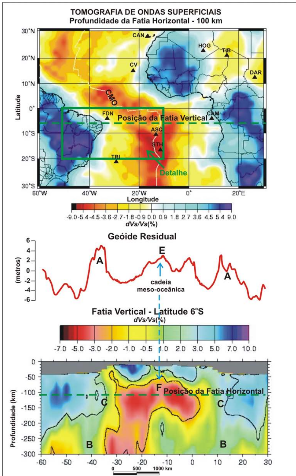
Figura 9.14: Correlação dos dados de tomografia de ondas superficiais com anomalias do geóide residual. Folia Vertical na Latitude -6^{\circ} e a Folia Horizontal localizada 100 km abaixo da Moho . CMO - Cadeia Meso-oceânica; PB - Província Borborema; CSF - Cráton do São Francisco. Possível hot spots : FDN - Fernando de Noronha; ASC - Ascensão; STH - Santa Helena; TRI - Trindade; CAN - Canárias; CV - Cabo Verde; CAM - Camarões; HOG - Hoggar; TIB - Tibesti; DAR - Darfur. Explicações no texto.
