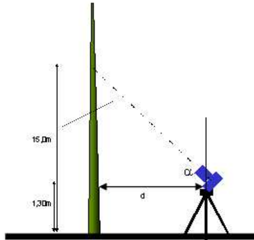
Figura 1.2: Inclinação da câmera em ângulo pré-definido.
