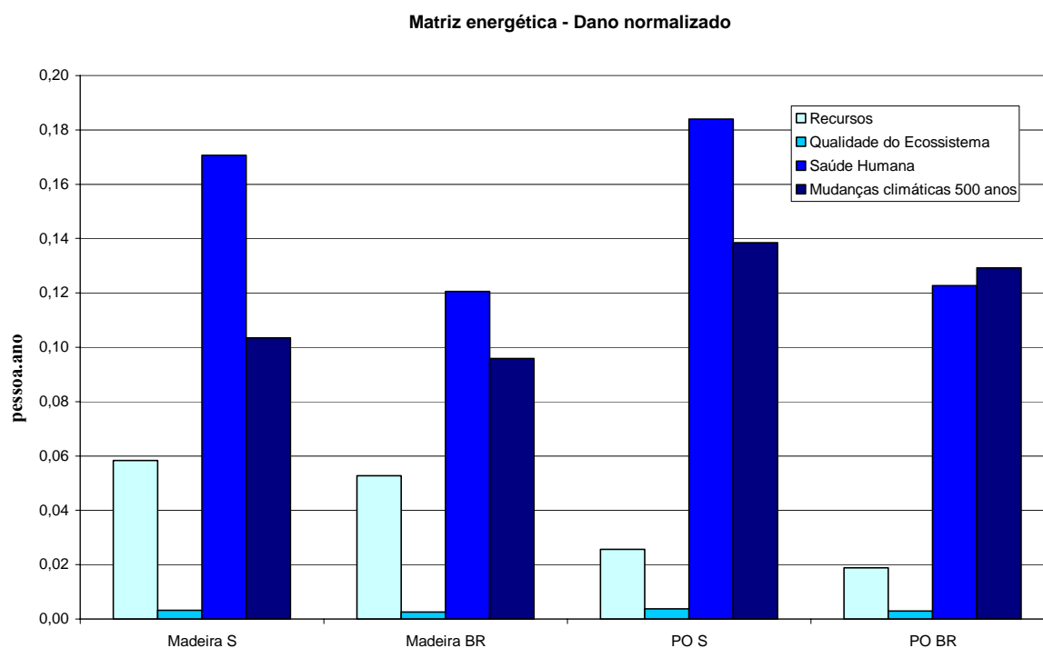
Figura 4.31 Escores de dano normalizado para os diferentes cenários relacionados à matriz energética. Unidade: pessoa.ano.
