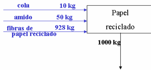
Figura 4.12 Fluxograma do processo de fabricação de papel reciclado. Unidade: kg de produto por tonelada de papel reciclado produzido.
