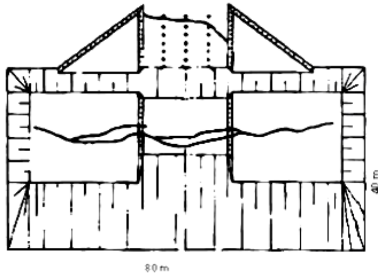
Figura 2.16 – Geometria do aterro e localização das trincas (Ortigão, 1980)
