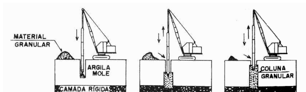
Figura 2.10 – Processo de Vibro-substituição (Almeida, 1996)
