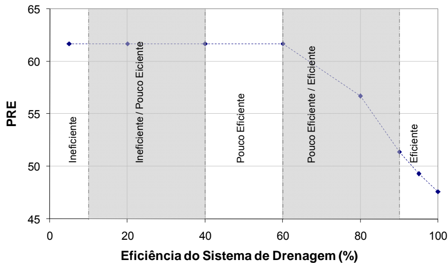
Figura 5.7. Variação de PRE com a Eficiência do Sistema de Drenagem
