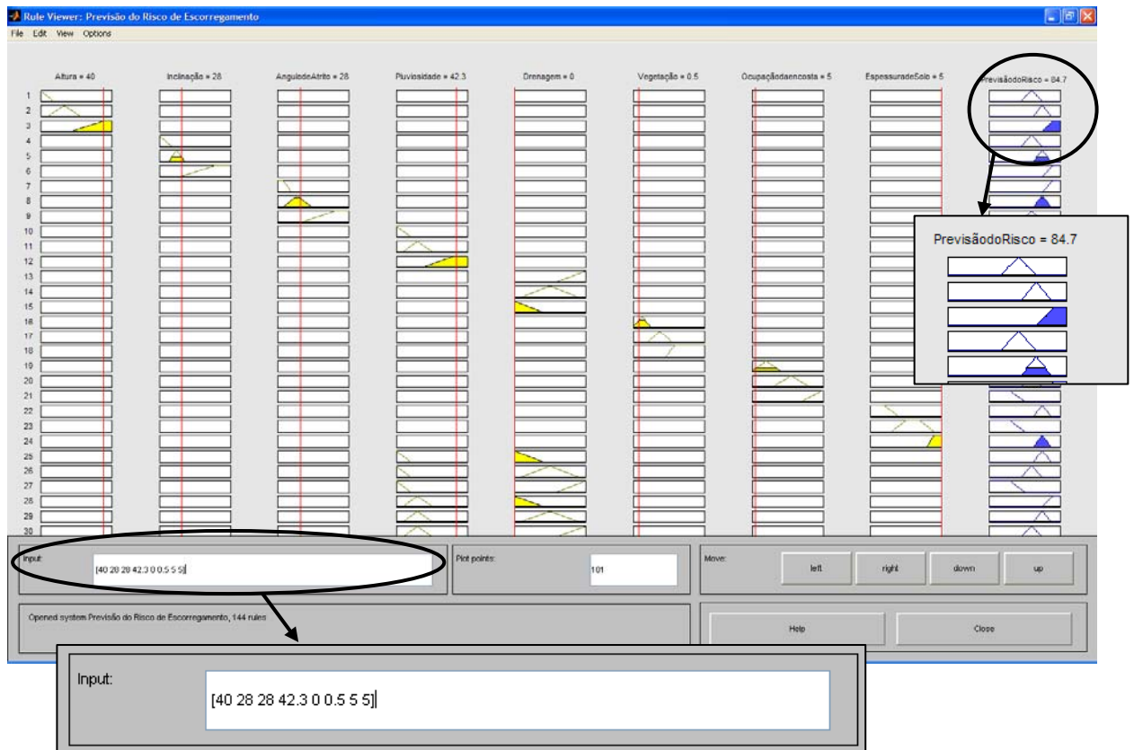
Figura 6.4. Análise Fuzzy para a Situação Após o Escorregamento
