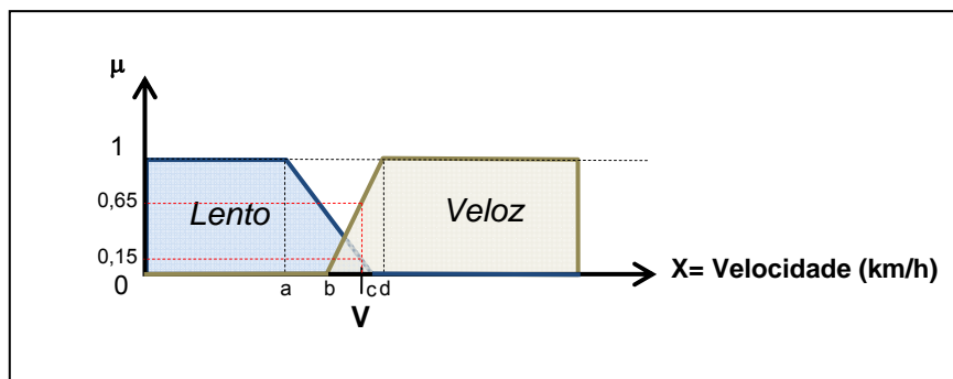
Figura 3.3. Exemplo em Lógica Nebulosa
