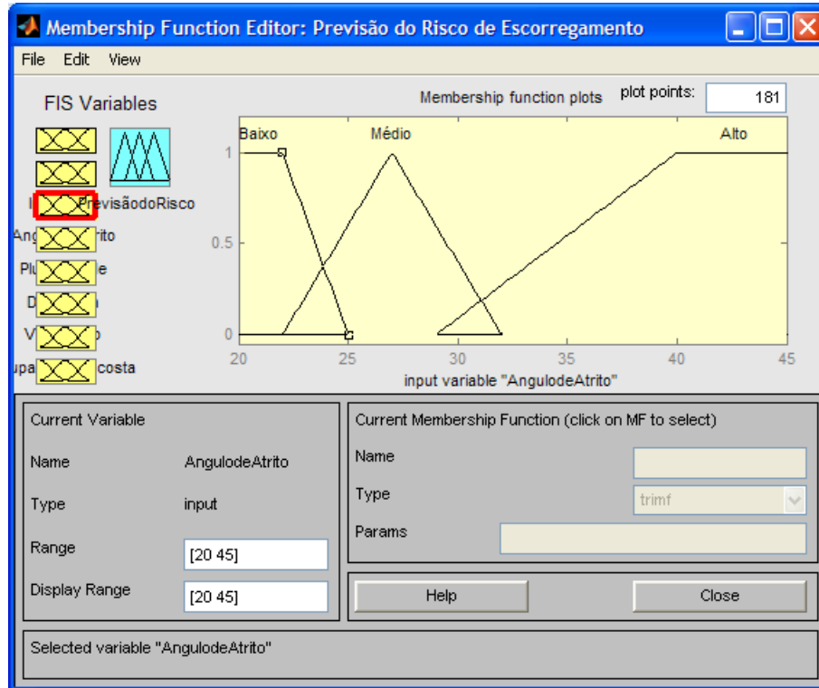
Figura 4.11. Funções de Pertinência dos Adjetivos da Variável Ângulo de Atrito
