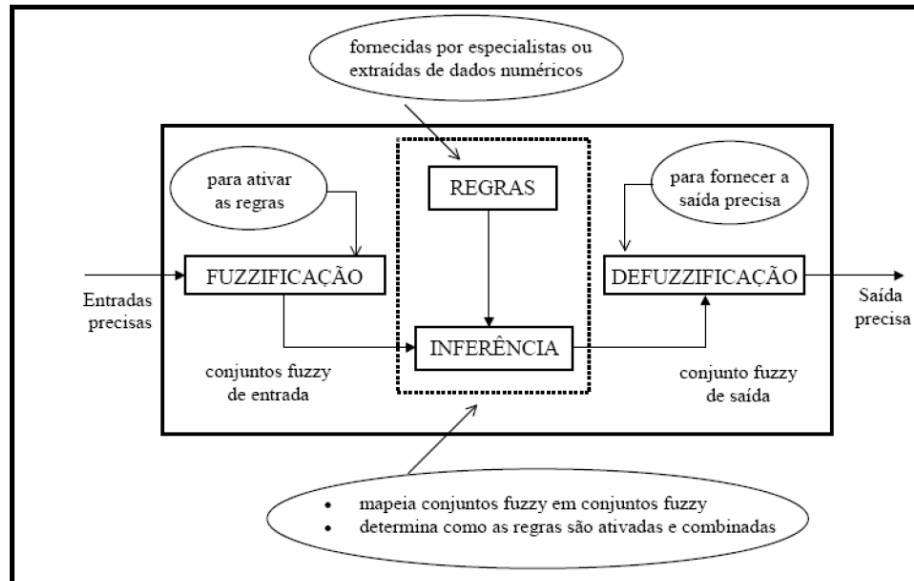
Figura 3.4. Sistema de Inferência Fuzzy (Tanscheit, 1995)
