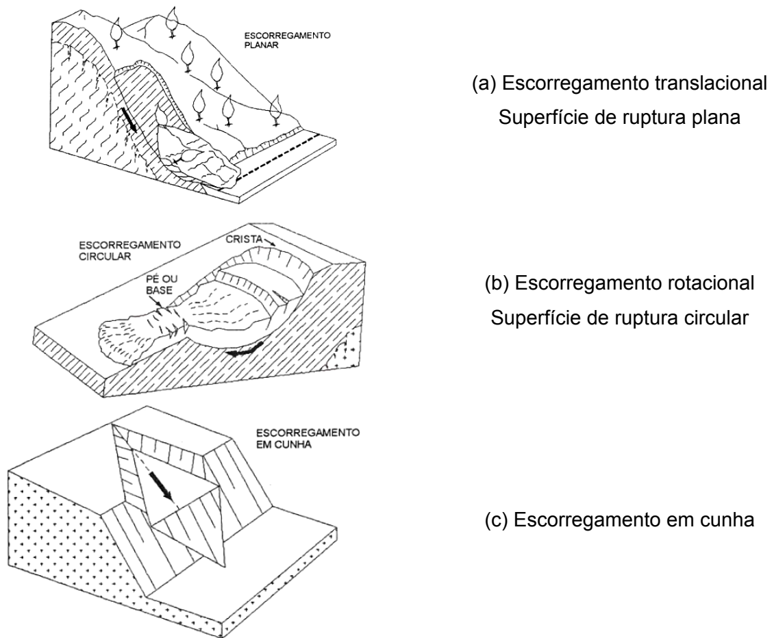
Figura 2.2. Tipos de escorregamento (Infanti Jr. & Fornasari Filho, 1998)
