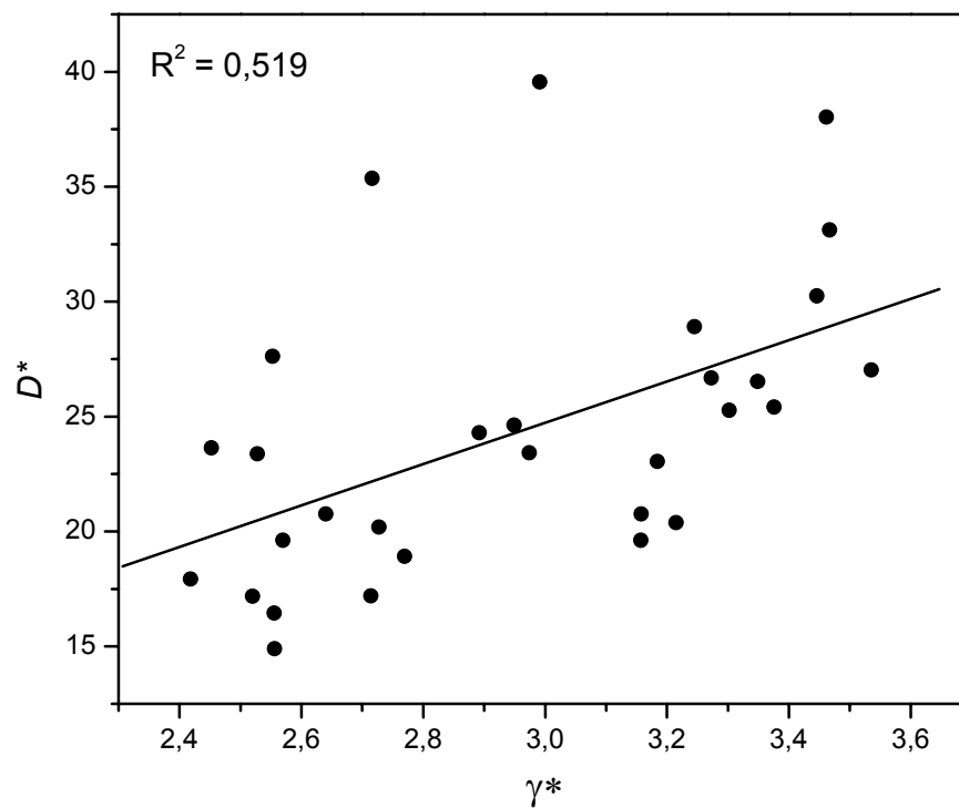
Figura 3.5 Relação entre os parâmetros D^* e \gamma^* , mostrando uma moderada correlação entre a termodinâmica e a cinética nas ligas formadoras MAGV
