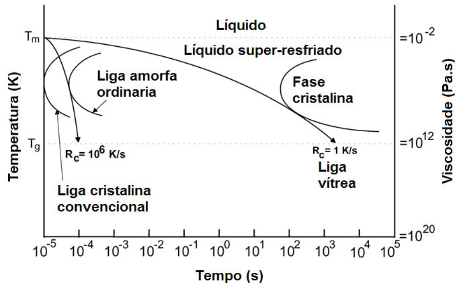
Figura 2.5 Diagrama esquemático mostrando a alta estabilidade térmica dos MAGV quando comparados aos amorfos convencionais [17].
