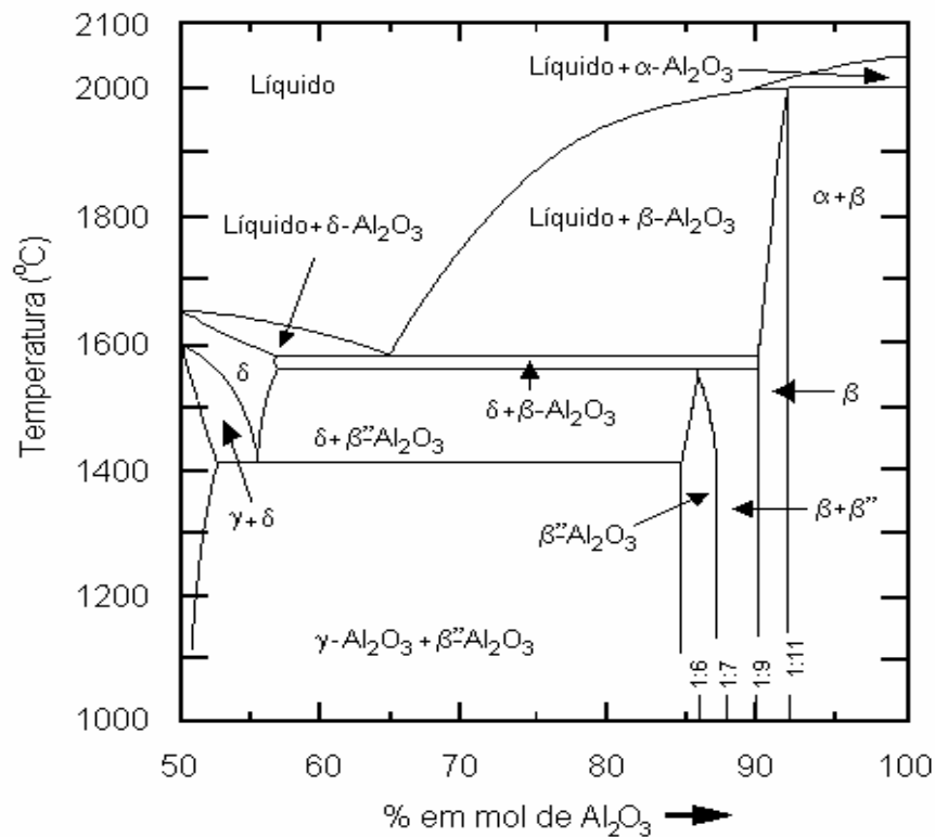
Figura 2.11 - Diagrama de equilíbrio binário entre \text{Na}_2\text{O} e \text{Al}_2\text{O}_3 , figura adaptada de Vandecruys [36].
