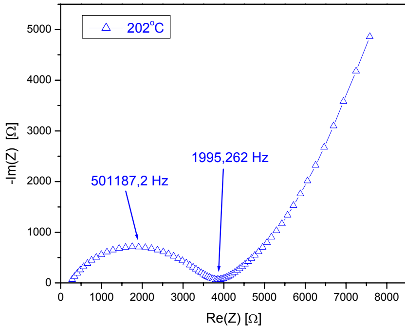
Figura A.3 - Espectro de impedância da amostra de Na β-alumina.
