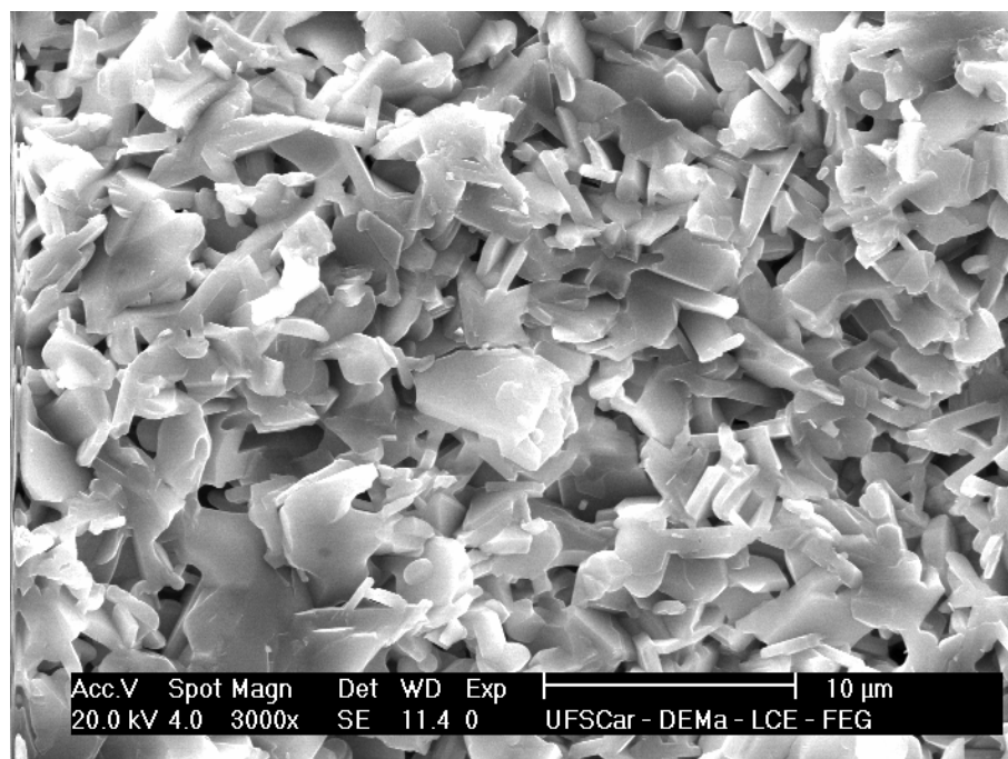
Figura 4.17 - Micrografia de fratura da amostra de Na-β-Alumina conformada por colagem de barbotina e sinterizado na condição de 1650°C com patamar de 4 horas.
