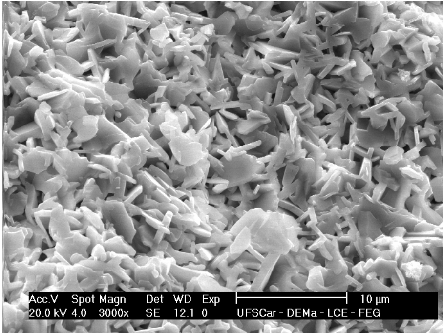
Figura 4.19 - Micrografia de fratura da amostra de La-β-Alumina conformada por prensagem isostática a frio e sinterizado na condição de 1650°C com patamar de 4 horas.
