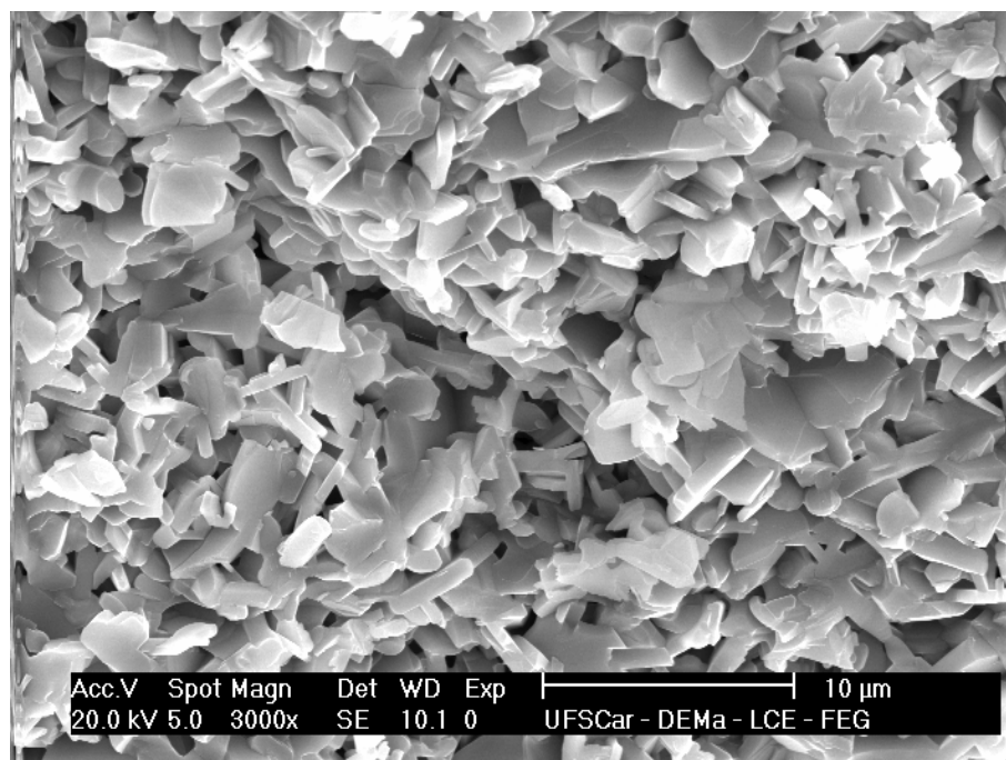
Figura 4.16 - Micrografia de fratura da amostra de Na-β-Alumina conformada por prensagem isostática a frio e sinterizado na condição de 1650°C com patamar de 4 horas.
