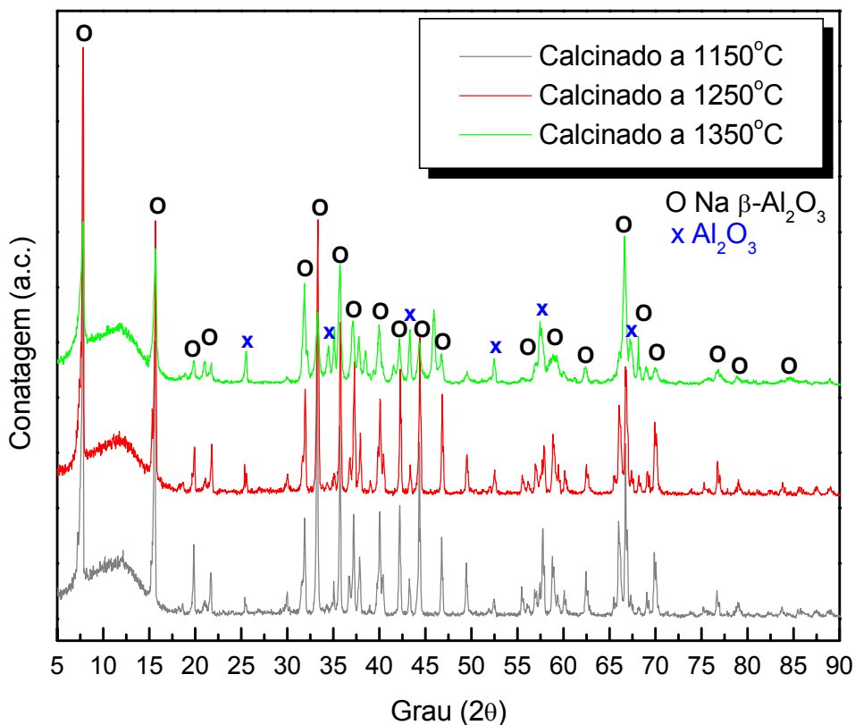
Figura 4.1 - Difratoograma de raios X dos pós de Na- \beta -alumina calcinados em diferentes condições de temperatura.
