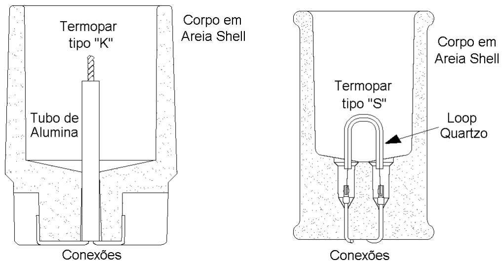
Figura 2.4 - Copos utilizados para análise de teor de silício, carbono e carbono equivalente por meio da curva de resfriamento [12].
