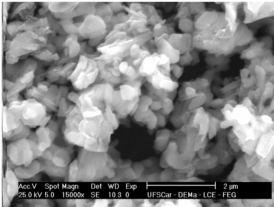
Figura 4.4 - Aspecto geral do pó de Na-β-Alumina após processo de calcinação (1150°C/4horas) seguido de moagem (moinho de bolas com relação de 10:1 entre meios de moagem e material durante 8 horas)
