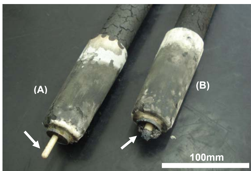
Figura 4.30 - Exemplo de sensor que (A) resistiu imersão e (B) não resistiu a imersão ao banho metálico.
