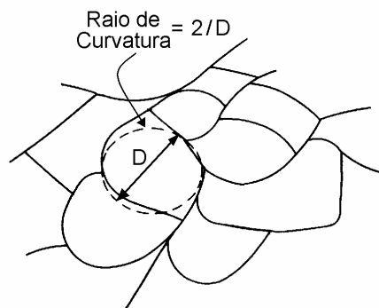
Figura 4.23 - Relação entre o tamanho de grão e diâmetro D .
