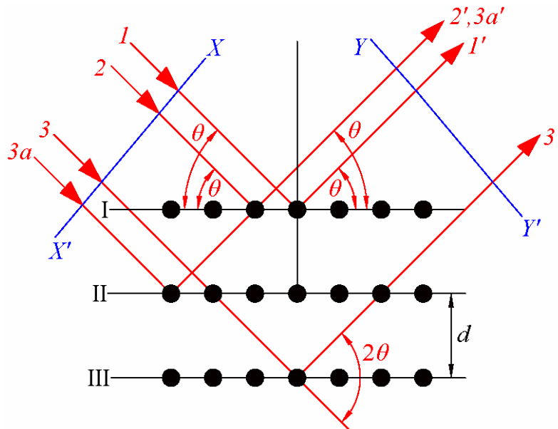
Figura 2.15 - Esquema ilustrando a difração dos feixes de raios X quando este incide sobre um reticulado cristalino [67].
