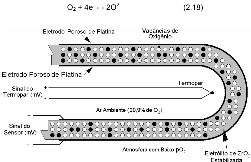
Figura 2.7 - Sensor de oxigênio para monitoramento de exaustão de gases em escapamento de automóveis [28].
