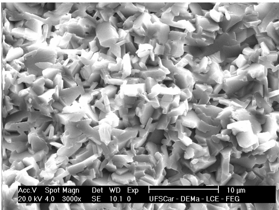
Figura 4.20 - Micrografia de fratura da amostra de La-β-Alumina conformada por colagem de barbotina e sinterizado na condição de 1650°C com patamar de 4 horas.
