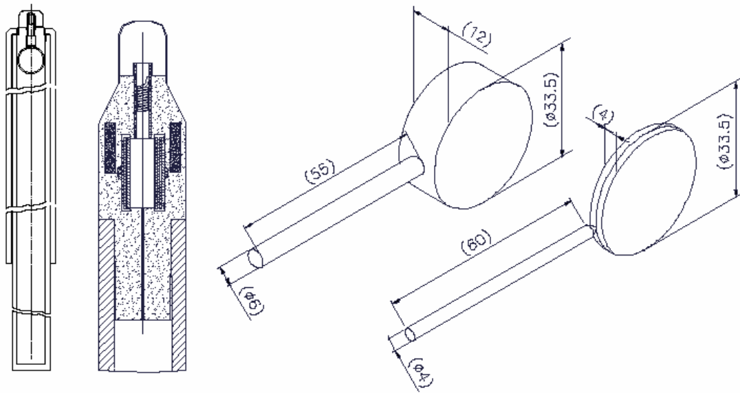
Figura 2.5 - Sonda para extração de metal e esquema da geometria da amostra extraída para análise via espectroscopia (dimensões em mm) [12].
