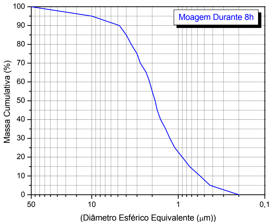
Figura 4.8 - Curva de distribuição granulométrica do pó de La-β-alumina calcinado a 1550 °C submetidas a ciclo de moagem de 8 horas.
