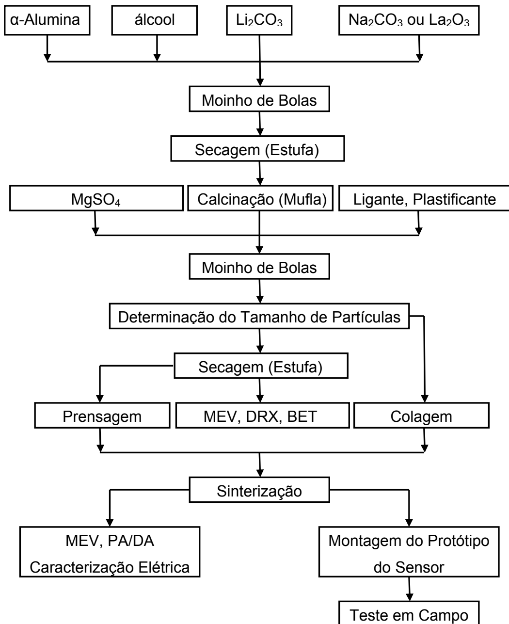
Figura 3.1 - Principais etapas envolvidas no desenvolvimento de sensores de \beta -alumina.
