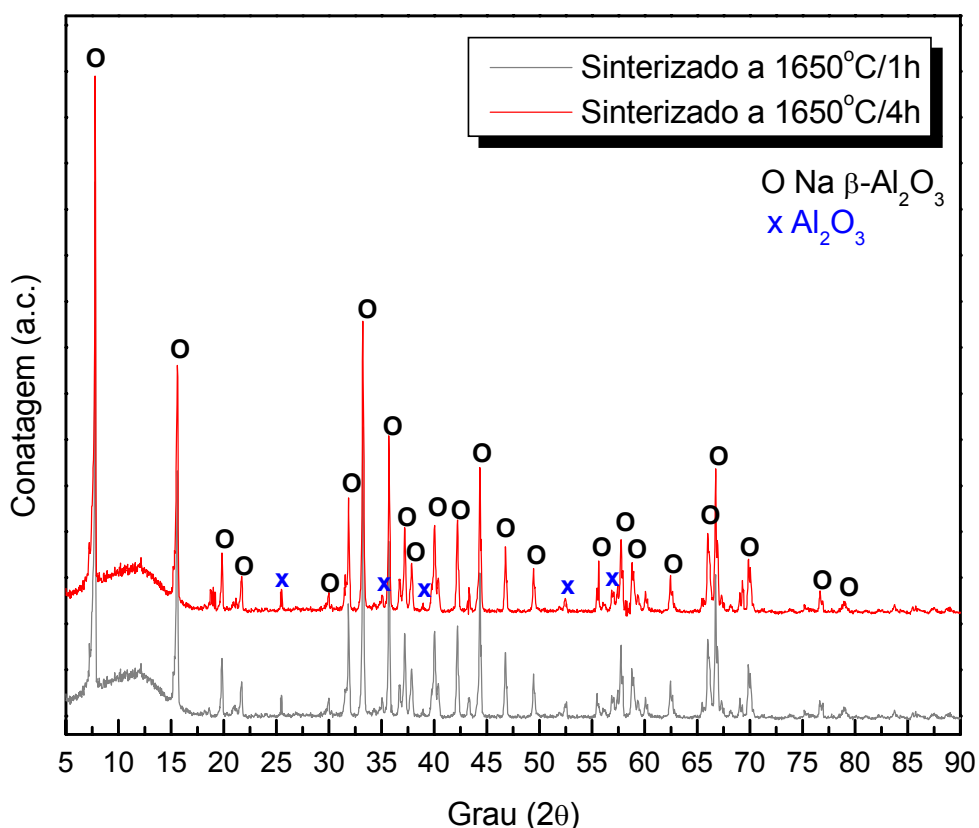
Figura 4.15 - Difração de raios X das amostras de Na-β-alumina após sinterização à condição de 1650°C com períodos de 1 hora e 4 horas.
