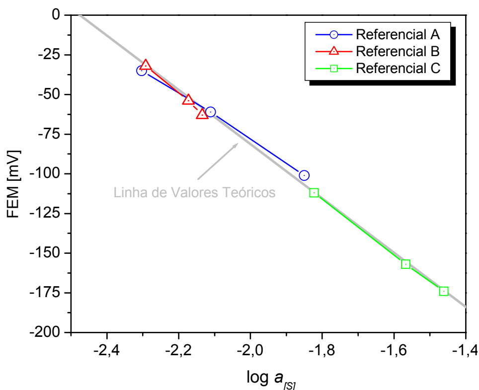
Figura 4.33 - Correlação entre a FEM gerada pelo sensor La- \beta -alumina com relação ao logaritmo da atividade do enxofre ( a_{S} ).
