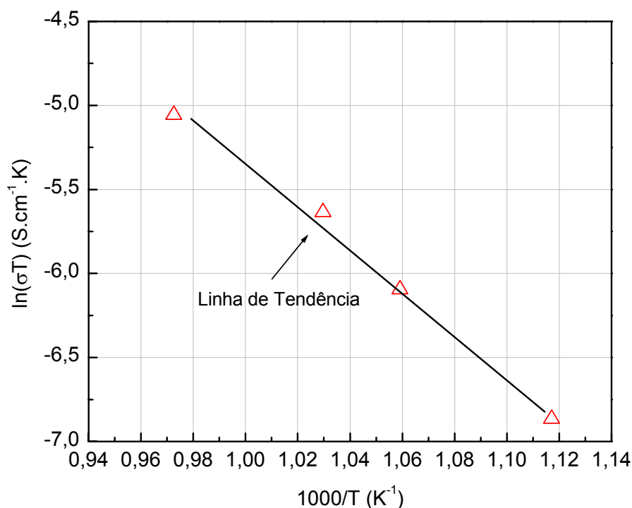
Figura A.9 - Gráfico de Arrhenius para a condutividade do La-β-alumina em função do inverso da temperatura.
