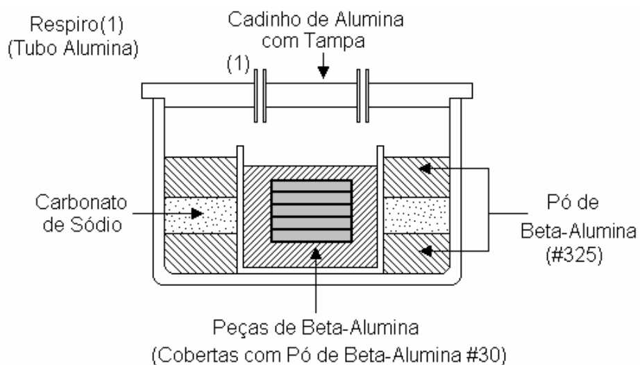
Figura 4.14 - Esquema ilustrando o sistema para sinterização de amostras preparadas a partir da compactação de Na- \beta -alumina.
