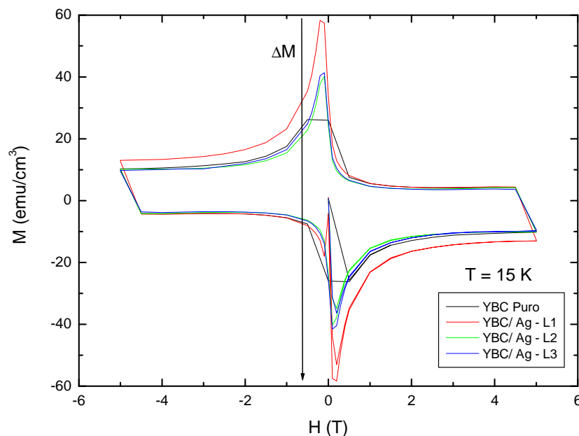
Figura 4.17 – Ciclos de histerese para as amostras de \text{YBa}_2\text{Cu}_3\text{O}_{7-\delta} e \text{YBa}_2\text{Cu}_3\text{O}_{7-\delta}/\text{Ag} . Em destaque, região de \Delta M
