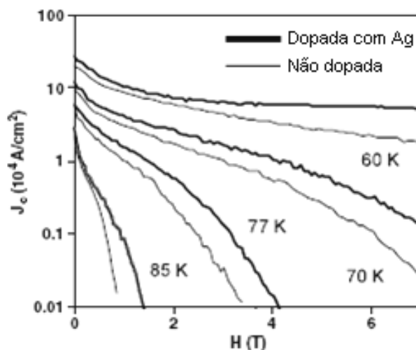
Figura 2.7 – Variação de J_c em função do campo magnético aplicado para amostras de \text{YBa}_2\text{Cu}_3\text{O}_{7-\delta} e \text{YBa}_2\text{Cu}_3\text{O}_{7-\delta}/\text{Ag} [57]- Figura adaptada.
