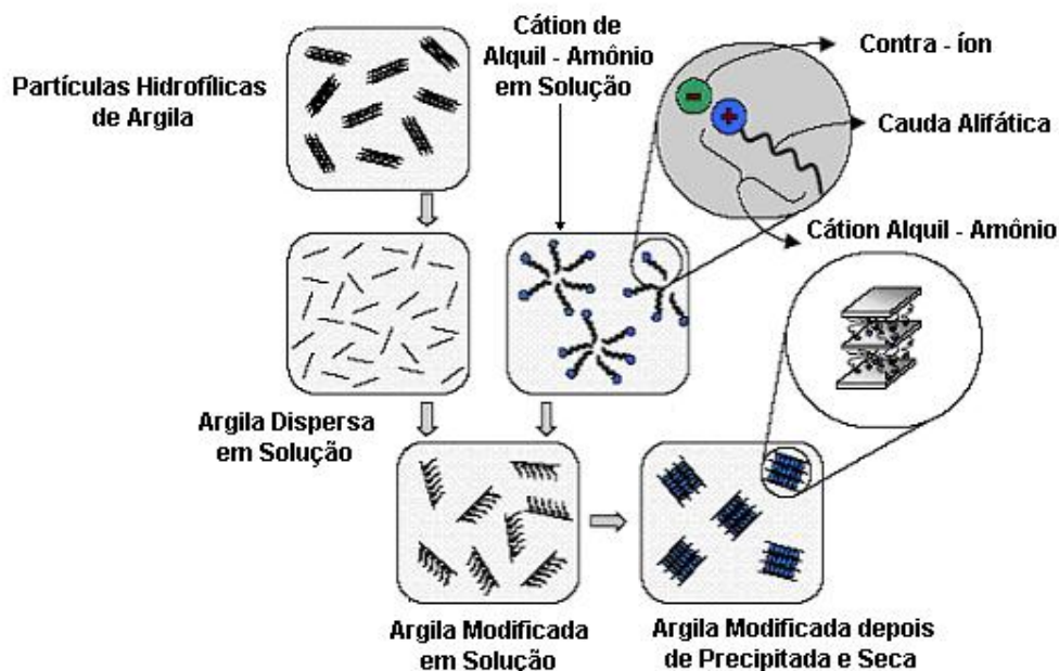
Figura 2.6 Representação esquemática do tratamento superficial da argila [19].
