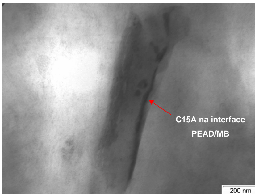
Figura 4.39 Micrografia de MET do grânulo do nanocompósito de PEAD/EVA 8/C15A (80/15/5), com aumento de 66000x.
