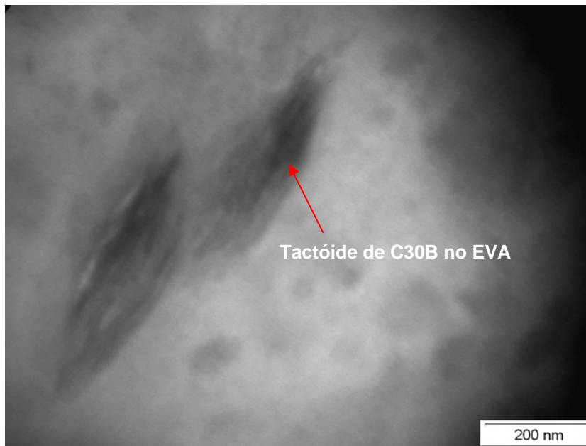
Figura 4.45 Micrografia de MET do grânulo do nanocompósito de PEAD/EVA 25/C30B (80/15/5), com aumento de 88000x.
