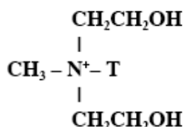
Figura 3.2 Estrutura química do modificador orgânico da Cloisite ® 30B [83].
