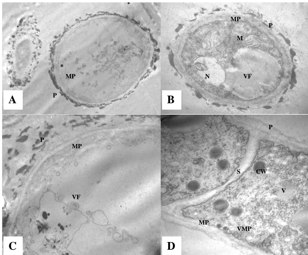
Figura 15. Fotomicrografia por microscopia eletrônica de transmissão de Aspergillus ochraceus irradiado com 2,0 kGy, isolado por diluição seriada do milho. Aumentos: A (x 5800); B (x 20700); C (x 13100); D (x 34600). CW: corpos Woronin; N: núcleo; M: mitocôndria; MP: membrana plasmática; P: parede celular; S: septo; V: vacúolo; VF: fusão de vacúolo; VMP: vesícula.
