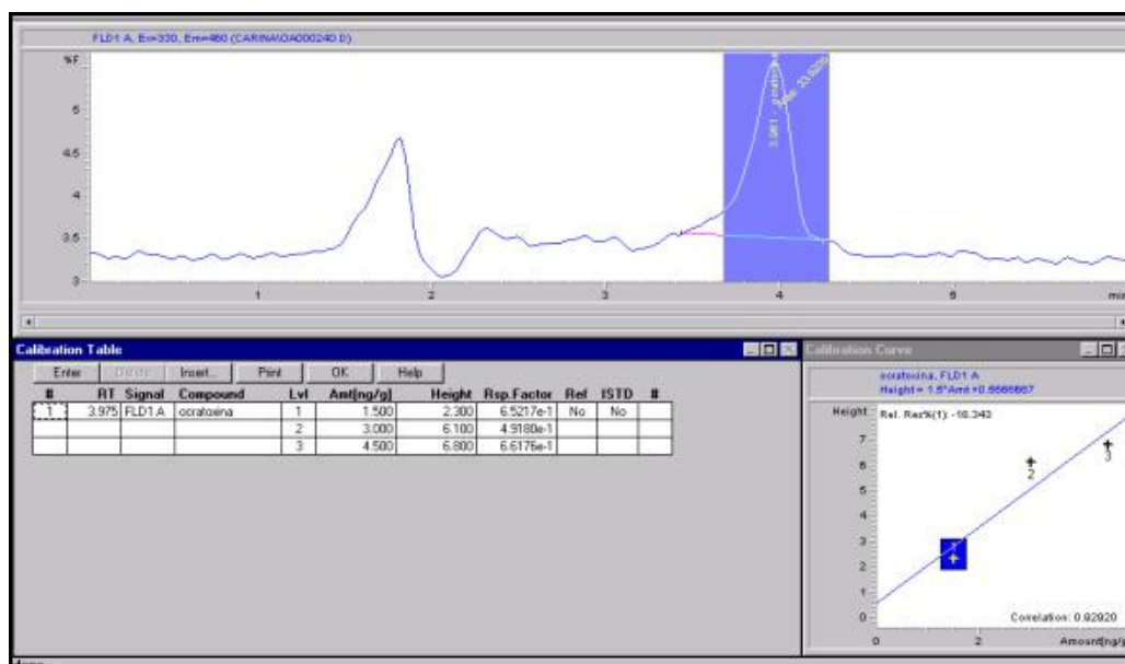
Figura 7. Cromatograma de uma solução padrão de ocratoxina A de 3 ng ml -1 .
