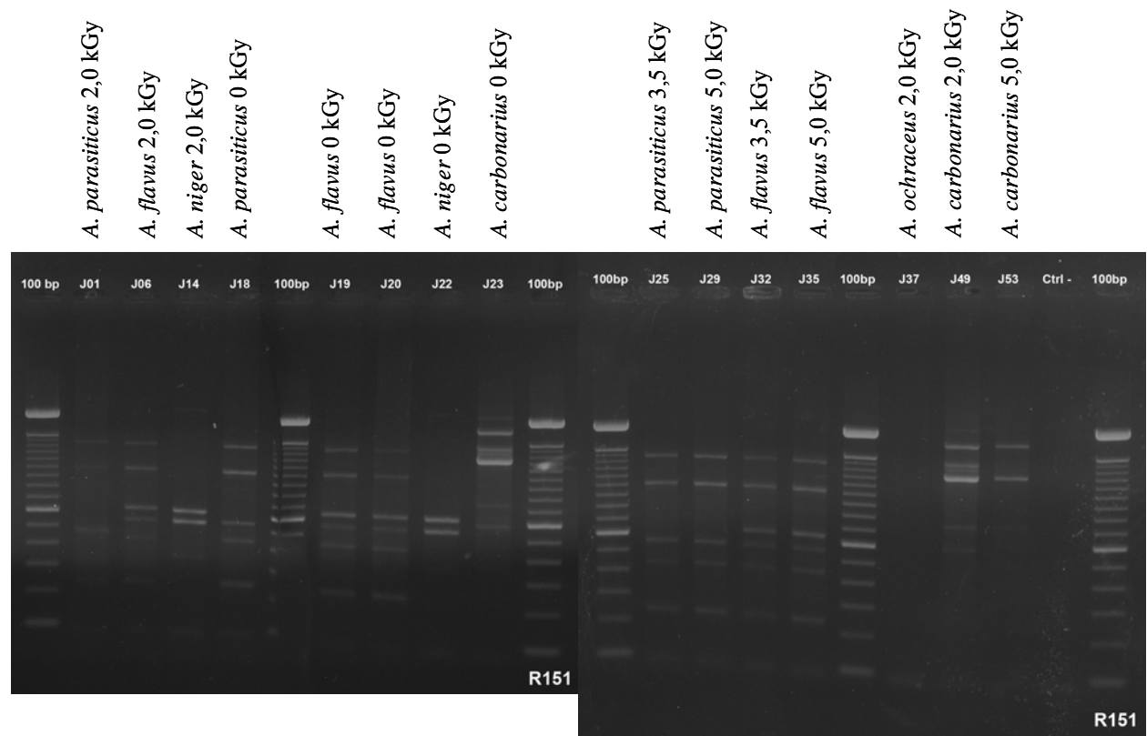
Figura 17. Produtos de amplificação por RAPD obtidos a partir de espécies de Aspergillus spp. É mostrada a amplificação com o primer R 151.
