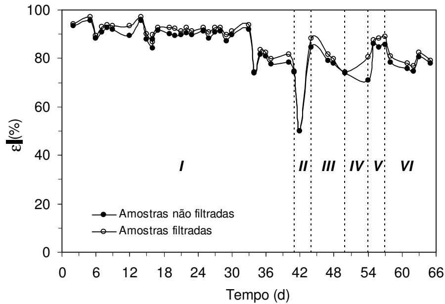
Figura 5.22 – Eficiência de remoção de matéria orgânica na operação com 4000 mgDQO/L ( I, III, e VI : 4000 mgDQO/L; II e V : 2000 mgDQO/L; IV : 1000 mgDQO/L)
