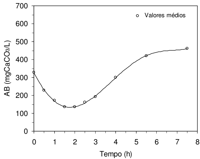
Figura 5.35 – Perfil de alcalinidade a bicarbonato (AB) na operação com 3000 mgDQO/L: AR-IPHP-II – Alimentação em batelada
