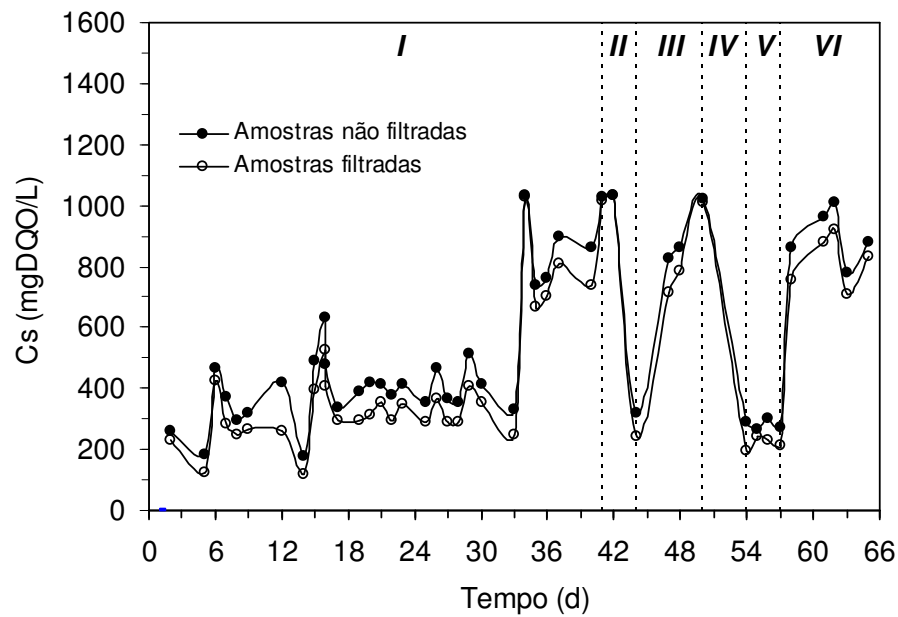
Figura 5.21 – Concentração de matéria orgânica na operação com 4000 mgDQO/L (I, III, e VI: 4000 mgDQO/L; II e V: 2000 mgDQO/L; IV: 1000 mgDQO/L)
