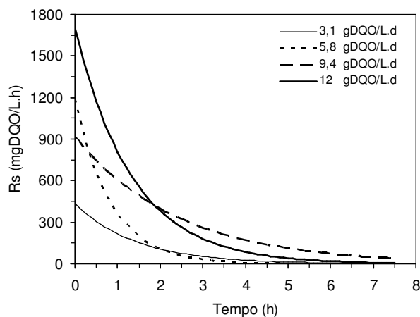
Figura 5.72 – Perfis de velocidade de reação nas operações com 3,1 a 12,0 gDQO/L.d e alimentação em batelada – Modelo III
