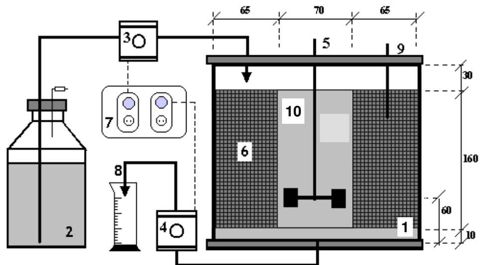
Figura 4.1 – Esquema do reator anaeróbico operado em bateladas seqüenciais contendo biomassa imobilizada (Dimensões em milímetros): (1) Tanque de reação, (2) Água residuária, (3) Bomba de alimentação, (4) Bomba de descarga, (5) Agitador mecânico, (6) Cesto contendo espumas com células imobilizadas, (7) Temporizadores, (8) Efluente tratado, (9) Termômetro, (10) “Draft tube”
