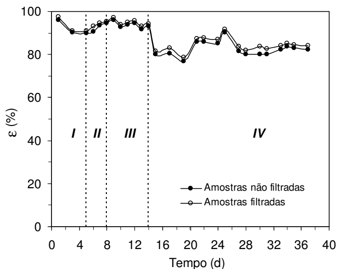
Figura 5.65 – Eficiência de remoção de matéria orgânica na operação com 3000 mgDQO/L ( C_A = 6000 mgDQO/L): AR-IPHP-I – Alimentação em batelada alimentada I : 3000 mgDQO/L - C_A = 6000 mgDQO/L; II : 1000 mgDQO/L - C_A = 2000 mgDQO/L; III : 2000 mgDQO/L - C_A = 4000 mgDQO/L; IV : 3000 mgDQO/L - C_A = 6000 mgDQO/L)
