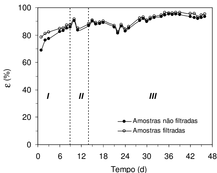
Figura 5.62 – Eficiência de remoção de matéria orgânica na operação com 3000 mgDQO/L:
