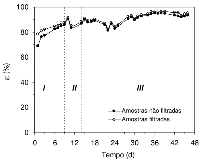
Figura 5.31 – Eficiência de remoção de matéria orgânica na operação com 3000 mgDQO/L:
