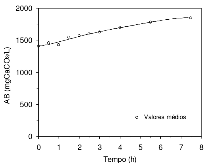
Figura 5.26 – Perfil de alcalinidade a bicarbonato (AB) na operação com 4000 mgDQO/L
