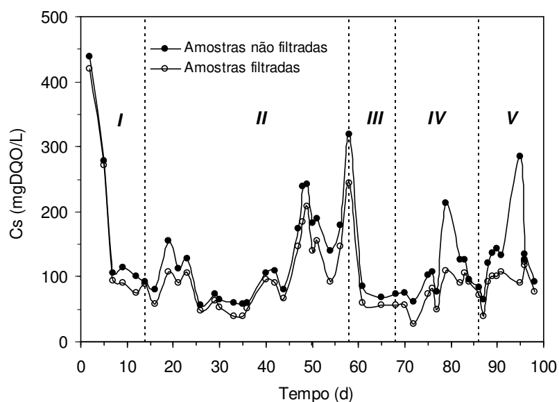
Figura 5.3 – Concentração de matéria orgânica na operação com 1000 mgDQO/L (I e IV: AR-IPHP-II e extrato de carne (fonte N); II e V: AR-IPHP-II e uréia (fonte N); III: AR-S)
