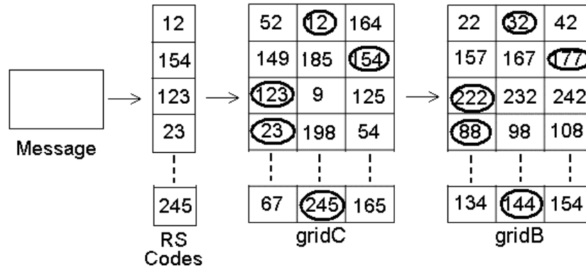
Figura 12 – Fuzzy Vault proposto por Nagar e Chaudhury (2006).
