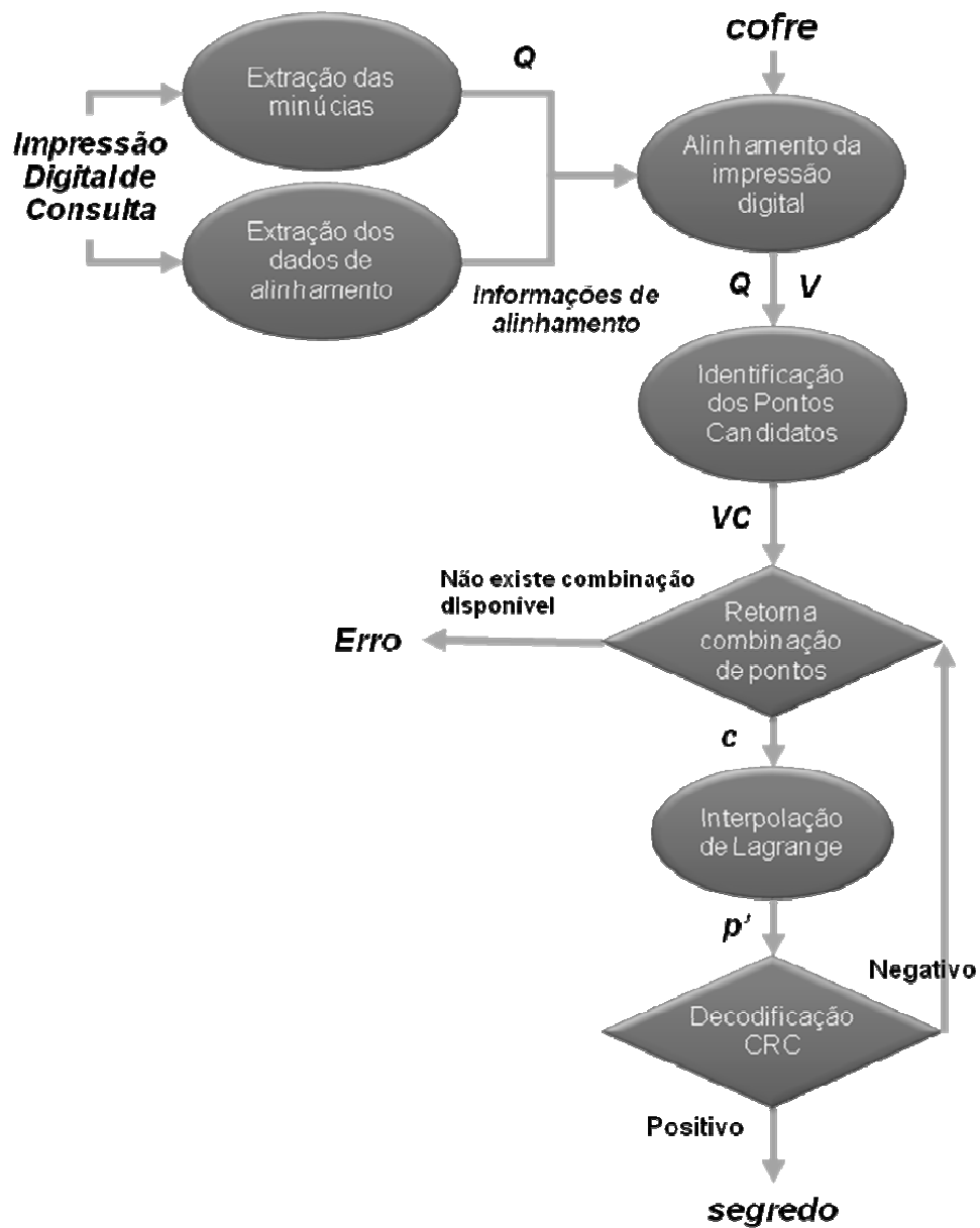
Figura 14 - Diagrama do processo de descriptação da implementação proposta
