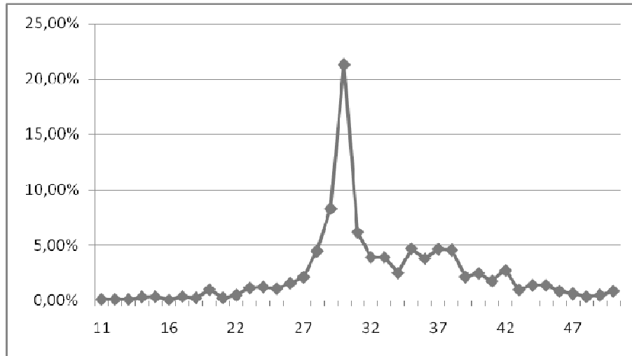
Figura 24 – Distribuição das encriptações em função da quantidade de minúcias da impressão digital modelo.
