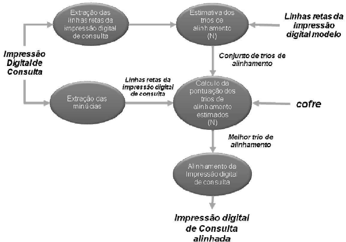
Figura 21 – Passos do algoritmo de alinhamento da impressão digital de consulta.
