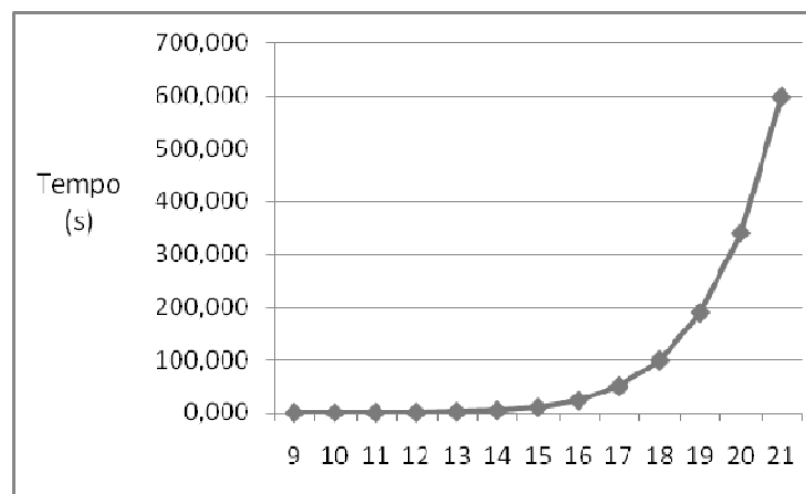
Figura 28 – Tempo de descriptação em função da quantidade de pontos candidatos (descriptações erradas).
