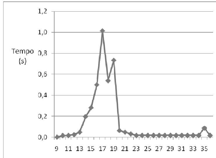
Figura 27 – Tempo descriptação em função da quantidade pontos candidatos (descriptações corretas).
