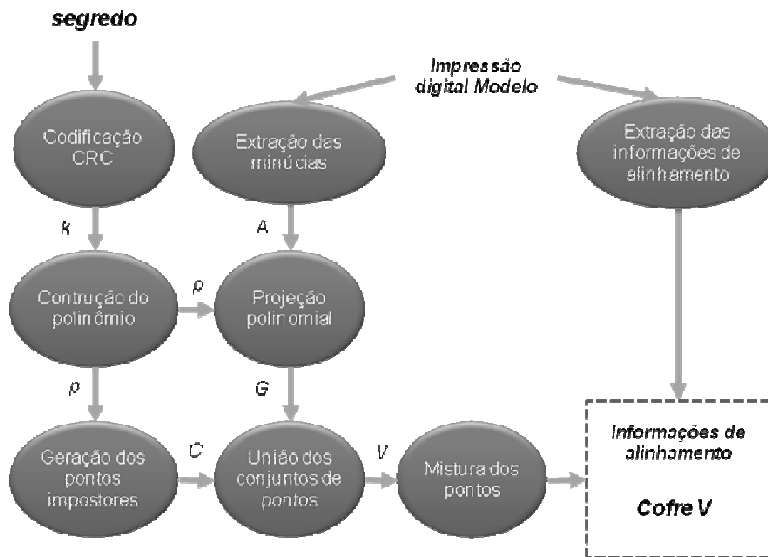
Figura 13 - Diagrama do processo de encriptação da implementação proposta.
