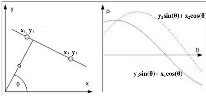
Figura 16: Mapeamento de pontos de uma reta do domínio espacial para o domínio da transformada de Hough (MARANA e JAIN, 2005).
