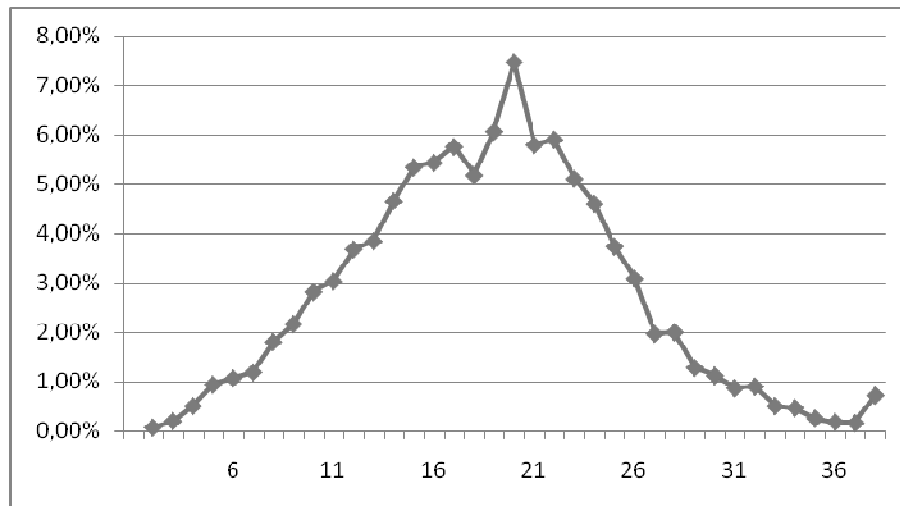
Figura 26 – Distribuição das descriptações em função da quantidade de pontos candidatos.
