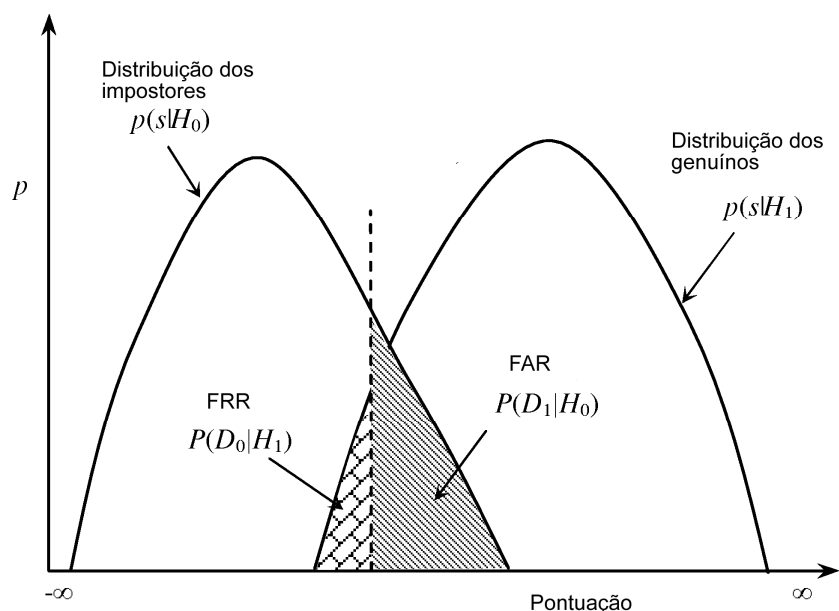
Figura 5 – Distribuição das probabilidades de erros nos sistemas biométricos (JAIN, ROSS e PRABHAKAR, 2001)
