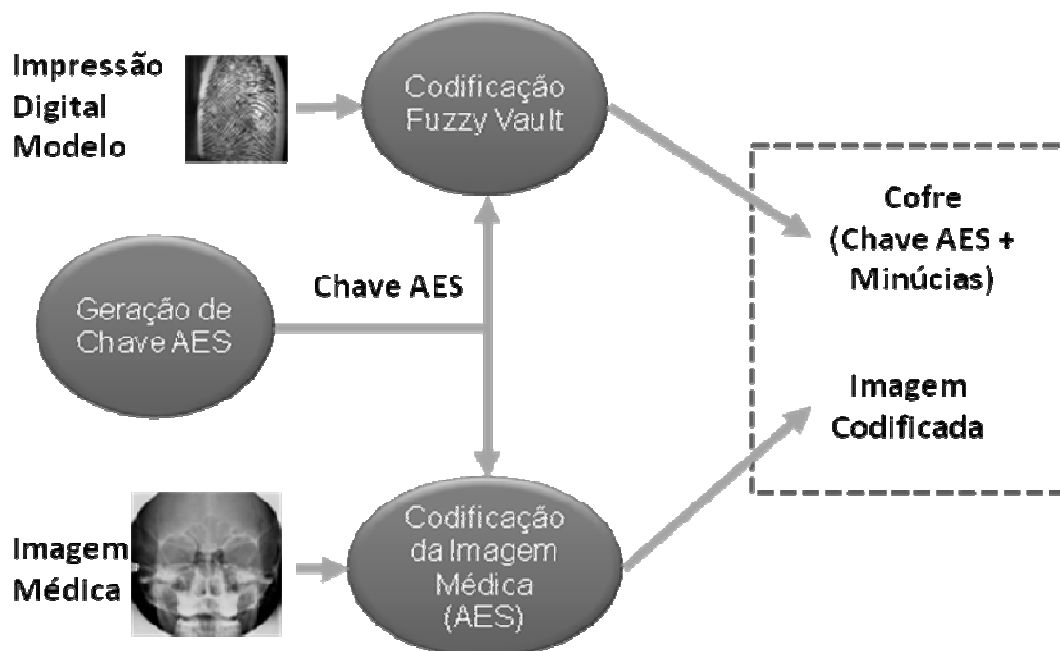
Figura 29 - Algoritmo de encriptação do cenário de proteção de imagens médicas usando biometria.
