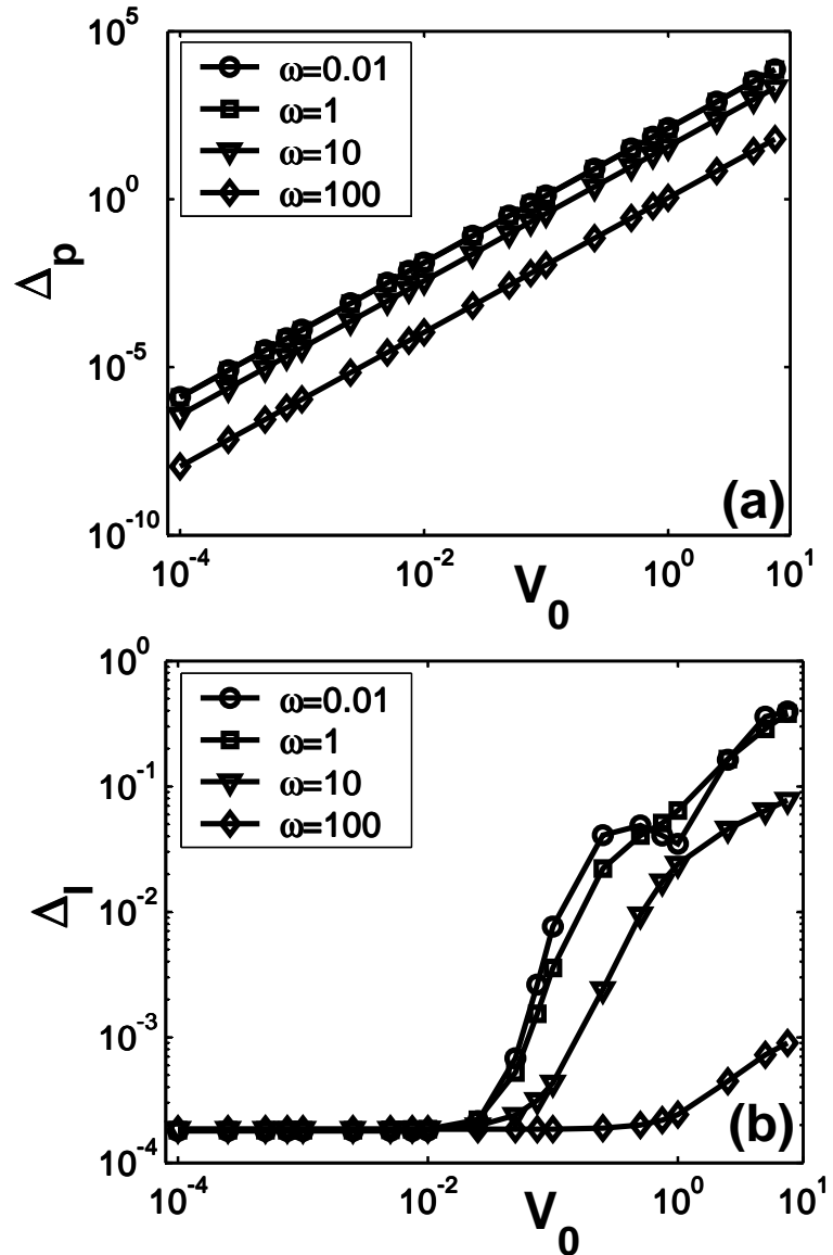
Figura 5.7: a) Quantificador para o desvio no número de íons \Delta_p (veja a Eq. (5.16)) versus a amplitude V_0 da voltagem aplicada, para diferentes valores da frequência; b) Quantificador para a diferença na corrente \Delta_I (veja a Eq. (5.17)) versus a amplitude V_0 da voltagem aplicada, também para diferentes valores da frequência.
