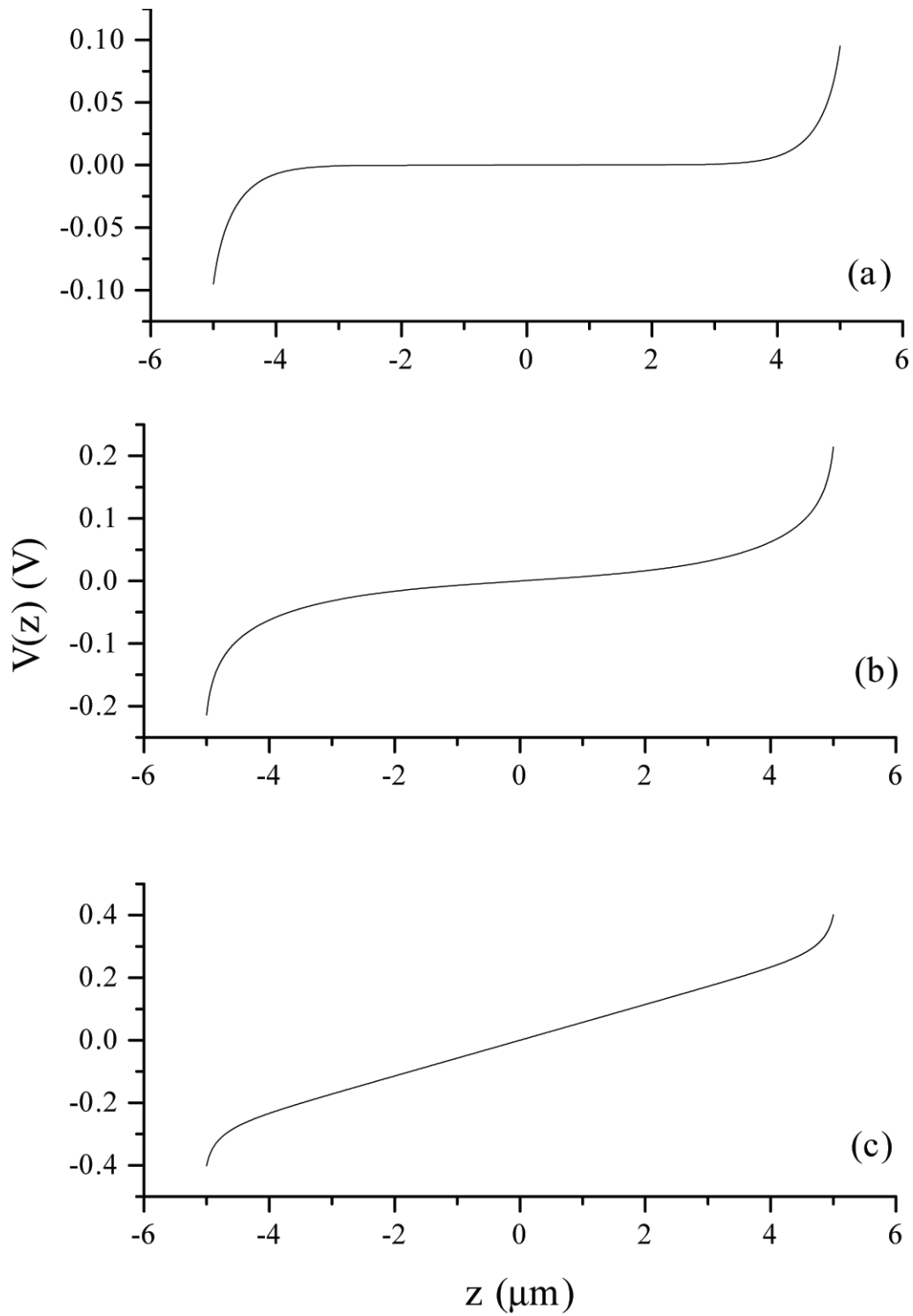
Figura 2.5: Voltagem V(z) versus z para d = 10\mu\text{m} e \lambda = 0.36\mu\text{m} . Para U pequeno, E se anula para z = 0 . (a) U = 0.2\text{ V} , (b) U = 0.4\text{ V} , e (c) U = 0.8\text{ V} .
