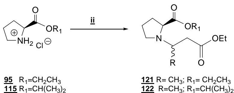
Esquema 3.4: Adição de Michael. Condições: crotonoato de etila, DIPEA, \text{CH}_3\text{CN} , 0^\circ\text{C} - 65^\circ\text{C} , 42 horas.
