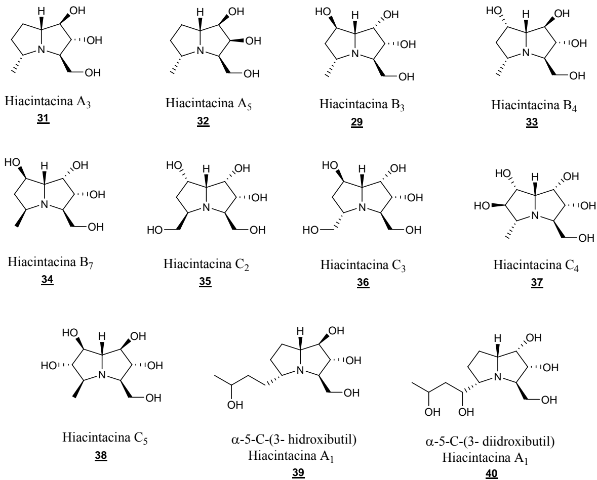
Figura 1.8: Alcalóides isolados da Scilla socialis .
