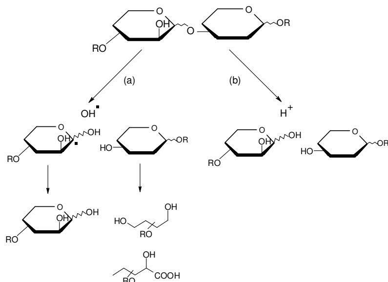
Figura 2. Mecanismo de reação da despolimerização via radical (a) e hidrólise ácida (b).
