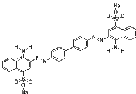
Figura 4 - Estrutura química do corante Vermelho Congo (ácido sulfônico-1-naftaleno-3,3-(4,4-bifenil-bis(azo))-bis(4-amino-di-sódio)).
