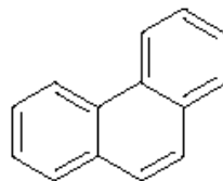
Figura 5 - Estrutura química do composto aromático fenantreno.
