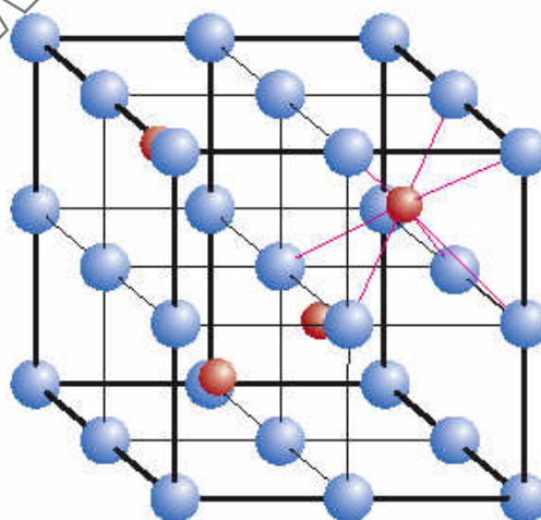
FIGURA 1.1: Estrutura da céria, onde as esferas vermelhas representam os sítios de cátions de cério e as esferas azuis os sítios de ânions de oxigênio 2 .
