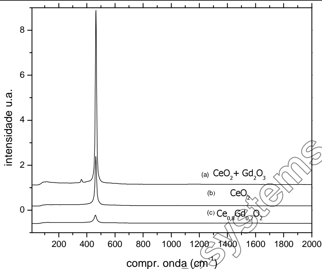
FIGURA 4.4: Espectro de RAMAN de (a) \text{CeO}_2 (Aldrich) misturada com \text{Gd}_2\text{O}_3 (Aldrich) a temperatura ambiente, e das fases (b) \text{CeO}_2 e (c) \text{Ce}_{0,8}\text{Gd}_{0,2}\text{O}_2 obtidas por coprecipitação neste trabalho a temperatura ambiente.
