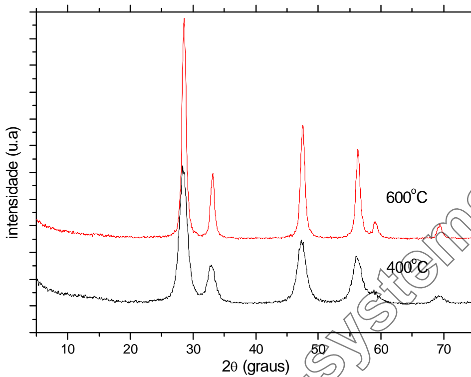
FIGURA 4.14: Difractogramas das amostras com 15% de Gd sintetizadas pelo método dos precursores poliméricos.
