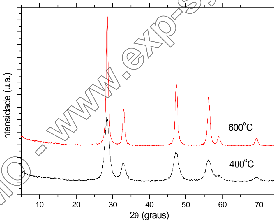
FIGURA 4.13: Difractogramas das amostras com 10% de Gd sintetizadas pelo método dos precursores poliméricos.
