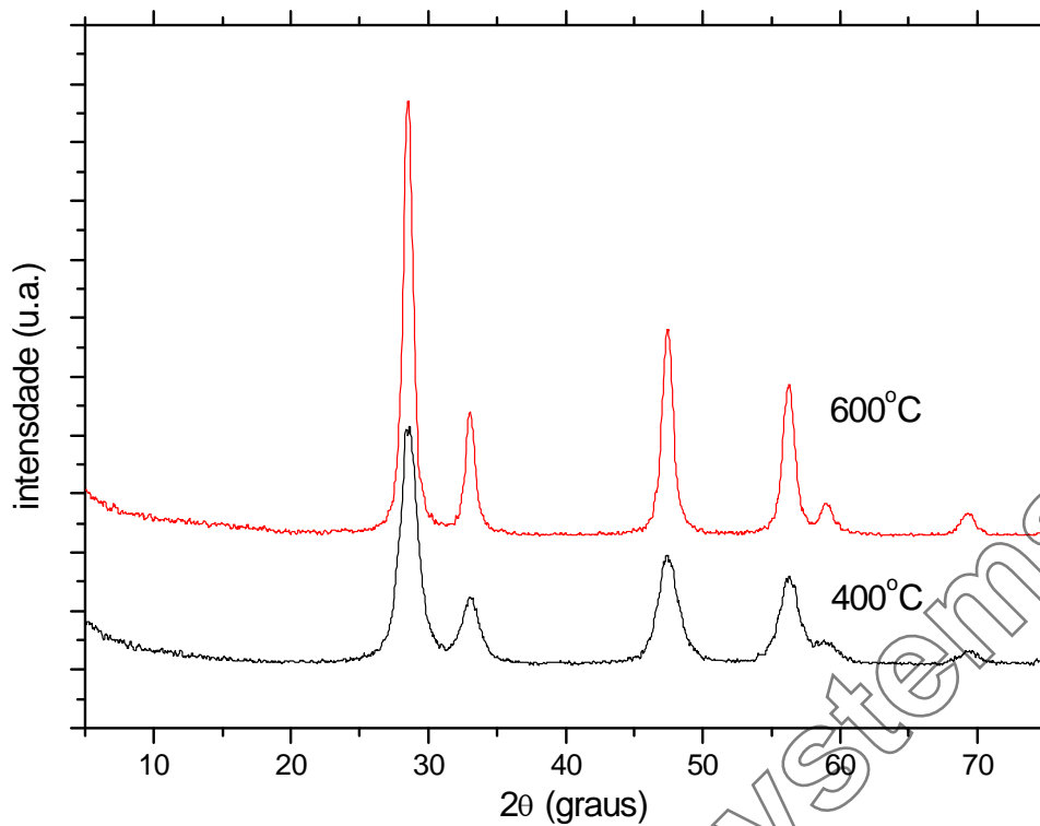
FIGURA 4.15: Difratomogramas das amostras com 20% de Gd sintetizadas pelo método dos precursores poliméricos
