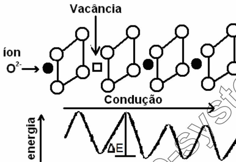
FIGURA 1.4: Variação da energia potencial iônica ao longo do caminho de difusão.
