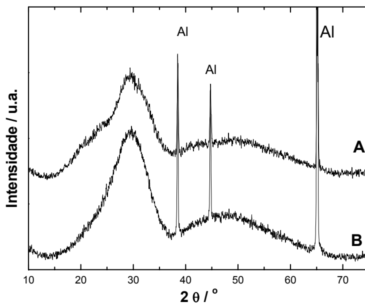
Figura 3.52: Difratograma de raios X das amostras obtidas via síntese não aquosa.
