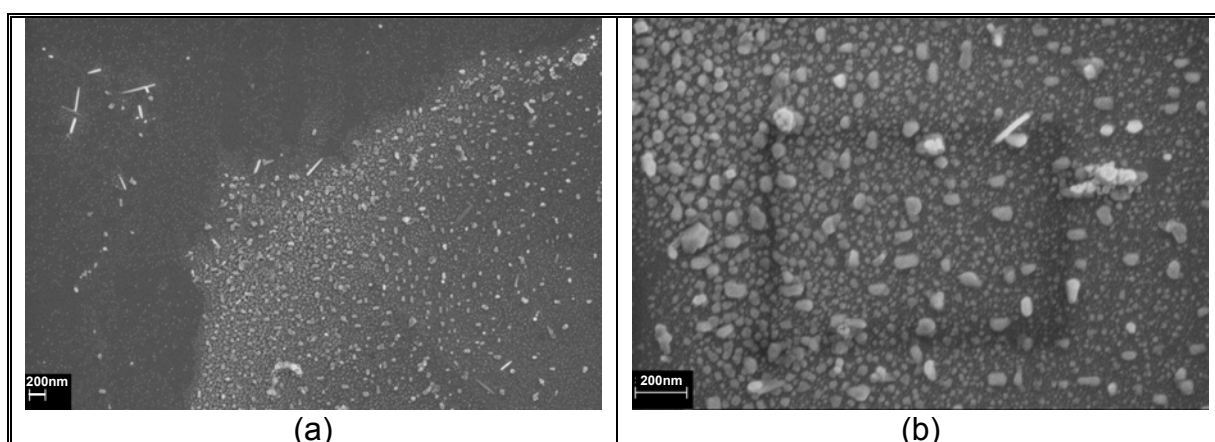
Figura 3.25: Imagens de MEV da amostras obtidas em substratos de STO imersos em R_a durante 15 minutos, (a) com aumento de 50000 vezes; (b) com aumento de 160000 vezes.
