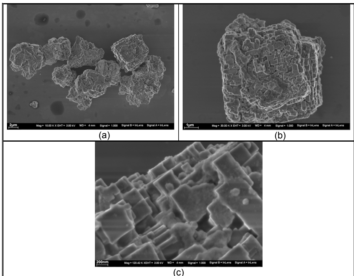
Figura 3.41: Imagens de MEV da amostra AA com aumentos de (a) de 10000 vezes; (b) de 30000 vezes e (c) de 120000 vezes.
