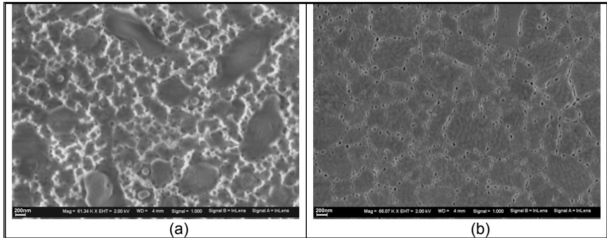
Figura 3.26: Imagens de MEV das amostras obtidas com R7 em substrato de MgO (a) por 15 min com aumento de 60000 vezes; (b) por 30 min com aumento de 66000 vezes.
