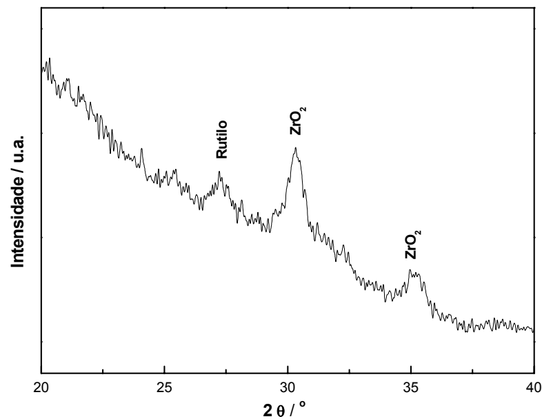
Figura 3.3: Difratograma de raios X do filme de uma camada sintetizado com R b e tratado termicamente em 700°C por 4 horas.
