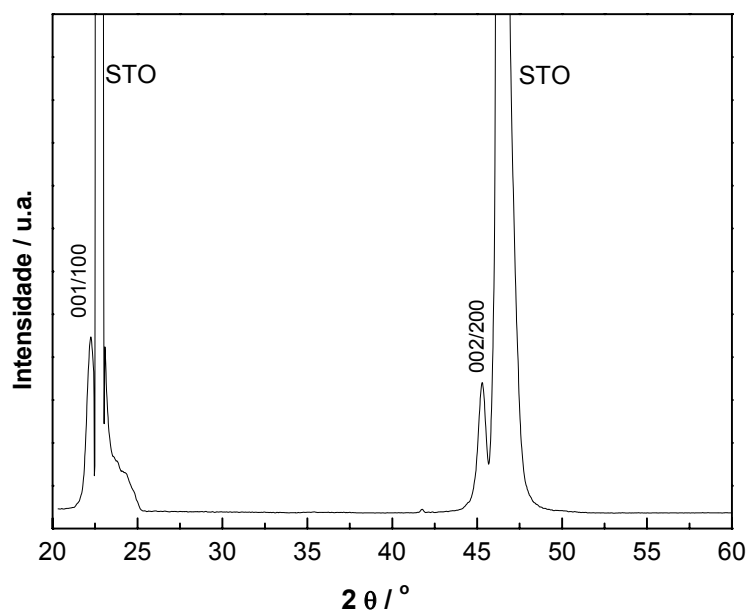
Figura 3.61: Difratograma de raios X de um filme de BTO de uma camada em substrato de STO tratado em 700°C.
