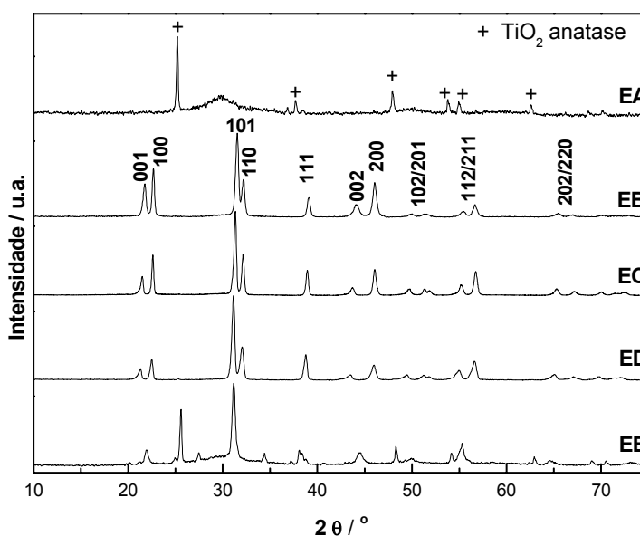
Figura 3.33: Difratomogramas de raios X dos pós EA, EB, EC, ED e EE obtidos via síntese hidrotermal.
