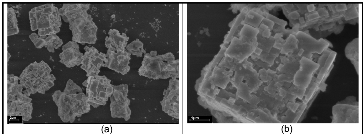
Figura 3.42: Imagens de MEV da amostra BB com aumentos de (a) de 100000 vezes e (b) de 40000 vezes.
