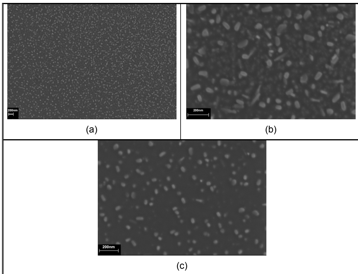
Figura 3.14: Imagens de MEV da amostras obtidas em substratos limpos com sulfocrômica por imersão de R_a durante 15 minutos (a) com aumento de 52000 vezes; (b) com aumento de 221000 vezes; (c) com aumento de 101000 vezes.
