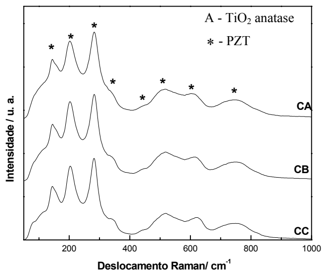
Figura 3.37: Espectros Raman dos pós CC, CB e CA obtidos via síntese hidrotermal.
