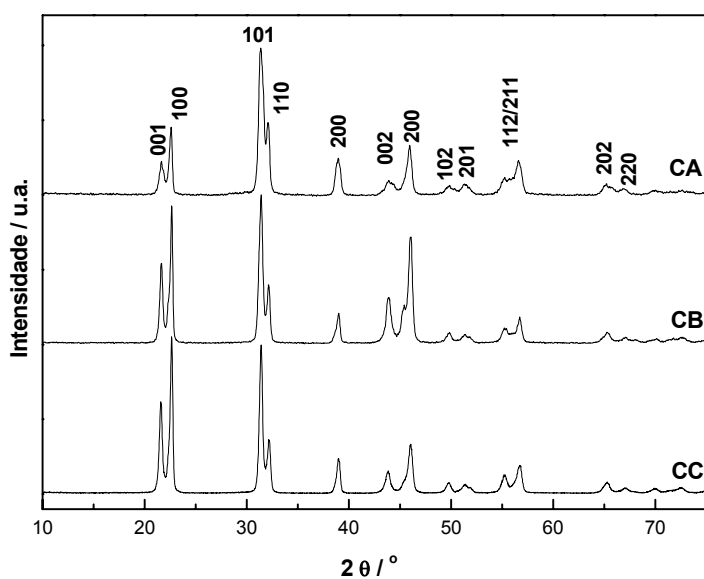
Figura 3.31: Difratogramas de raios X dos pós CC, CB e CA obtidos via síntese hidrotermal.
