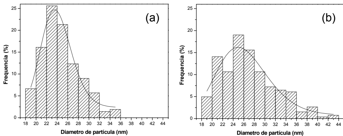
Figura 3.21: Distribuição do tamanho de partículas das amostras obtidas em substratos hidrofílicos imersos em R_a durante (a) 15 minutos e (b) 30 minutos.
