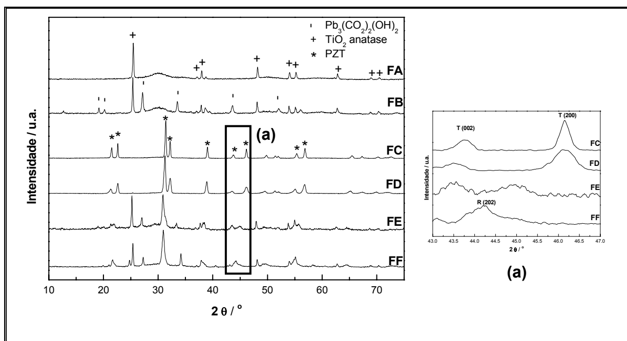
Figura 3.34: Difratogramas de raios X dos pós FA, FB, FC, FD, FE e FF obtidos via síntese hidrotermal.
