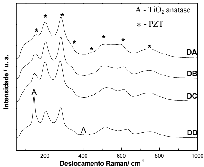
Figura3.38: Espectros Raman dos pós DD, DC, DB e DA obtidos via síntese hidrotermal.
