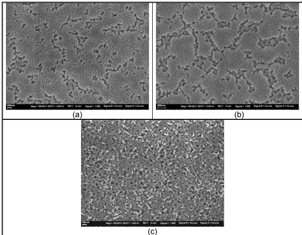
Figura 3.57: Imagens de MEV com aumento de 100000 vezes das amostras de BTO obtidas com as viscosidades (a) 16mPa.s; (b) 11mPa.s e (c) 7mPa.s.
