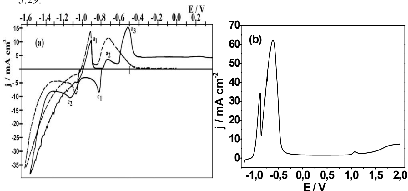
FIGURA 5.29: Curvas voltamétricas: (a) do eletrodo de platina em 0,05M Pb(NO 3 ) 2 + 0,05M SnCl 2 + 0,1M NaKC 4 H 4 O 6 e 0,4M NaOH (—) e 0,05M SnCl 2 + 0,1M NaKC 4 H 4 O 6 e 0,4M NaOH (----), (b) do eletrodo de Sn em 0,1M NaKC 4 H 4 O 6 e 0,4M NaOH, v = 10\text{mV s}^{-1} .
