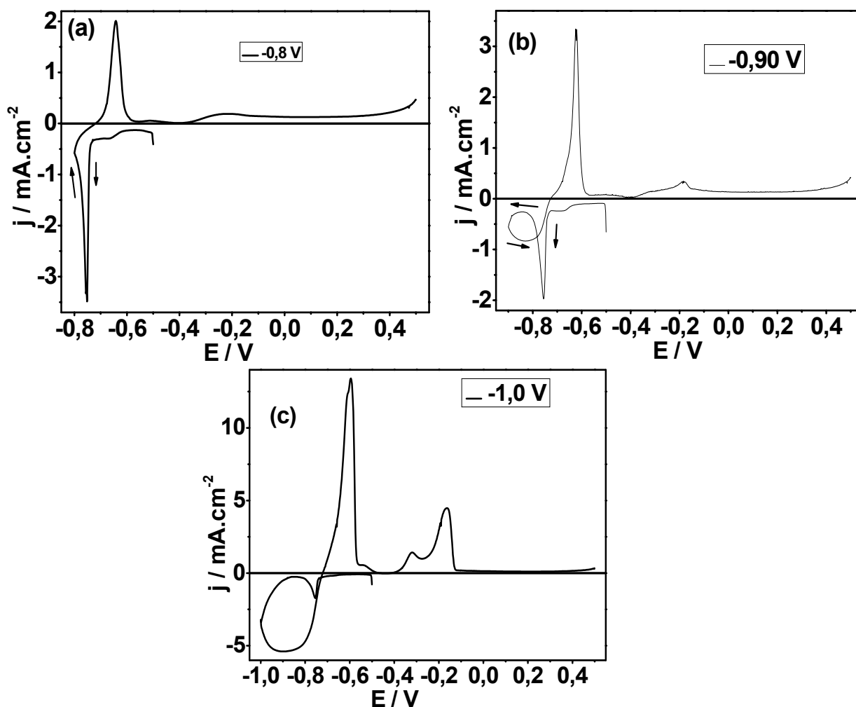
FIGURA 5.48: Curvas voltamétricas do eletrodo de platina em 0,1\text{M Pb}(\text{NO}_3)_2 + 0,1\text{M CuSO}_4 + 0,2\text{M sorbitol} + 3,0\text{M NaOH} ; efeito do potencial limite: (a) -0,80 V, (b) -0,90 V e (c) -1,0 V, v = 10\text{mV s}^{-1} .
