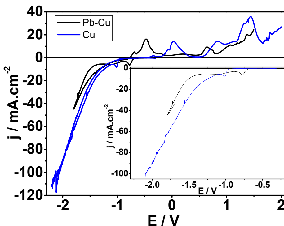
FIGURA 5.62: Curva voltamétrica do eletrodo de platina em 0,05\text{M Pb}(\text{NO}_3)_2 + 0,05\text{M CuSO}_4 + 0,1\text{M EDTA} + 0,4\text{M NaOH} (linha preta) e 0,05\text{M CuSO}_4 + 0,1\text{M EDTA} + 0,4\text{M NaOH} (linha azul), v = 10\text{mV}\cdot\text{s}^{-1} .
