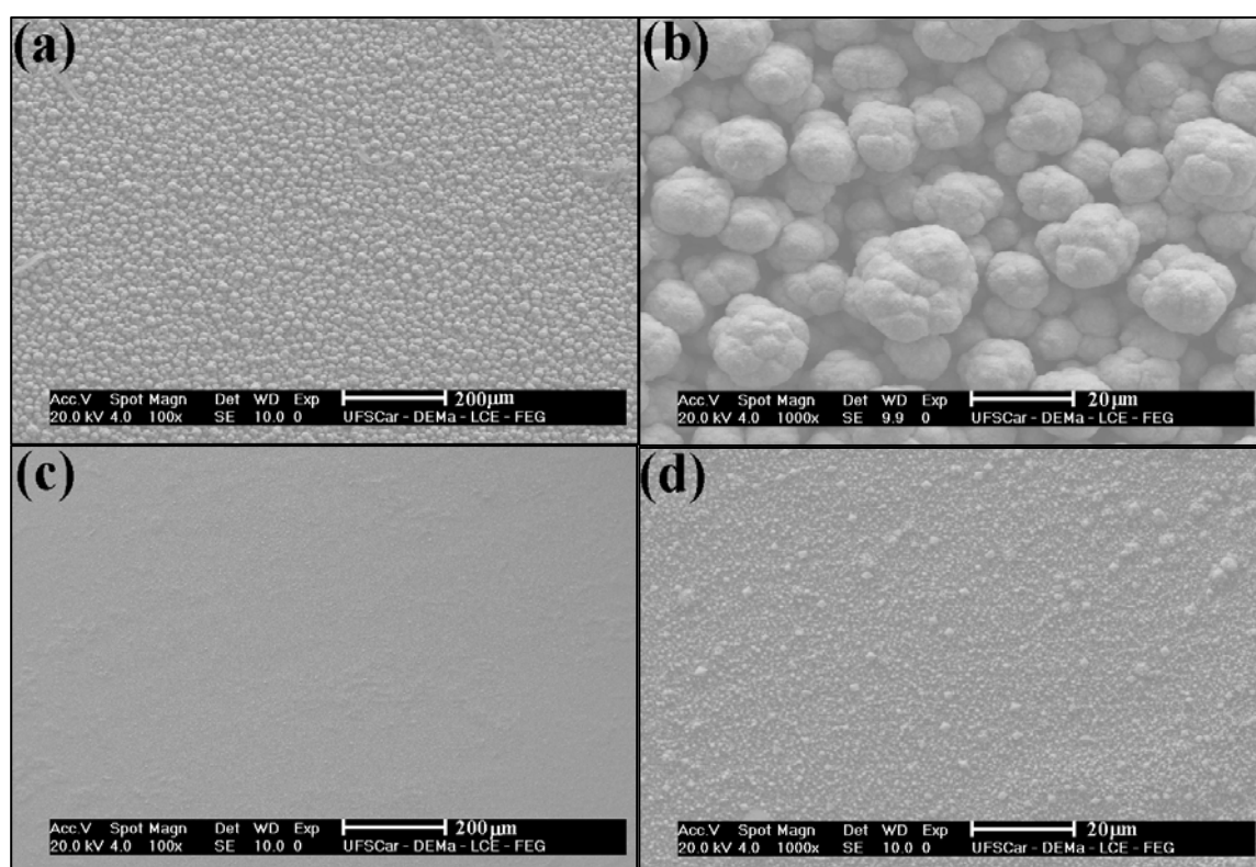
FIGURA 5.59 – MEV dos filmes de Pb-Cu, obtidos potenciostaticamente de -0,300\text{ V} para -0,780\text{ V} , q_d = 5\text{ C.cm}^{-2} (a) 100X e (b) 1000X; de -0,300\text{ V} para -1,0\text{ V} , q_d = 5\text{ C.cm}^{-2} (c) 100X e (d) 1000X. Solução de deposição: 0,05\text{M Pb(NO}_3)_2 + 0,05\text{M CuSO}_4 + 0,1\text{M NaKC}_4\text{H}_4\text{O}_6 e 0,4\text{M NaOH} .
