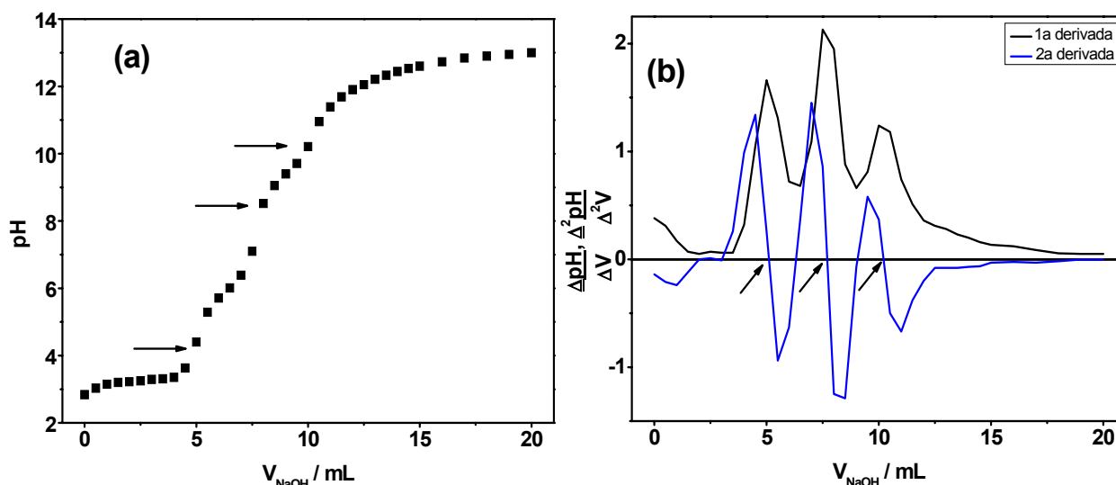
FIGURA 5.14: (a) Curva de pH para a titulação potenciométrica da solução de 0,05M \text{CuSO}_4 + 0,1M de EDTA com solução de NaOH 0,9706M, (b) Curvas da 1ª e 2ª derivadas.
