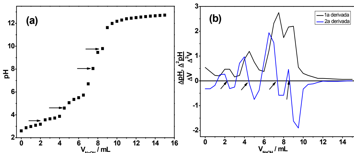
FIGURA 5.4: (a) Curva de pH para a titulação potenciométrica da solução de 0,05\text{M Pb}(\text{NO}_3)_2 + 0,05\text{M SnCl}_2 com solução de \text{NaOH } 0,9706\text{M} , (b) Curvas da 1ª e 2ª derivadas.
