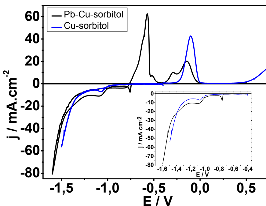
FIGURA 5.46: Curvas voltamétricas do eletrodo de platina em 0,1M Pb(NO_3)_2 + 0,1M CuSO_4 + 0,2M sorbitol e 3,0M NaOH (—) e 0,1M CuSO_4 + 0,2M sorbitol e 3,0M NaOH (—), v = 10\text{mV s}^{-1} .
