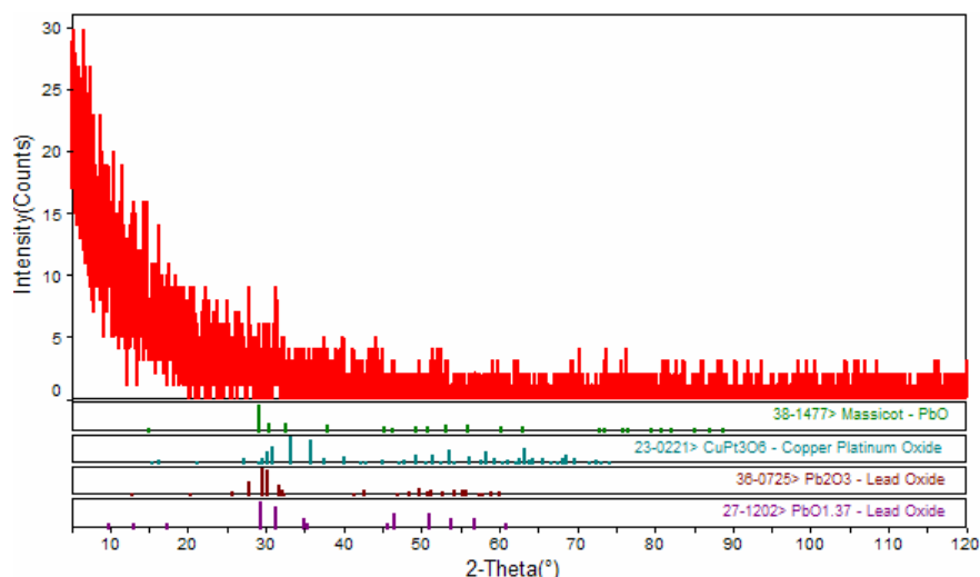
FIGURA 5.50 – Difratoograma de raios X dos depósitos obtidos potenciostaticamente de -0,400 V para -0,760 V com densidade de carga de 5,0\text{C cm}^{-2} . Solução de deposição: 0,1\text{M Pb}(\text{NO}_3)_2 + 0,1\text{M CuSO}_4 + 0,2\text{M sorbitol} e 3,0\text{M NaOH} .
