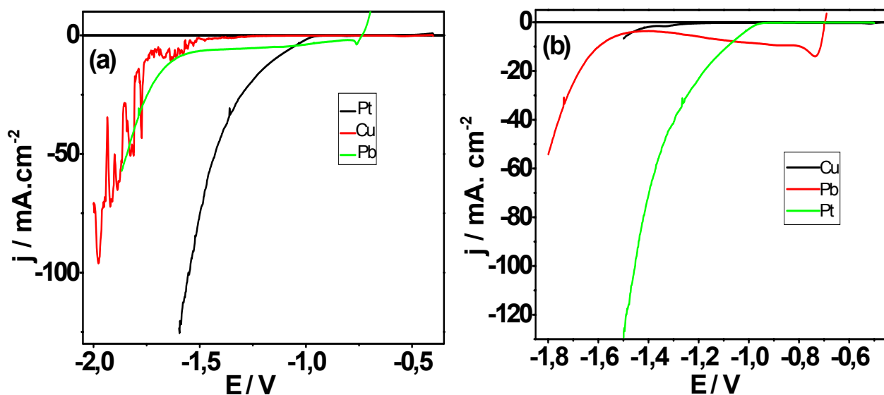
FIGURA 5.47: Curvas voltamétricas: (a) dos eletrodos de Pt, Pb, Cu, em 0,2 M sorbitol e 3,0M NaOH e (b) dos eletrodos de Pb, Pt, Sn em 3,0M NaOH, v = 10\text{mV s}^{-1} .
