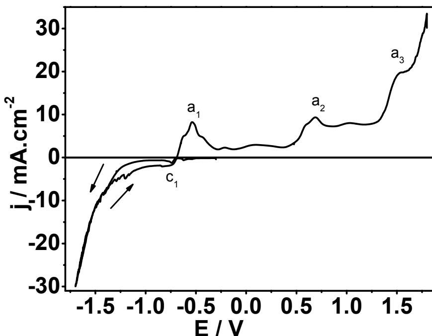
FIGURA 5.53: Curva voltamétrica do eletrodo de platina em 0,05\text{M Pb}(\text{NO}_3)_2 + 0,05\text{M CuSO}_4 + 0,1\text{M NaKC}_4\text{H}_4\text{O}_6 e 0,4\text{M NaOH} , v = 10\text{mV}\cdot\text{s}^{-1} .
