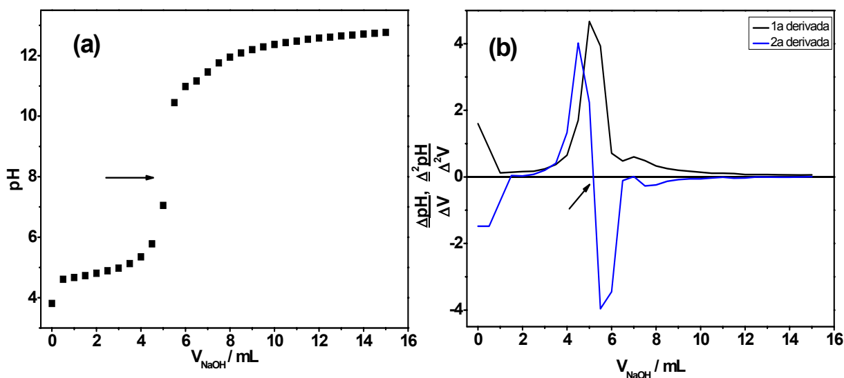
FIGURA 5.12: (a) Curva de pH para a titulação potenciométrica da solução de 0,05M \text{CuSO}_4 + 0,4M de sorbitol com solução de NaOH 0,9706M, (b) Curvas da 1ª e 2ª derivadas.
