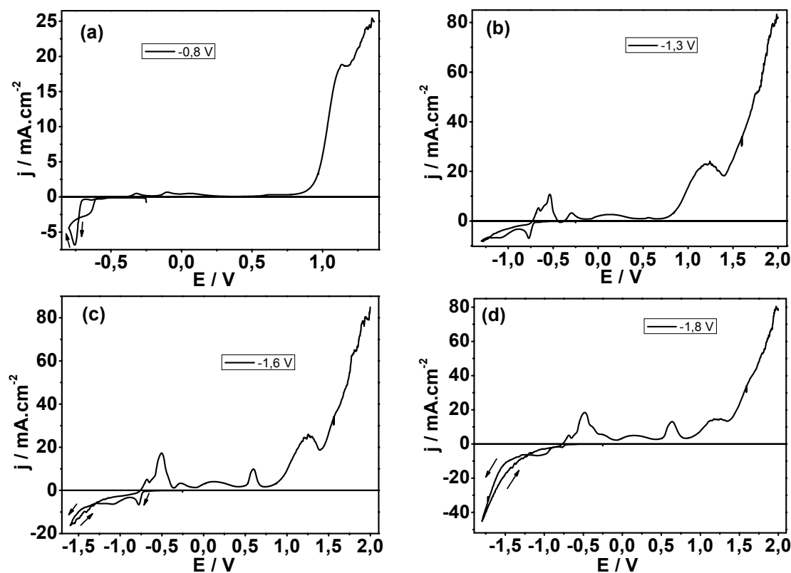
FIGURA 5.63: Curva voltamétrica do eletrodo de platina em 0,05M Pb(NO_3)_2 + 0,05M CuSO_4 + 0,1M EDTA e 0,4M NaOH; efeito do potencial limite: (a) -0,8 V, (b) -1,3 V, (c) -1,6 V e (d) -1,8 V, v = 10 \text{mV} \cdot \text{s}^{-1} .
