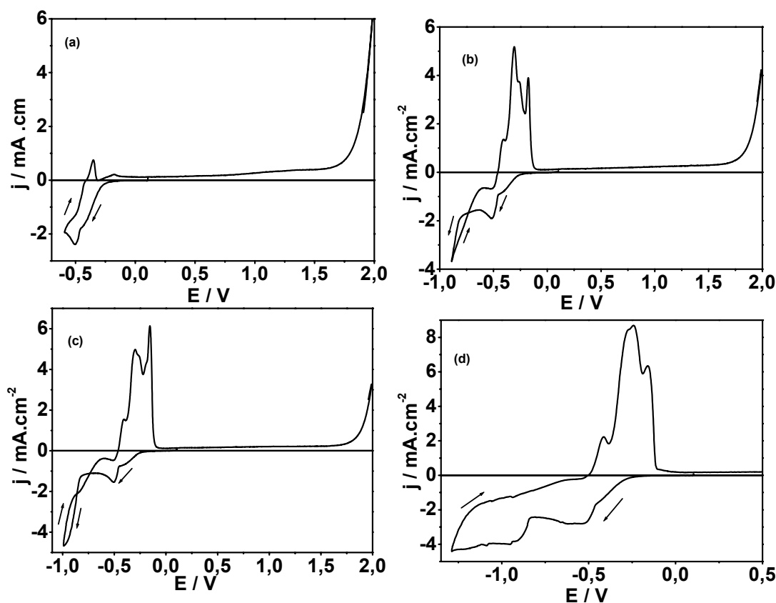
FIGURA 5.39: Curvas voltamétricas do eletrodo de platina em 0,05\text{M Pb}(\text{NO}_3)_2 + 0,05\text{M SnCl}_2 + 0,1\text{M EDTA} + 0,4\text{M NaOH} ; efeito do potencial limite: (a) -0,60\text{ V} , (b) -0,90\text{ V} , (c) -1,0\text{ V} e (d) -1,30\text{ V} , \nu = 10\text{mV s}^{-1} .
