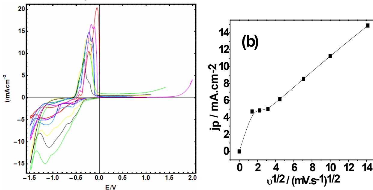
FIGURA 5.40. (a) Curvas voltamétricas do eletrodo de platina em 0,05M \text{Pb}(\text{NO}_3)_2 + 0,05M \text{SnCl}_2 + 0.1 M EDTA e 0,4 M NaOH em várias velocidades de varredura ( v / \text{mV s}^{-1} ): (—) 2,0 ; (—) 5,0 ; (—) 10 ; (—) 20 ; (—) 50; (—) 100; (—) 200. (b) Gráfico de j_p com v^{1/2} para (■) 2º pico.
