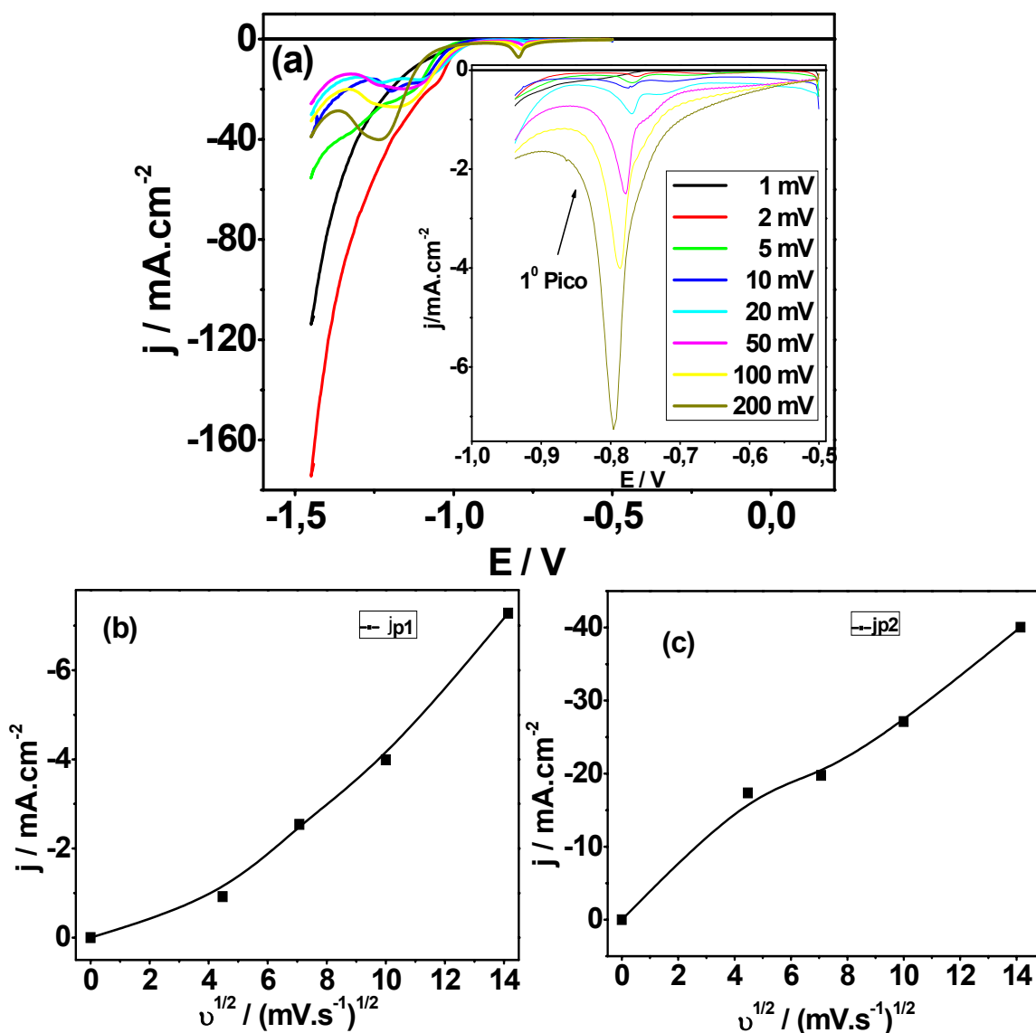
FIGURA 5.49. (a) Curvas voltamétricas do eletrodo de platina em 0,1\text{M Pb}(\text{NO}_3)_2 + 0,1\text{M CuSO}_4 + 0,2\text{M sorbitol} + 3,0\text{M NaOH} em várias velocidades de varredura ( v / \text{mV s}^{-1} ): (—) 1,0 ; (—) 2,0 ; (—) 5,0 ; (—) 10 ; (—) 20 ;
