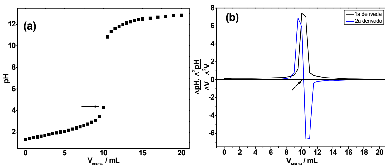
FIGURA 5.15: (a) Curva de pH para a titulação potenciométrica da solução de 0,05\text{M Pb}(\text{NO}_3)_2 + 0,05\text{M CuSO}_4 + 0,1\text{M} de EDTA com solução de NaOH 0,9706\text{M} , (b) Curvas da 1ª e 2ª derivadas.
