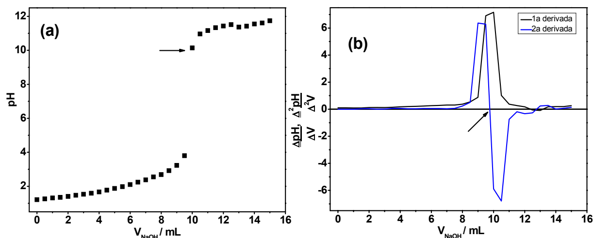
FIGURA 5.8 (a) Curva de pH para a titulação potenciométrica da solução de 0,05\text{M Pb}(\text{NO}_3)_2 + 0,05\text{M SnCl}_2 + 0,1\text{M} de EDTA com solução de NaOH 0,9706\text{M} , (b) Curvas da 1ª e 2ª derivadas.
