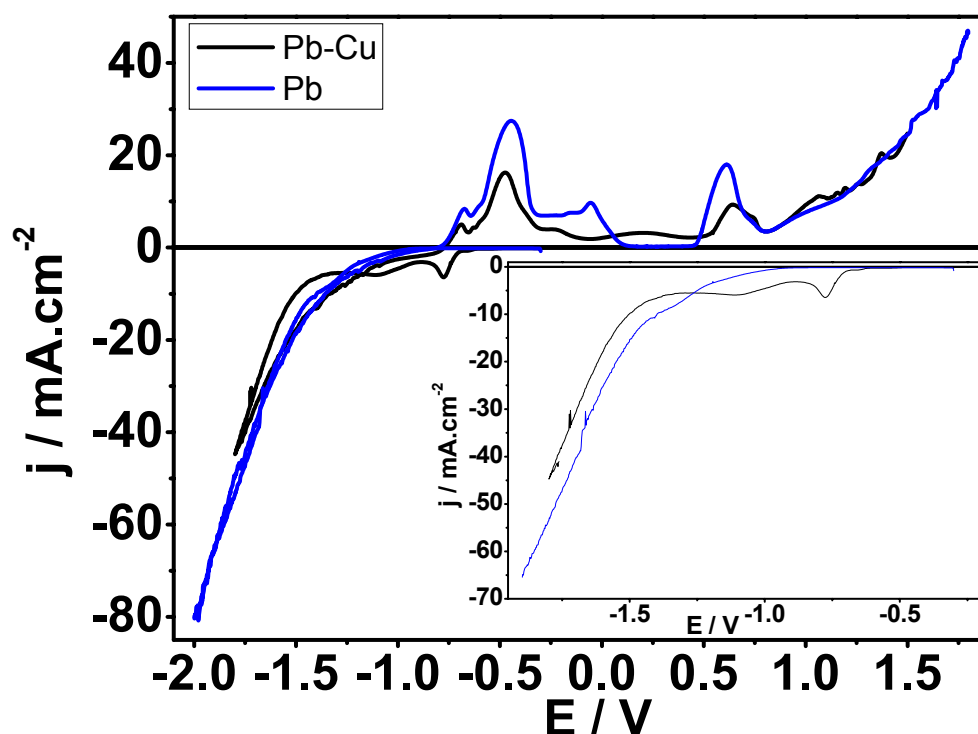
FIGURA 5.61: Curva voltamétrica do eletrodo de platina em 0,05\text{M Pb}(\text{NO}_3)_2 + 0,05\text{M CuSO}_4 + 0,1\text{M EDTA} + 0,4\text{M NaOH} (linha preta) e 0,05\text{M Pb}(\text{NO}_3)_2 + 0,1\text{M EDTA} + 0,4\text{M NaOH} (linha azul), v = 10\text{mV}\cdot\text{s}^{-1} .
