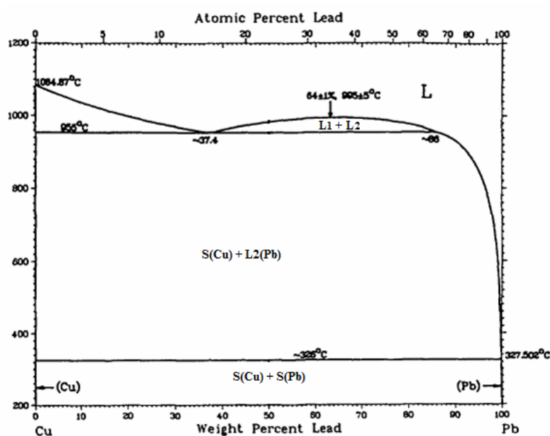
FIGURA 3.5 Diagrama de fases da liga Pb-Cu
