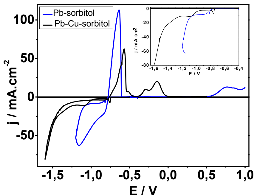
FIGURA 5.45: Curvas voltamétricas do eletrodo de platina em 0,1M Pb(NO_3)_2 + 0,1M CuSO_4 + 0,2M sorbitol e 3,0M NaOH (—) e 0,1M Pb(NO_3)_2 + 0,2M sorbitol e 3,0M NaOH (—), v = 10\text{mV s}^{-1} .
