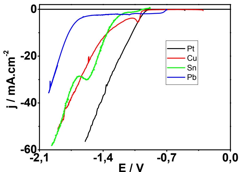
FIGURA 5.36: Curvas voltamétricas: (a) dos eletrodos de Pt, Pb, Sn, Cu, em 0,1M EDTA e 0,4M NaOH, v = 10\text{mV s}^{-1} .
