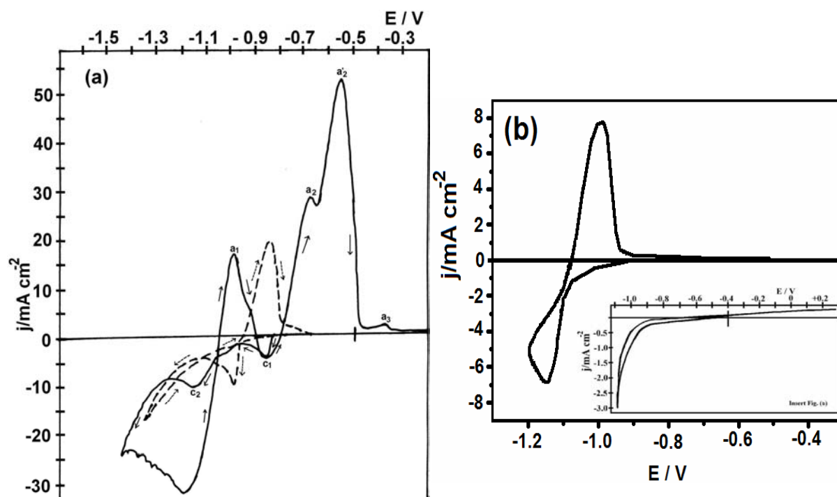
FIGURA 5.20: Curvas voltamétricas do eletrodo de platina em: (a) 0,05M \text{Pb}(\text{NO}_3)_2 + 0,05M \text{SnCl}_2 + 0,4M sorbitol e 0,8M NaOH (—) e 0,05M \text{SnCl}_2 + 0,4M sorbitol e 0,8M NaOH (----), (b) 0,05M \text{SnCl}_2 + 0,4M sorbitol + 0,8M NaOH, v = 10\text{mV s}^{-1} .
