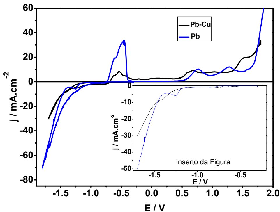
FIGURA 5.54: Curva voltamétrica do eletrodo de platina em 0,05M \text{Pb}(\text{NO}_3)_2 + 0,05M \text{CuSO}_4 + 0,1M \text{NaKC}_4\text{H}_4\text{O}_6 e 0,4M \text{NaOH} (linha preta) e 0,05M \text{Pb}(\text{NO}_3)_2 + 0,1M \text{NaKC}_4\text{H}_4\text{O}_6 e 0,4M \text{NaOH} (linha azul), \nu = 10\text{mV}\cdot\text{s}^{-1} .
