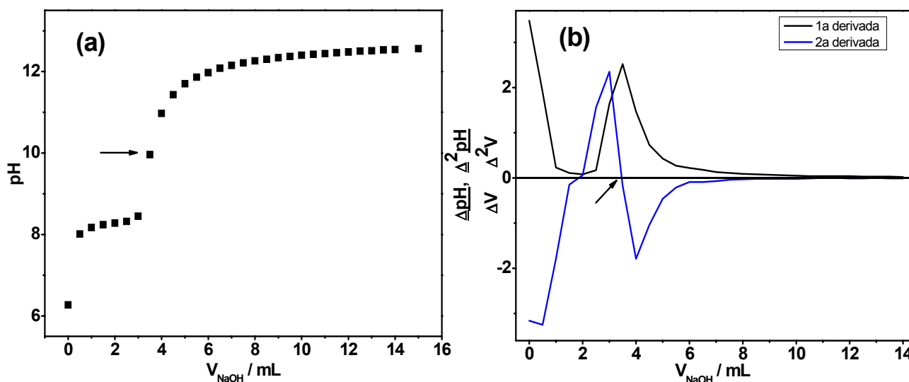
FIGURA 5.9 (a) Curva de pH para a titulação potenciométrica da solução de 0,05M \text{Pb}(\text{NO}_3)_2 + 0,1\text{M NaKC}_4\text{H}_4\text{O}_6 com solução de \text{NaOH} 0,9706M, (b) Curvas da 1ª e 2ª derivadas.
