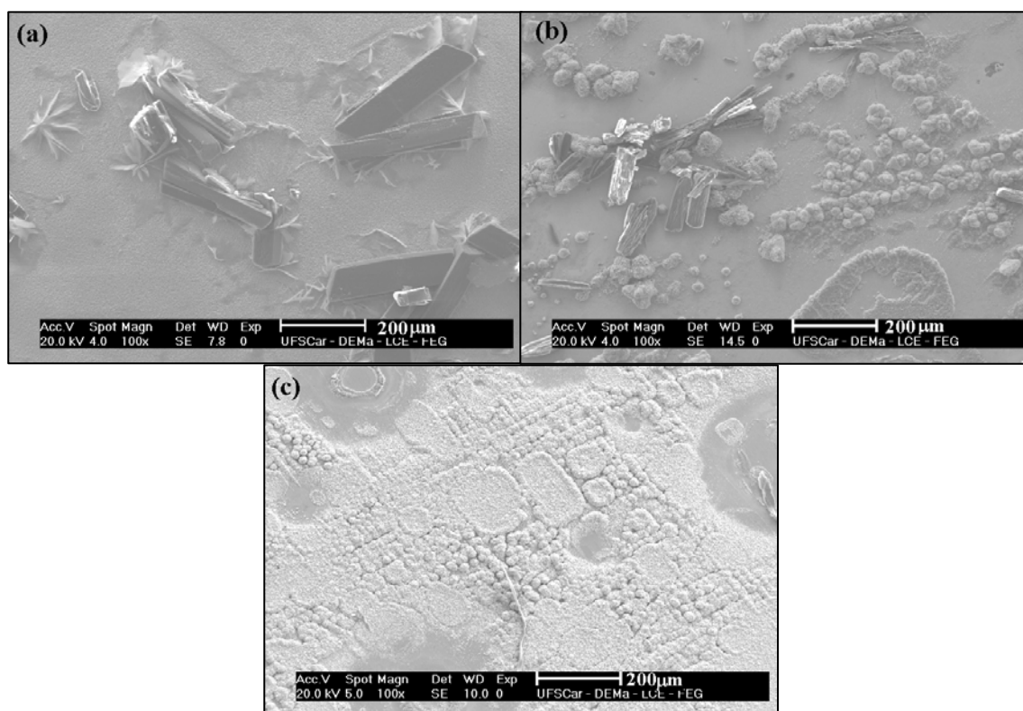
FIGURA 5.42 – MEV dos filmes de Pb-Sn, obtidos cronamperometricamente: (a) de 0,0 V para -0,560 V, com q_d = 5 \text{ C.cm}^{-2} , de -0,0 V para -1,10 V, (b) com q_d = 1 \text{ C.cm}^{-2} e (c) com q_d = 10 \text{ C.cm}^{-2} . Solução de deposição: 0,05 \text{ M Pb(NO}_3)_2 + 0,05 \text{ M SnCl}_2 + 0,1 \text{ M EDTA} + 0,4 \text{ M NaOH} .
