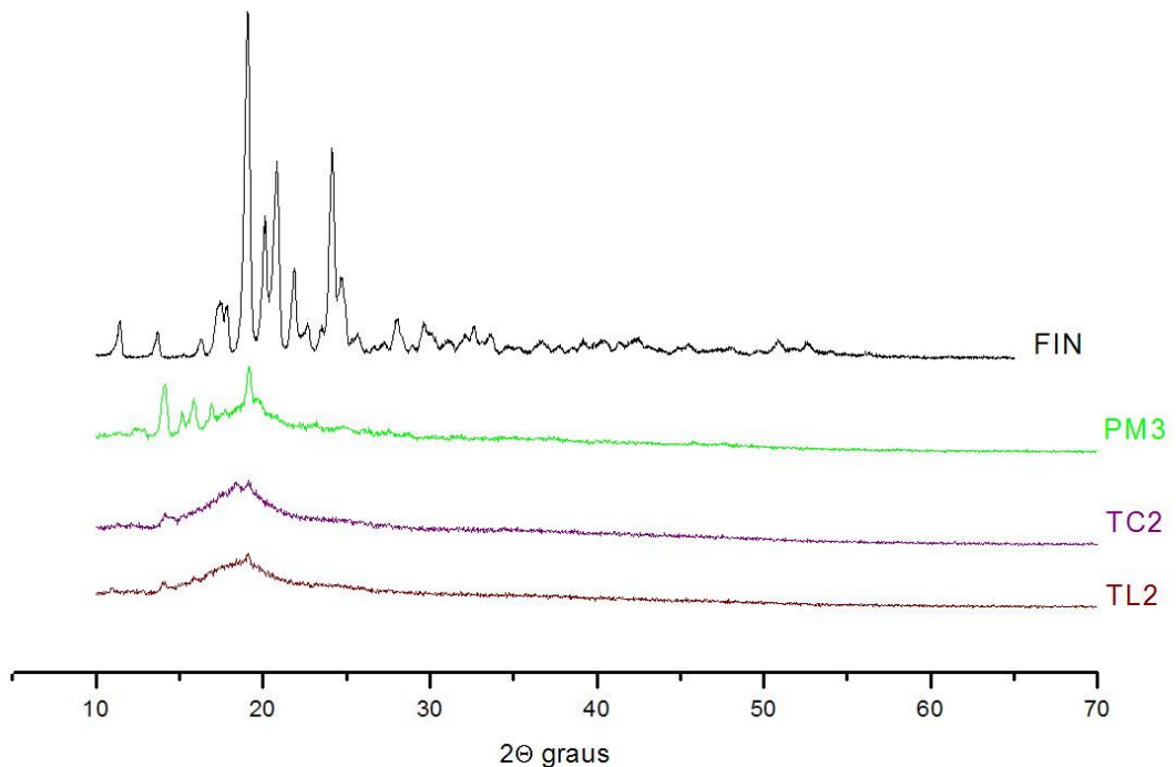
FIGURA 23 - DIFRATOGRAMAS OBTIDOS PARA A FINASTERIDA (FIN), MISTURA-FÍSICA FINASTERIDA:HPβCD:PVP K-30 (PM3) E SISTEMAS TERNÁRIOS OBTIDOS POR COEVAPORAÇÃO (TC2) E LIOFILIZAÇÃO (TL2), OPERANDO A 40 KV E 40 MA, COM VELOCIDADE DE VARREDURA DE 2 GRAUS/MINUTO (2 THETA)
