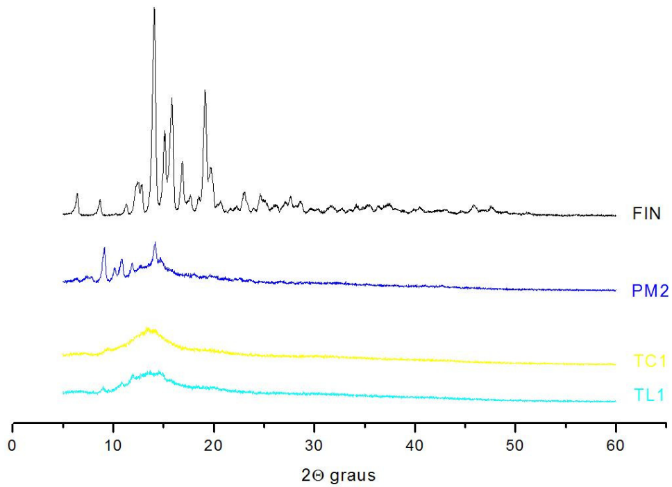
FIGURA 22 - DIFRATOGRAMAS OBTIDOS PARA A FINASTERIDA (FIN); MISTURA-FÍSICA FINASTERIDA:HPβCD:QUITOSANA (PM2) E SISTEMAS TERNÁRIOS OBTIDOS POR COEVAPORAÇÃO (TC1) E LIOFILIZAÇÃO (TL1), OPERANDO A 40 KV E 40 MA, COM VELOCIDADE DE VARREDURA DE 2 GRAUS/MINUTO (2 THETA)
