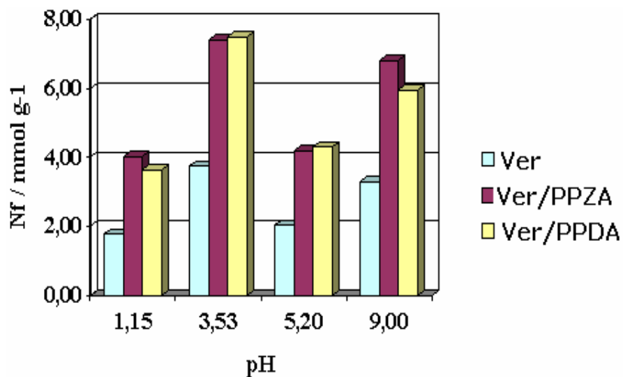
Figura 3.18. Comparação da adsorção de chumbo em vermiculita (Ver), modificada com piperazina (Ver/PPZA) e com piperidina (Ver/PPDA) em vários pH a 298 K e 1 atm.
