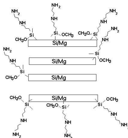
Figura 1.7. Esquema genérico da organofuncionalização de silicatos lamelares [4].
