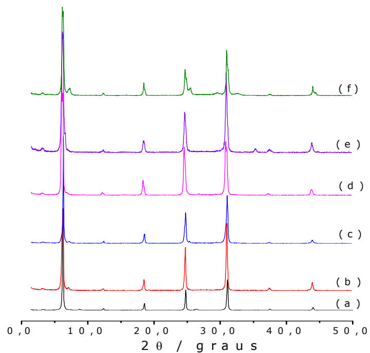
Figura 3.9. Difratomogramas de Raios-X para (a) vermiculita e do híbrido Ver/PPZA em mmol g -1 (b) 0,41; (c) 0,46; (d) 0,48; (e) 0,49 e (f) 0,52.
