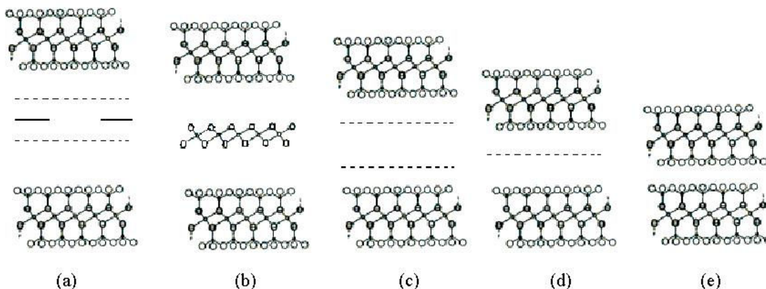
Figura 3.12. Várias fases de hidratação para a vermiculita: (a) 1481 pm, (b) 1436 pm, (c) 1382 pm, (d) 1159 pm e (e) 902 pm.
