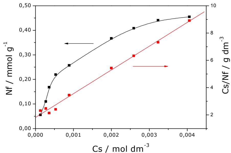
Figura 3.21. Isoterma de intercalação de Ver/BUTIL e sua linearização a 298 K e 1 atm.
