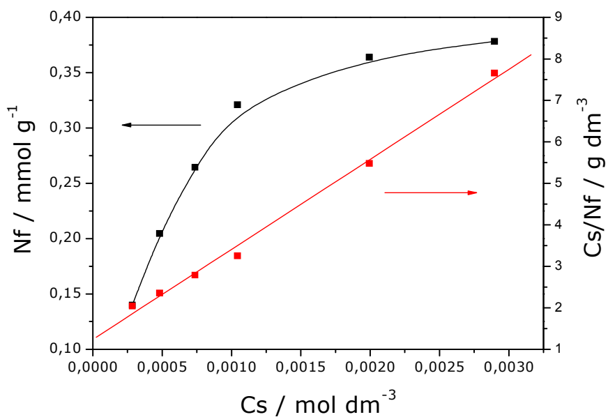
Figura 3.22. Isoterma de intercalação de Ver/HEXIL e sua linearização a 298 K e 1 atm.
