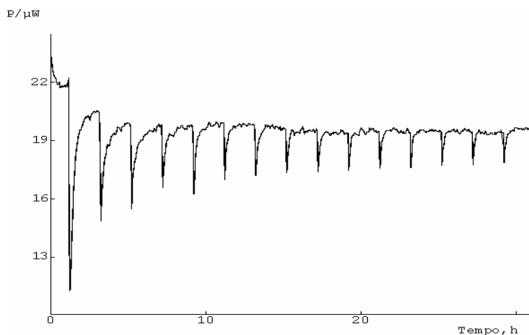
Figura 2.5. Ilustração de uma curva potência versus tempo onde se observam os efeitos térmicos resultantes da titulação.
