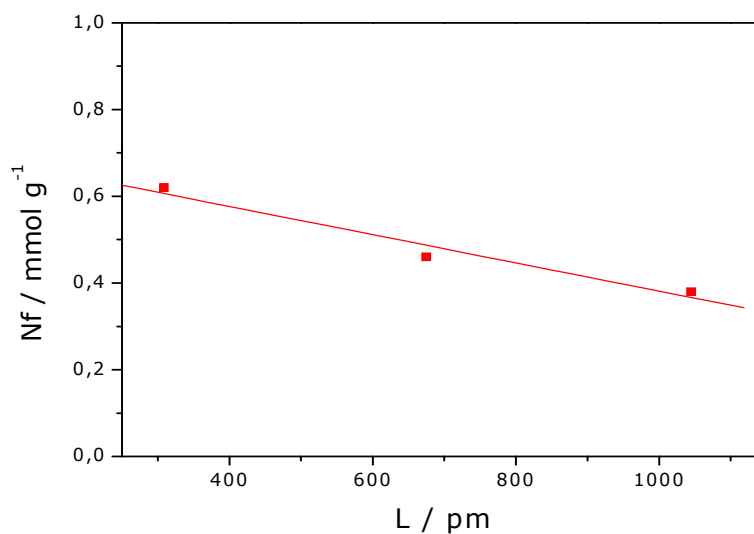
Figura 3.23. Correlação entre a quantidade máxima de amina intercalada dentro do espaço lamelar da vermiculita com o comprimento de cadeia orgânica.
