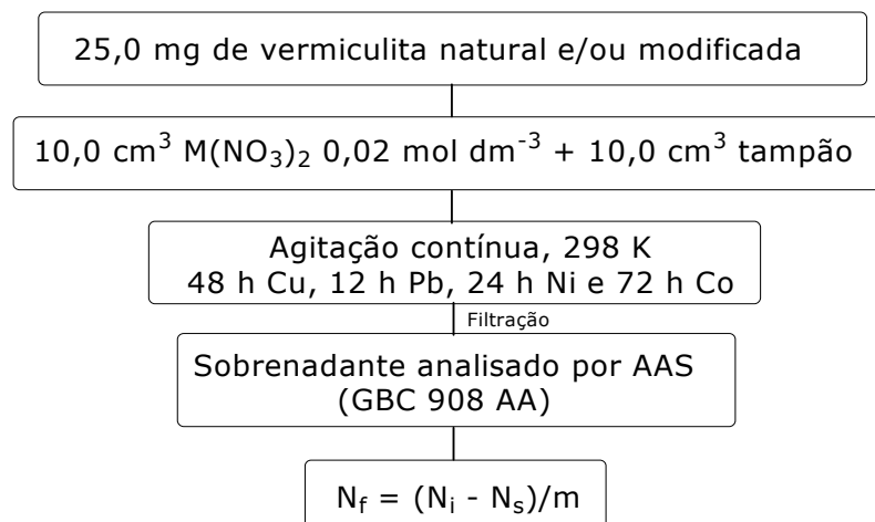
Figura 2.2. Representação do procedimento aplicado para adsorção de metais a diferentes pH em vermiculita modificada.
