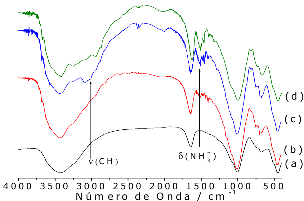
Figura 3.25. Espectros de absorção na região do infravermelho para (a) vermiculita, e dos híbridos (b) Ver/ETIL, (c) Ver/BUTIL e Ver/HEXIL.
