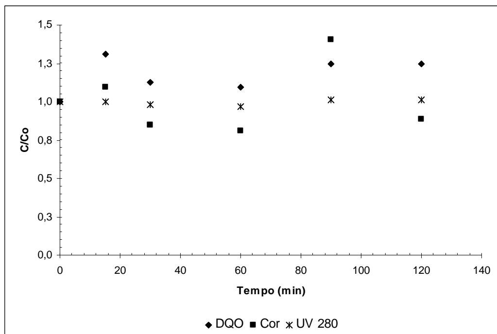
Figura 5-15 – Cinética de degradação do efluente de curtume na presença do Birm® para diferentes parâmetros operacionais. Condições experimentais: pH_0 = 3 e [Birm®]_0 = 12 g/L.
