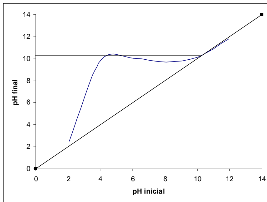
Figura 5-4 – Determinação do ponto de carga zero (pH pcz ) do Birm®
