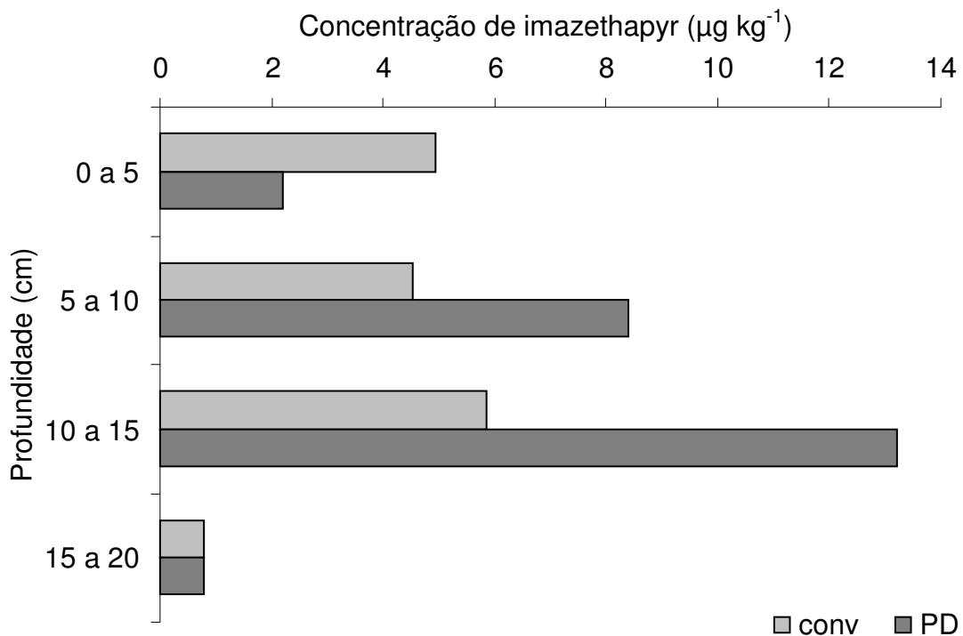
Figura 4 – Concentração de imazethapyr expressa em \mu\text{g} de ingrediente ativo por \text{kg} de solo ( \mu\text{g kg}^{-1} ), para dois manejos de solo, plantio convencional (PC) e plantio direto (PD) e quatro profundidades 0-5, 5-10; 10-15 e 15-20 cm após a coleta do arroz no terceiro ano num sistema de rotação dois anos arroz Clearfield e um ano arroz convencional.
