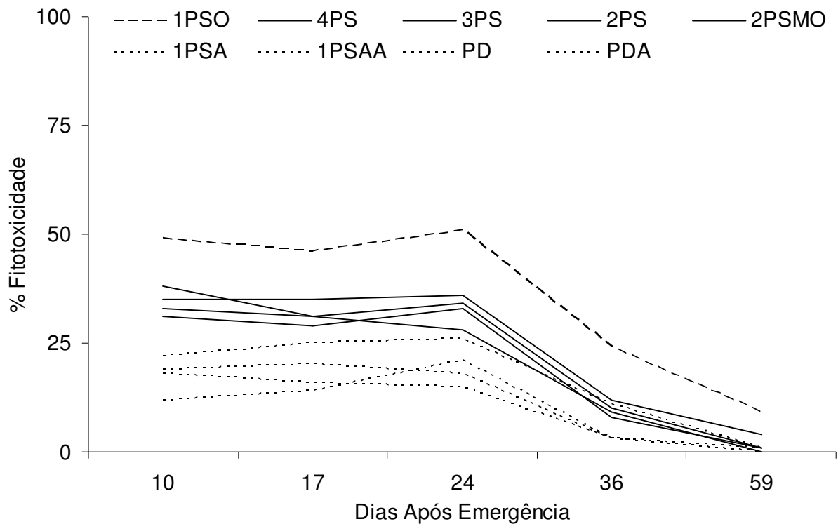
Figura 3 - Fitotoxicidade da mistura formulada de imazethapyr e imazapic ( 75+25 \text{ g ha}^{-1} ) na cultivar IRGA 417 semeada após um ano da última aplicação dos herbicidas, num sistema com dois anos de uso dos herbicidas, em cinco épocas de avaliação e nove preparos de solos: plantio direto (PD); plantio direto mais azevém (PDA); um preparo de solo (PS) em abril (1PSA); um PS em abril mais azevém (1PSAA); um PS em outubro (1PSO); dois PS em maio e outubro (2PSMO); dois PS em abril e outubro (2PS); três PS em abril, maio e outubro (3PS); quatro PS em abril, maio, agosto e outubro (4PS). Santa Maria, RS, 2006/07.
