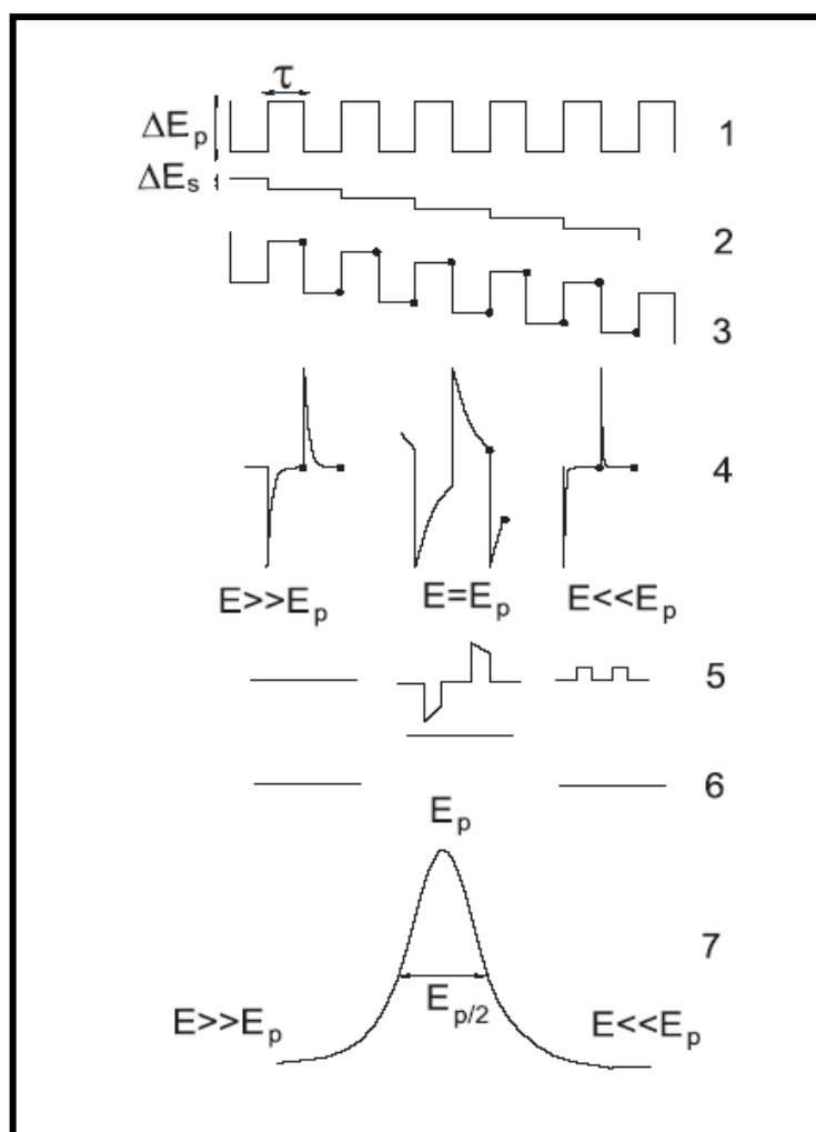
Figura 1.8 - Representação esquemática da voltametria de onda quadrada, onde: 1) potencial na forma de onda; 2) escada de potencial; 3) forma de aplicação do potencial na SWV; 4) forma da onda da corrente; 5) sinal da corrente; 6) corrente diferencial e 7) corrente total 81 .
