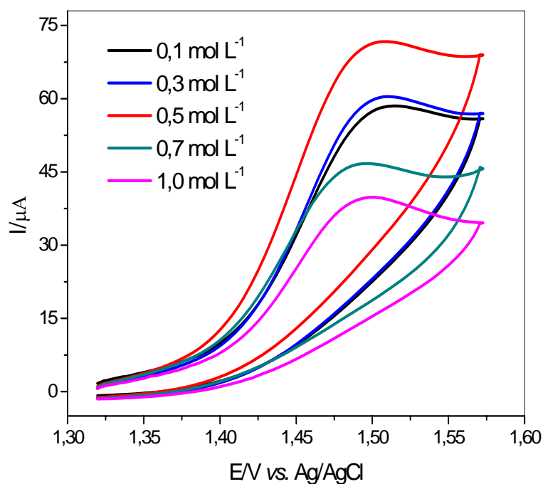
Figura 3.4 - Voltamogramas cíclicos obtidos para o aspartame em diferentes concentrações do eletrólito suporte ácido sulfúrico ( \text{H}_2\text{SO}_4 ). ( [\text{Aspartame}] = 5,0 \times 10^{-5} \text{ mol L}^{-1} , v = 50 \text{ mV s}^{-1} ).
