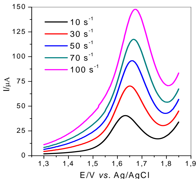
Figura 3.8 - Influência da variação da frequência de aplicação dos pulsos de potencial no aspecto geral dos voltamogramas do aspartame ( 1,0 \times 10^{-4} \text{ mol L}^{-1} , a = 40 \text{ mV} , \Delta E_s = 2 \text{ mV} , \text{H}_2\text{SO}_4 \text{ } 0,5 \text{ mol L}^{-1} ).
