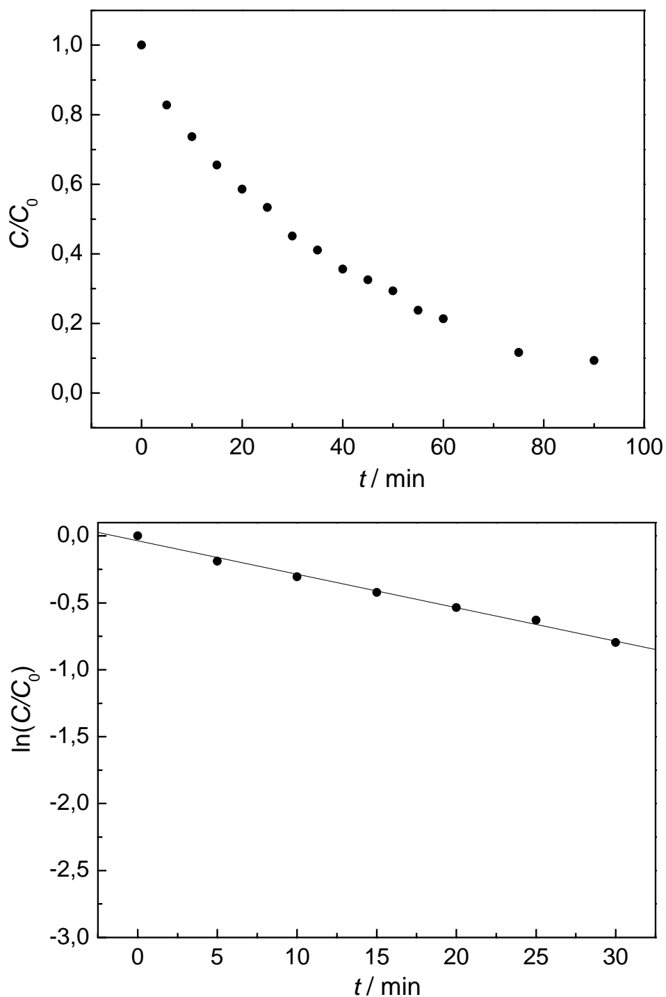
Figura A4 – (a) Concentração de Pb(II) normalizada vs. tempo para experimento de remoção eletrolítica de Pb(II) para o nível codificado (+1, +1) utilizado no planejamento fatorial completo 2^2 com esponja de aço inoxidável de menor massa; (b) Logaritmo neperiano da concentração normalizada de Pb(II) vs. tempo para 30 minutos de eletrólise; Solução: \text{NaNO}_3 0,10 \text{ mol L}^{-1} + \text{H}_3\text{BO}_3 0,10 \text{ mol L}^{-1} + 50 \text{ mg L}^{-1} de Pb(II); (pH 4,8).
