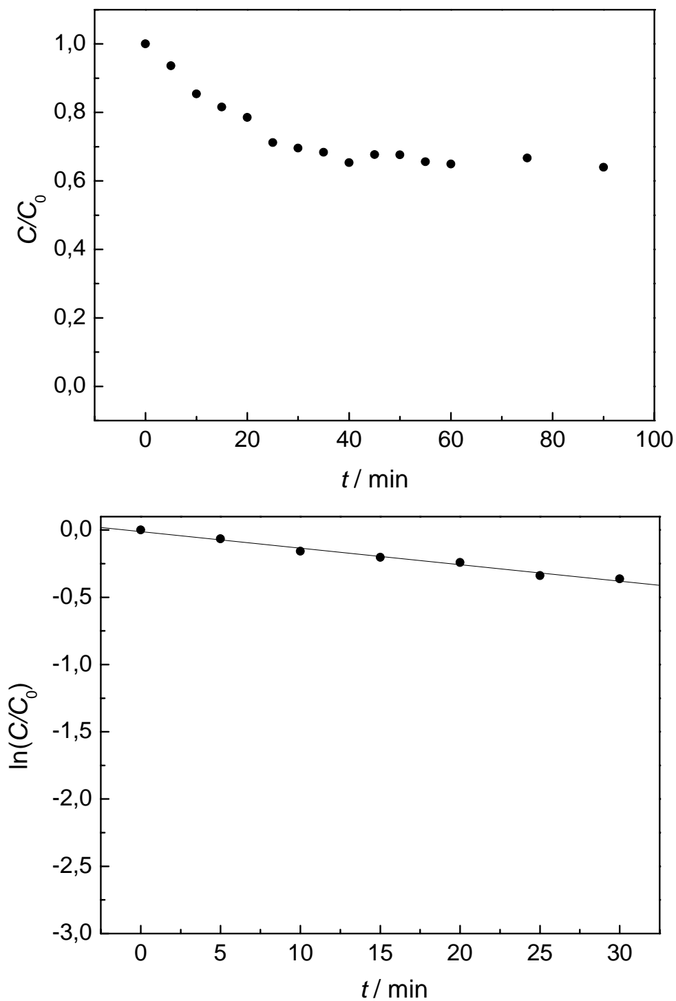
Figura A11 – (a) Concentração de Pb(II) normalizada vs. tempo para experimento de remoção eletrolítica de Pb(II) para o nível codificado (-1, +1) utilizado no planejamento fatorial composto central; (b) Logaritmo neperiano da concentração normalizada de Pb(II) vs. tempo para 30 minutos de eletrólise; Solução: \text{NaNO}_3 0,10 \text{ mol L}^{-1} + \text{H}_3\text{BO}_3 0,10 \text{ mol L}^{-1} + 50 \text{ mg L}^{-1} de Pb(II); (pH 4,8).
