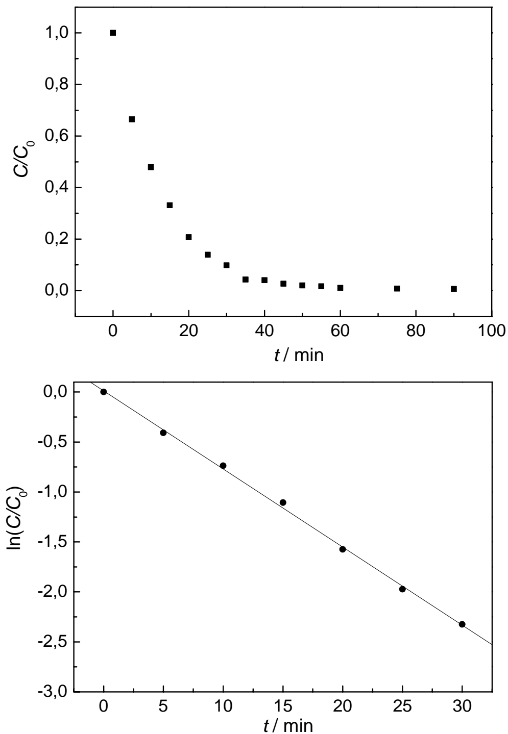
Figura A8 – (a) Concentração de Pb(II) normalizada vs. tempo para experimento de remoção eletrolítica de Pb(II) para o nível codificado (+1, +1) utilizado no planejamento fatorial completo 2^2 com esponja de aço inoxidável de maior massa; (b) Logaritmo neperiano da concentração normalizada de Pb(II) vs. tempo para 30 minutos de eletrólise; Solução: \text{NaNO}_3 0,10 \text{ mol L}^{-1} + \text{H}_3\text{BO}_3 0,10 \text{ mol L}^{-1} + 50 \text{ mg L}^{-1} de Pb(II); (pH 4,8).
