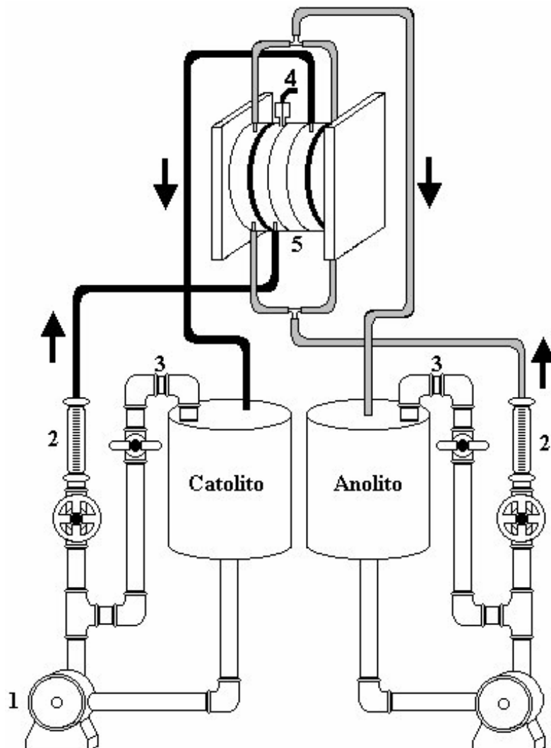
FIGURA 3.1 – Representação esquemática do sistema de recirculação construído para remoção de íons Pb(II): 1) bombas, 2) medidores de vazão, 3) desvios, 4) eletrodo de referência (ECS) e 5) reator eletroquímico.
