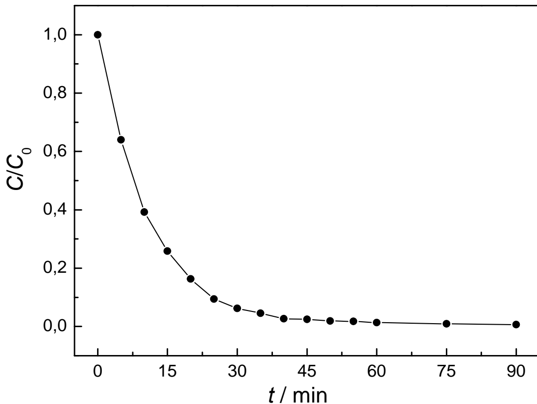
FIGURA 4.12 – Concentração de Pb(II) normalizada vs. tempo de eletrólise aplicando-se uma corrente de -0,25 \text{ A} e um fluxo de 250 \text{ L h}^{-1} (ponto ótimo) a uma esponja de aço inoxidável de um reator eletroquímico operando em configuração “flow-through”. Solução: \text{NaNO}_3 0,10 \text{ mol L}^{-1} + \text{H}_3\text{BO}_3 0,10 \text{ mol L}^{-1} + 50 \text{ ppm de Pb(II)} (pH 4,8).
