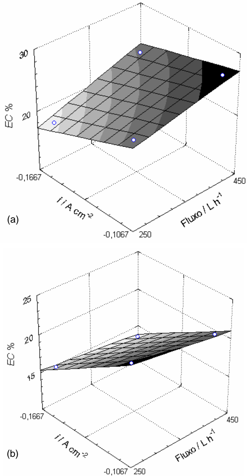
FIGURA 4.4 – Superfícies de respostas para eficiência de corrente (EC) ajustadas aos dados do planejamento fatorial completo 2^2 , utilizando esponjas de aço inoxidável de (a) menor (8,024 g) e (b) maior (18,004 g) massa, após 30 minutos de eletrólise.
