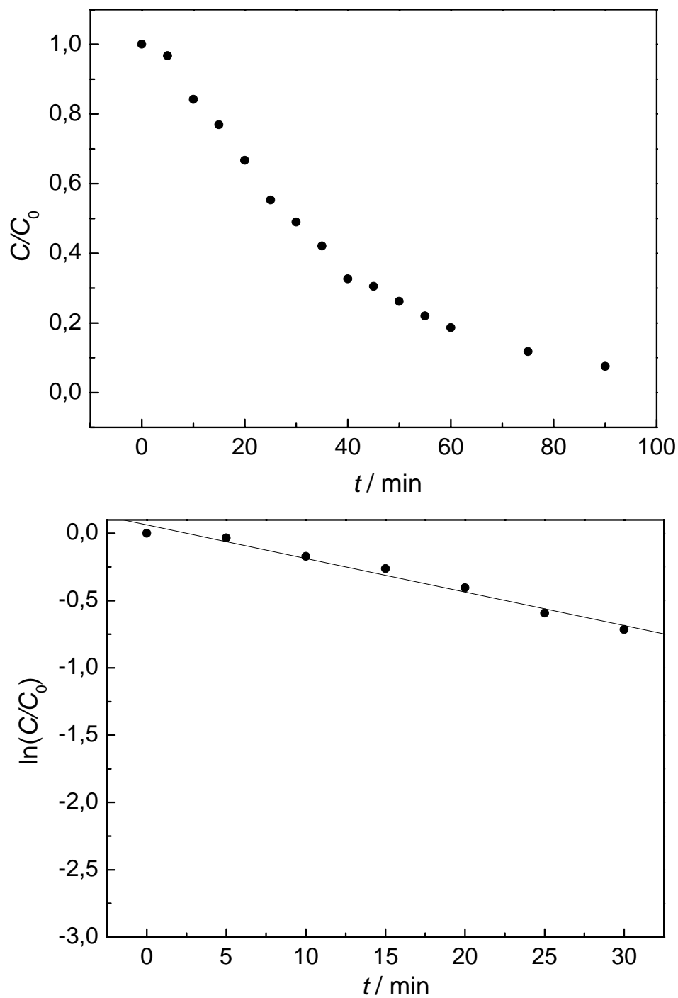
Figura A2 – (a) Concentração de Pb(II) normalizada vs. tempo para experimento de remoção eletrolítica de Pb(II) para o nível codificado (+1, -1) utilizado no planejamento fatorial completo 2^2 com esponja de aço inoxidável de menor massa; (b) Logaritmo neperiano da concentração normalizada de Pb(II) vs. tempo para 30 minutos de eletrólise; Solução: \text{NaNO}_3 0,10 \text{ mol L}^{-1} + \text{H}_3\text{BO}_3 0,10 \text{ mol L}^{-1} + 50 \text{ mg L}^{-1} de Pb(II); (pH 4,8).
