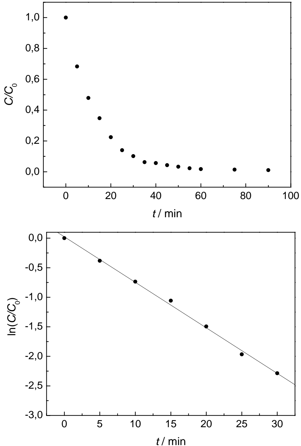
Figura A14 – (a) Concentração de Pb(II) normalizada vs. tempo para experimento de remoção eletrolítica de Pb(II) para o nível codificado (+1, +1) utilizado no planejamento fatorial composto central; (b) Logaritmo neperiano da concentração normalizada de Pb(II) vs. tempo para 30 minutos de eletrólise; Solução: \text{NaNO}_3 0,10 \text{ mol L}^{-1} + \text{H}_3\text{BO}_3 0,10 \text{ mol L}^{-1} + 50 \text{ mg L}^{-1} de Pb(II); (pH 4,8).
