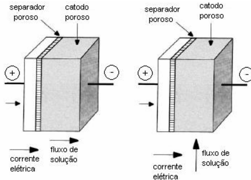
FIGURA 1.2 – Diferentes configurações de reatores de fluxo: a) “flow-through” e b) “flow-by” (KOENE e JANSSEN, 2001).
