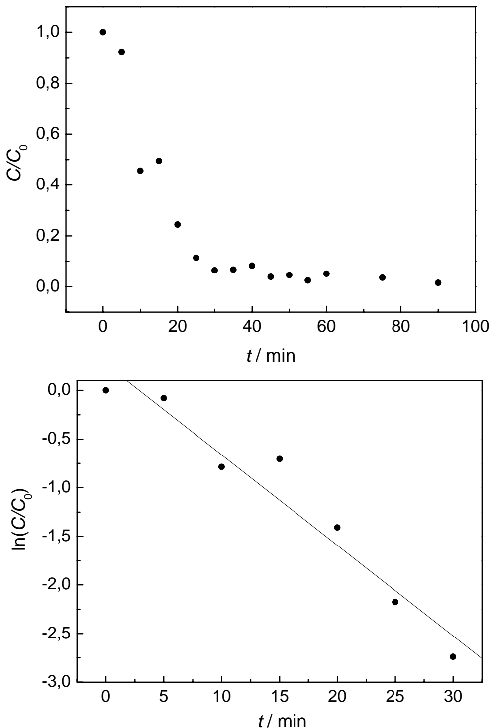
Figura A17 – (a) Concentração de Pb(II) normalizada vs. tempo para experimento de remoção eletrolítica de Pb(II) para o nível codificado (0, 0) utilizado no planejamento fatorial composto central; (b) Logaritmo neperiano da concentração normalizada de Pb(II) vs. tempo para 30 minutos de eletrólise; Solução: \text{NaNO}_3 0,10 \text{ mol L}^{-1} + \text{H}_3\text{BO}_3 0,10 \text{ mol L}^{-1} + 50 \text{ mg L}^{-1} de Pb(II); (pH 4,8).
