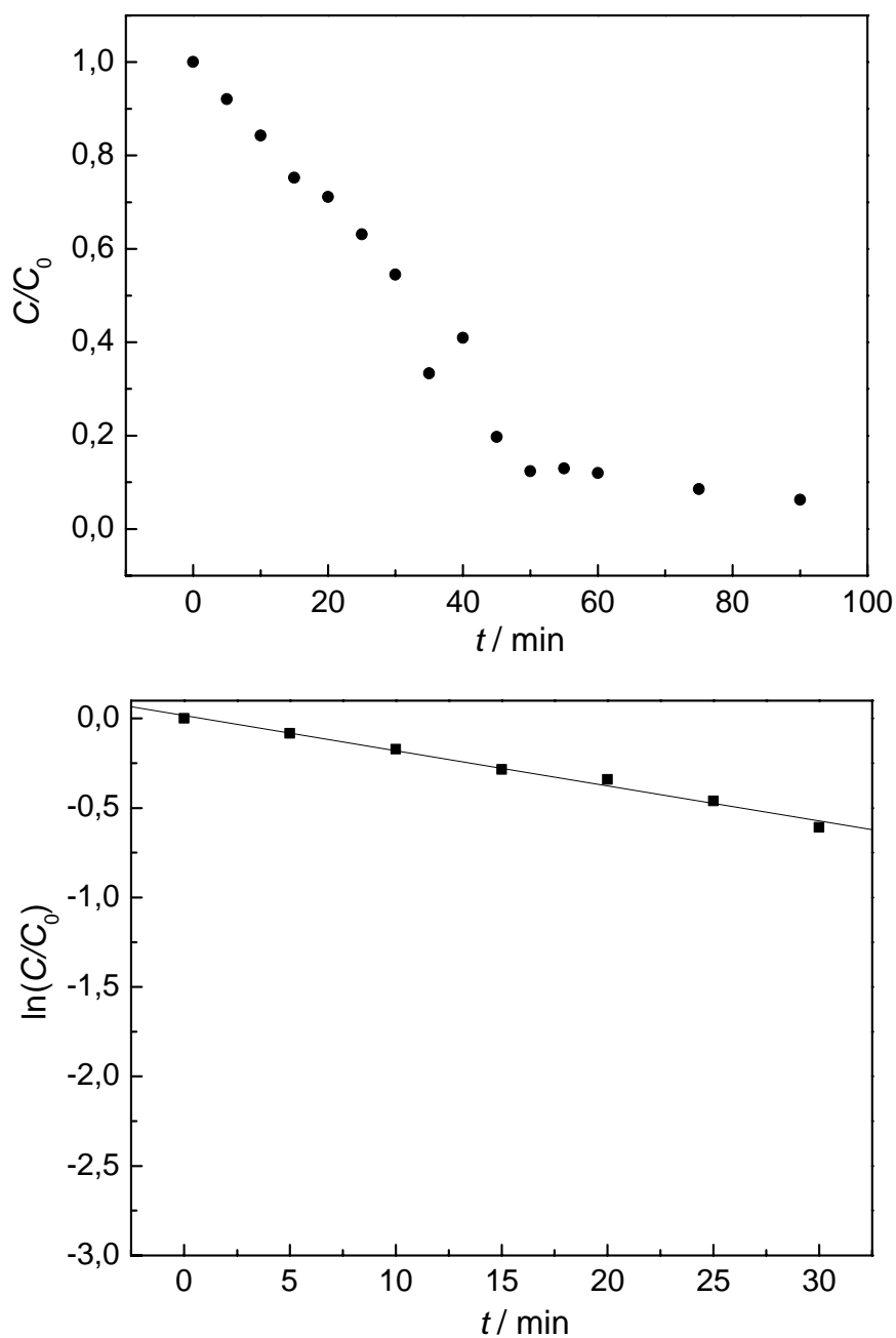
Figura A1 – (a) Concentração de Pb(II) normalizada vs. tempo para experimento de remoção eletrolítica de Pb(II) para o nível codificado (-1, -1) utilizado no planejamento fatorial completo 2^2 com esponja de aço inoxidável de menor massa; (b) Logaritmo neperiano da concentração normalizada de Pb(II) vs. tempo para 30 minutos de eletrólise; Solução: \text{NaNO}_3 0,10 \text{ mol L}^{-1} + \text{H}_3\text{BO}_3 0,10 \text{ mol L}^{-1} + 50 \text{ mg L}^{-1} de Pb(II); (pH 4,8).
