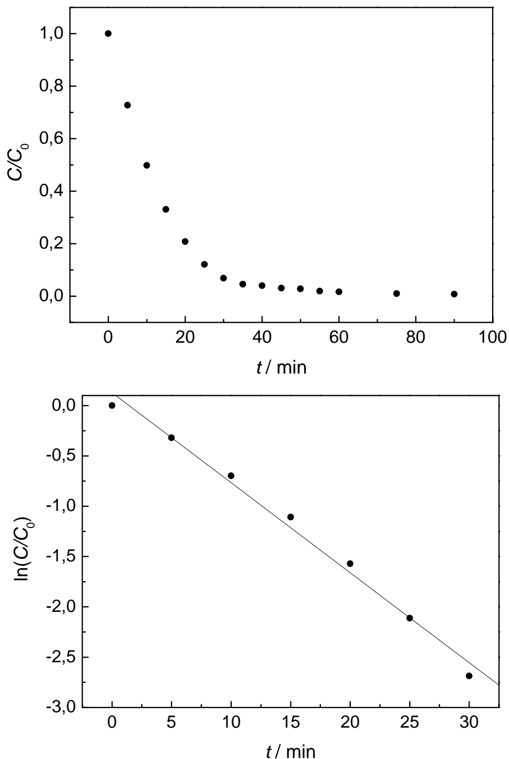
Figura A16 – (a) Concentração de Pb(II) normalizada vs. tempo para experimento de remoção eletrolítica de Pb(II) para o nível codificado (+1,41, 0) utilizado no planejamento fatorial composto central; (b) Logaritmo neperiano da concentração normalizada de Pb(II) vs. tempo para 30 minutos de eletrólise; Solução: \text{NaNO}_3 0,10 mol \text{L}^{-1} + \text{H}_3\text{BO}_3 0,10 mol \text{L}^{-1} + 50 mg \text{L}^{-1} de Pb(II); (pH 4,8).
