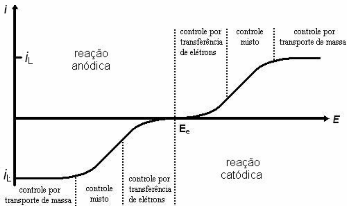
FIGURA 1.3 – Curva de densidade de corrente em função do potencial para diferentes regiões de controle cinético.
