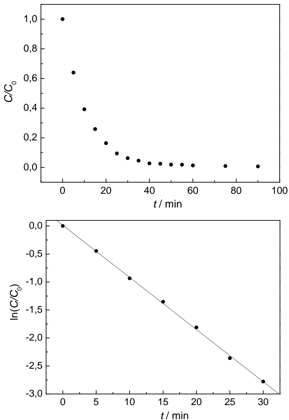
Figura A6 – (a) Concentração de Pb(II) normalizada vs. tempo para experimento de remoção eletrolítica de Pb(II) para o nível codificado (+1, -1) utilizado no planejamento fatorial completo 2^2 com esponja de aço inoxidável de maior massa; (b) Logaritmo neperiano da concentração normalizada de Pb(II) vs. tempo para 30 minutos de eletrólise; Solução: \text{NaNO}_3 0,10 \text{ mol L}^{-1} + \text{H}_3\text{BO}_3 0,10 \text{ mol L}^{-1} + 50 \text{ mg L}^{-1} de Pb(II); (pH 4,8).
