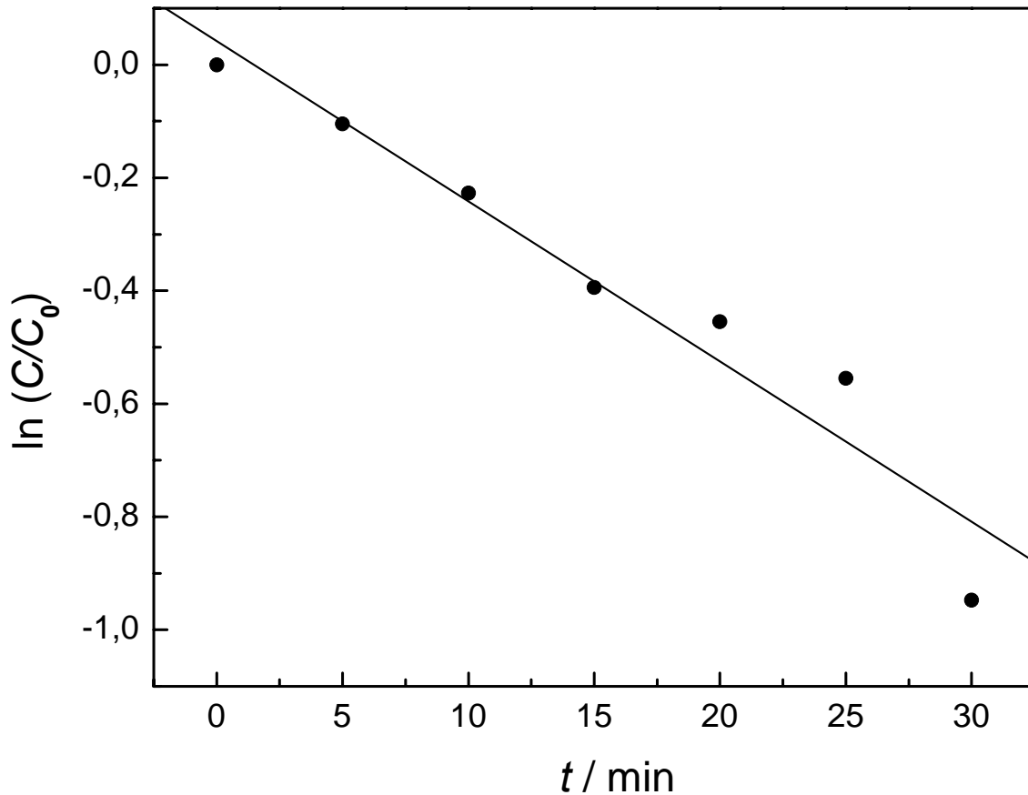
FIGURA 4.10 – Logaritmo neperiano da concentração normalizada de Pb(II) vs. tempo para 30 minutos de eletrólise correspondente à Figura 4.9.
