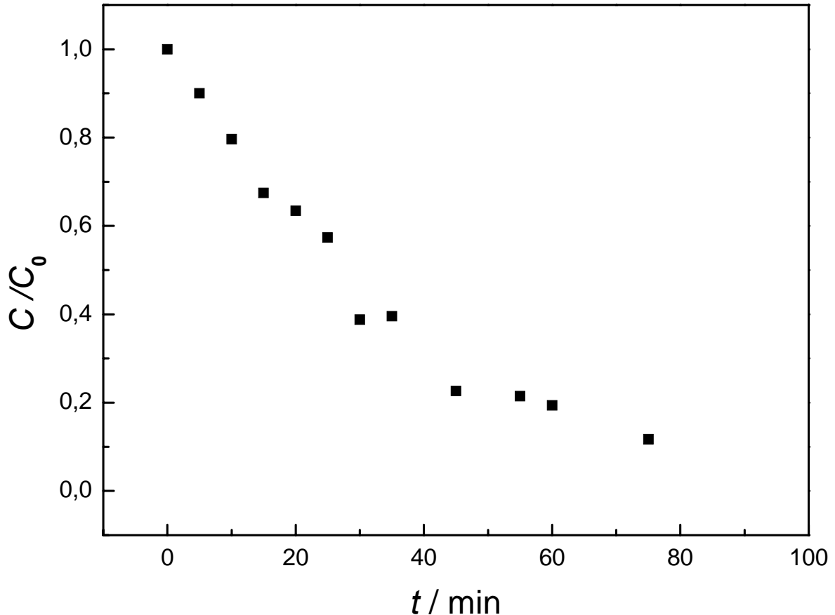
FIGURA 4.9 – Concentração de Pb(II) normalizada vs. tempo de eletrólise aplicando-se uma corrente de -0,14 \text{ A} e um fluxo de 250 \text{ L h}^{-1} a uma esponja de aço inoxidável de um reator eletroquímico operando em configuração “flow-through”. Solução: \text{NaNO}_3 0,10 \text{ mol L}^{-1} + \text{H}_3\text{BO}_3 0,10 \text{ mol L}^{-1} + 50 \text{ mg L}^{-1} de Pb(II) (pH 4,8).
