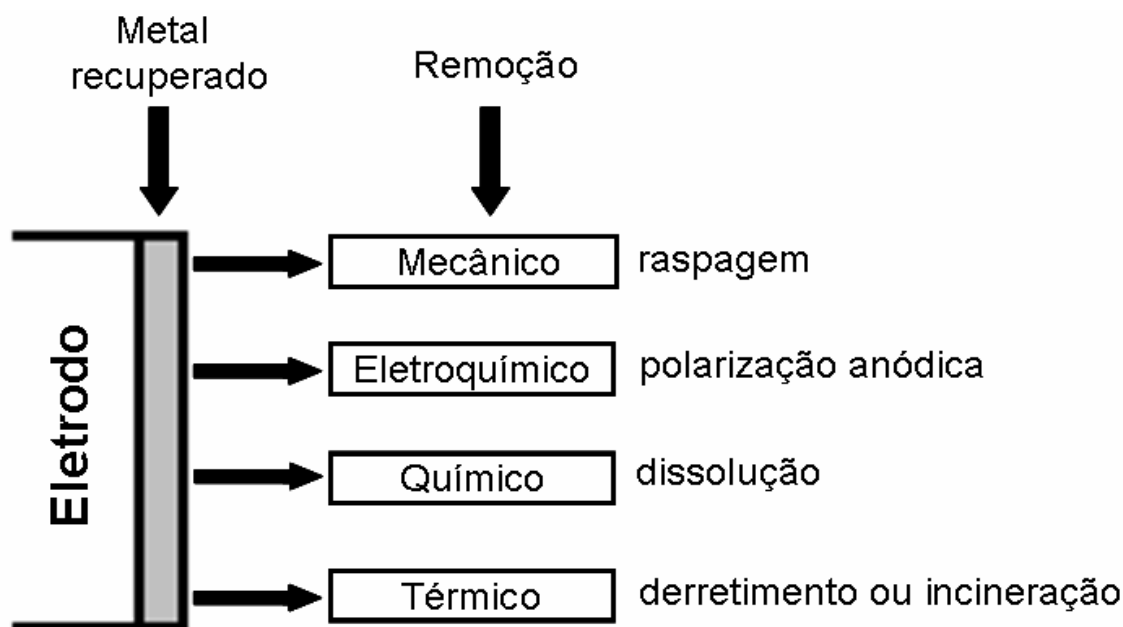
FIGURA 1.4 – Processos utilizados para remoção de metais eletrodepositados.
