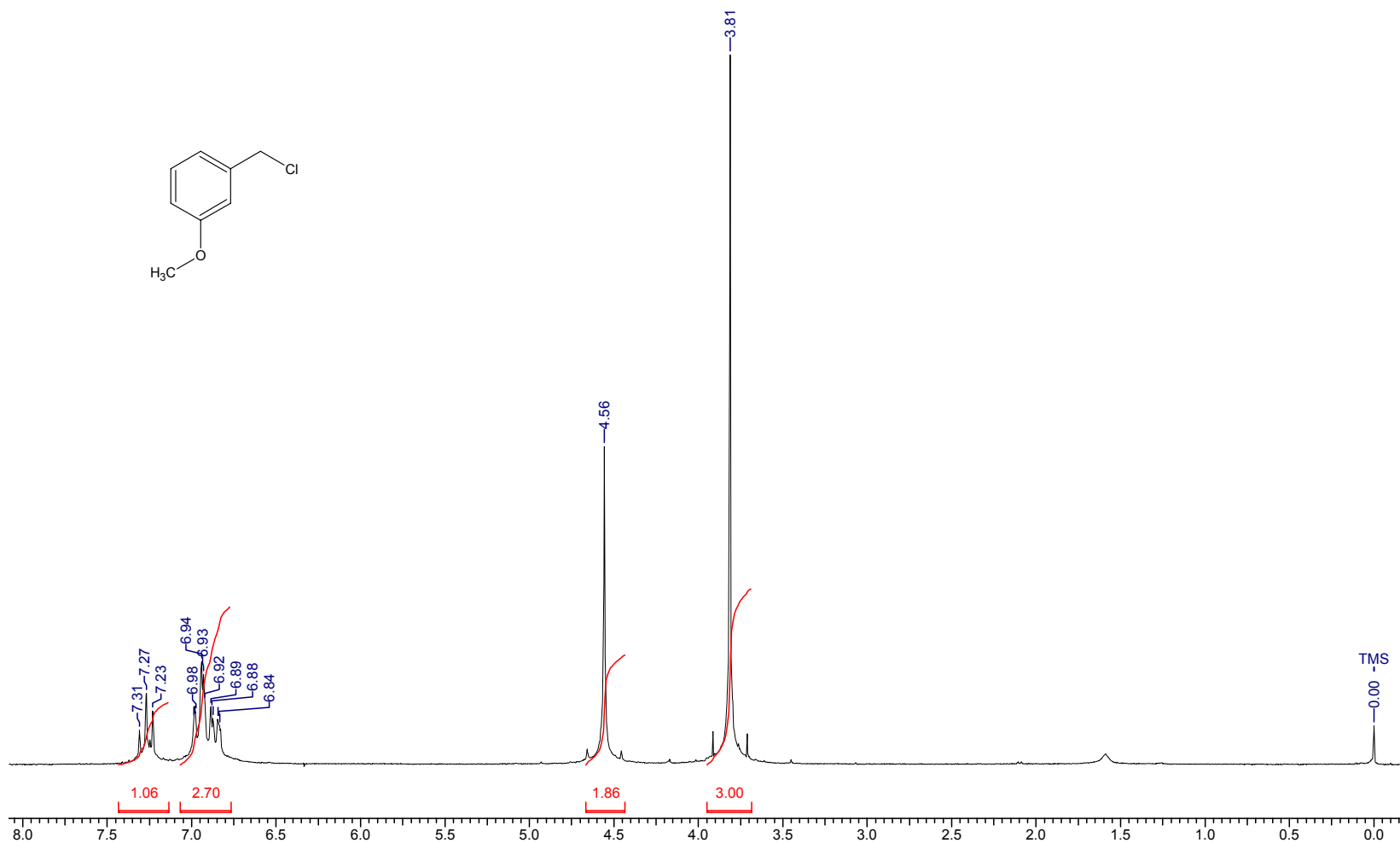
Espectro de RMN ^1\text{H} do 1-(clorometil)-3-metoxibenzeno (10)
