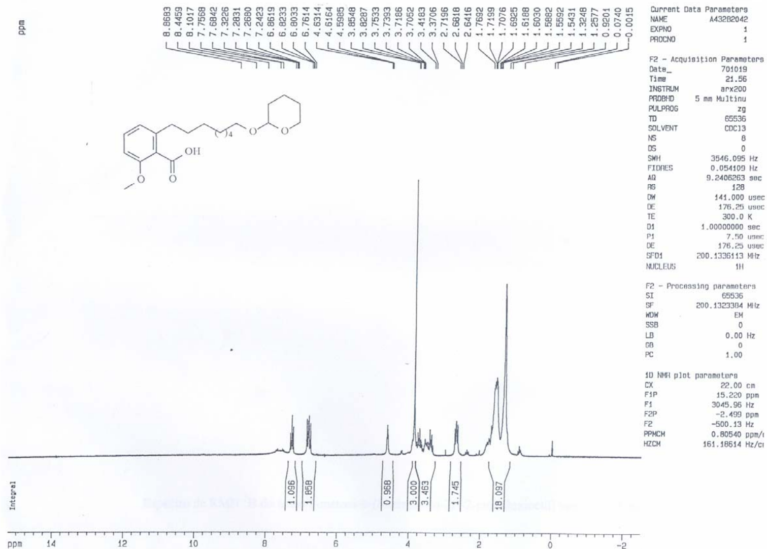
Espectro de RMN 1 H do ácido 2-metoxi-6-(8-tetraidro-2H-2-piraniloxioctil) benzóico (21b)
