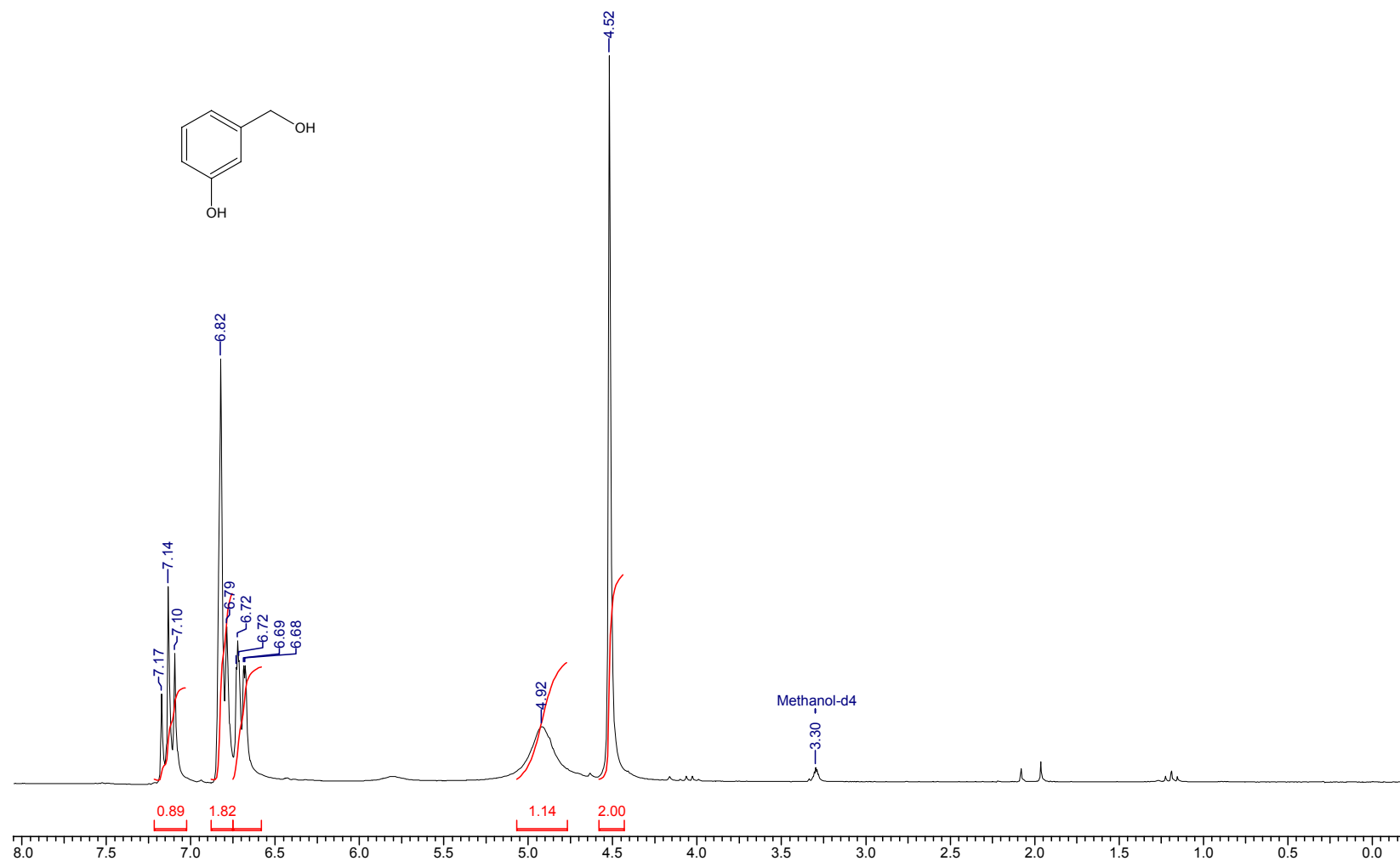
Espectro de RMN ^1\text{H} do 3-(hidroximetil)fenol (34)
