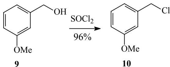
ESQUEMA 3.3 - Obtenção do 1-(clorometil)-3-metoxibenzeno ( 10 )
