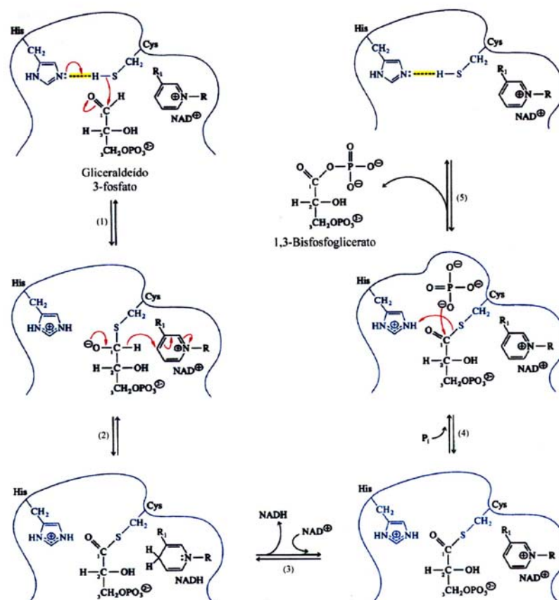
FIGURA 1.11 - Mecanismo da reação enzimática da gGAPDH (HORTON et al. , 1996). 1) Grupo sulfidrila da cisteína ionizada ataca o C1 do G3P, resultando na formação do hemitioacetil; 2) íon hidreto do complexo reduz o \text{NAD}^+ , formando o intermediário tioéster; 3) liberação do NADH e entrada de outra molécula de \text{NAD}^+ ; 4) fosfato inorgânico ataca o grupo carbonila do intermediário tioéster, formando o produto 1,3-bisfosfoglicerato; 5) dissociação do produto.
