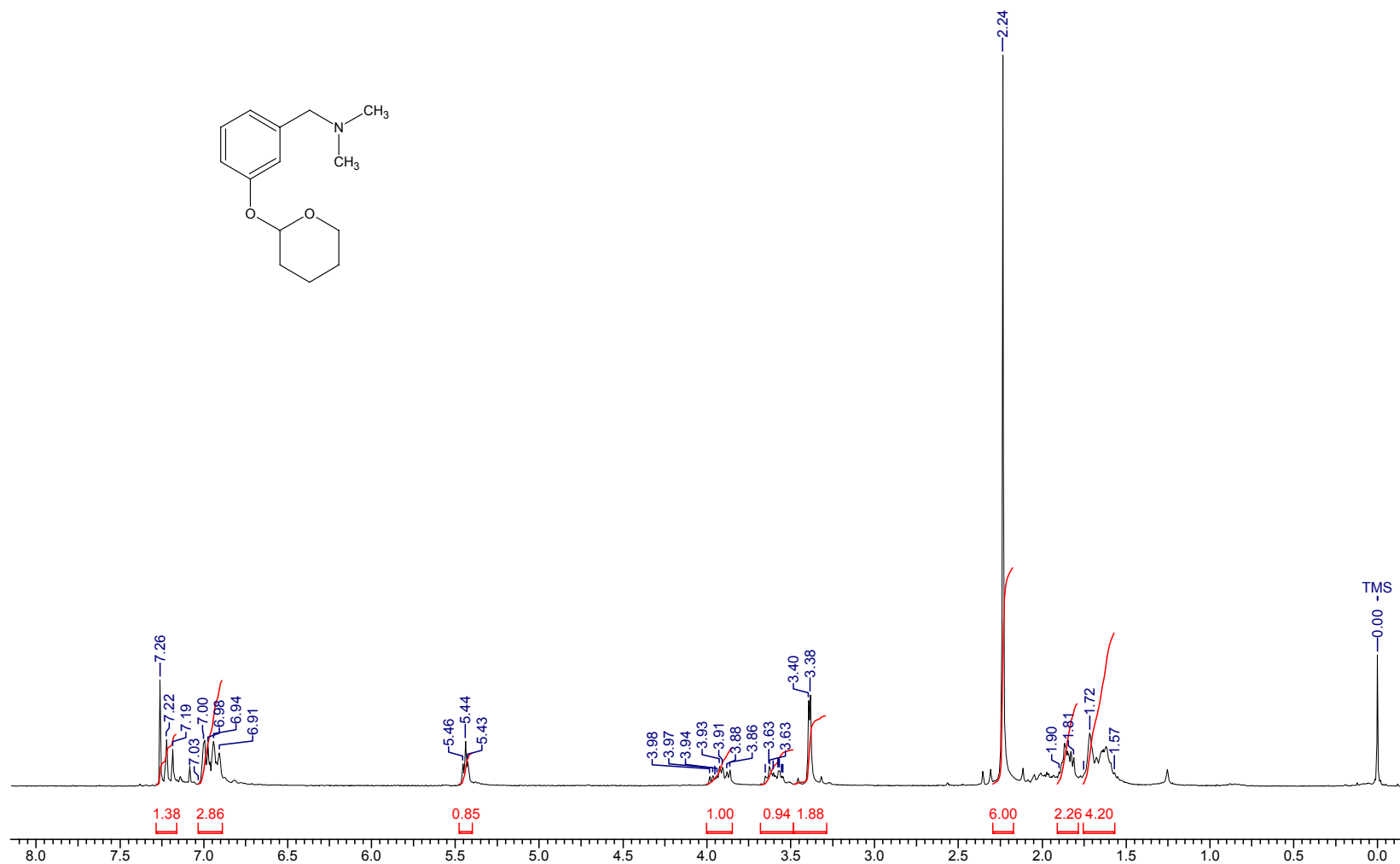
Espectro de RMN 1 H da N,N -dimetil-1-[3-(tetraidro-2 H -piran-2-iloxi)fenil]metanamina (37)
