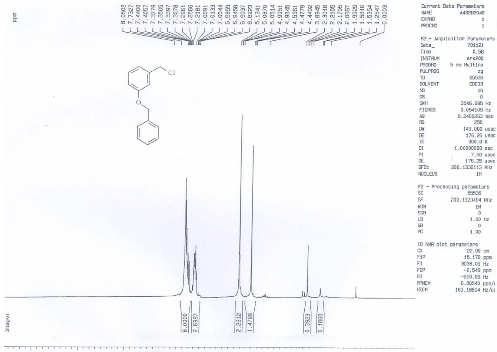
Espectro de RMN ^1\text{H} do 1-(benziloxy)-3-(clorometil)benzeno (30)
