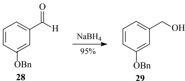
ESQUEMA 3.23 - Obtenção do [3-(benziloxi)fenil]metanol ( 29 )
