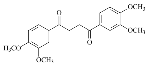
FIGURA 1.5 - Estrutura da 1,4-diaril-1,4-dicetona com atividade tripanocida
