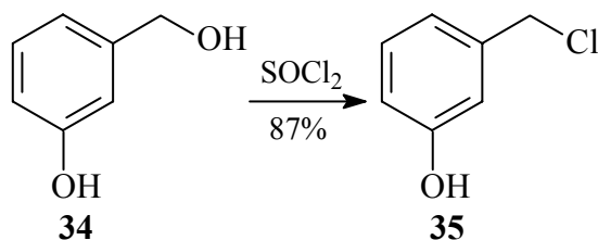
ESQUEMA 3.29 - Obtenção do 3-(clorometil)fenol ( 35 )
