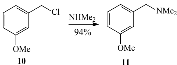
ESQUEMA 3.4 - Obtenção da 1-(3-metoxifenil)- N,N -dimetilmetanamina ( 11 )
