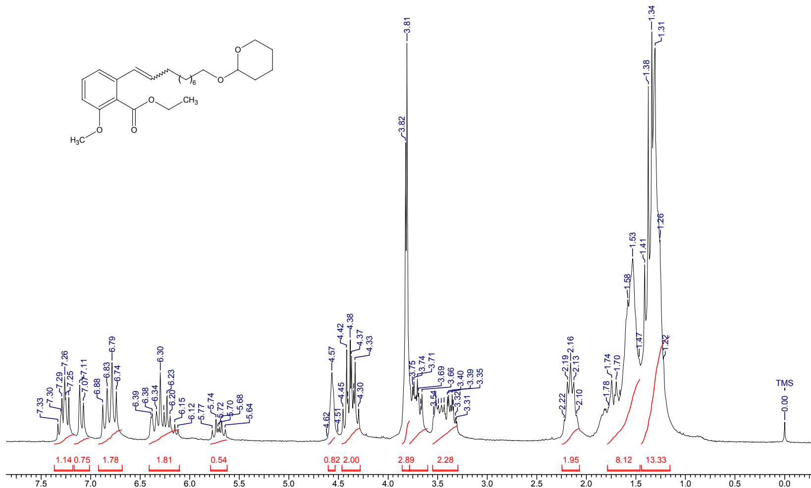
Espectro de RMN 1 H do 2-metoxi-6-[10-(tetraidro-piran-2-iloxi)-dec-1-enil]-benzoato de etila (19c)
