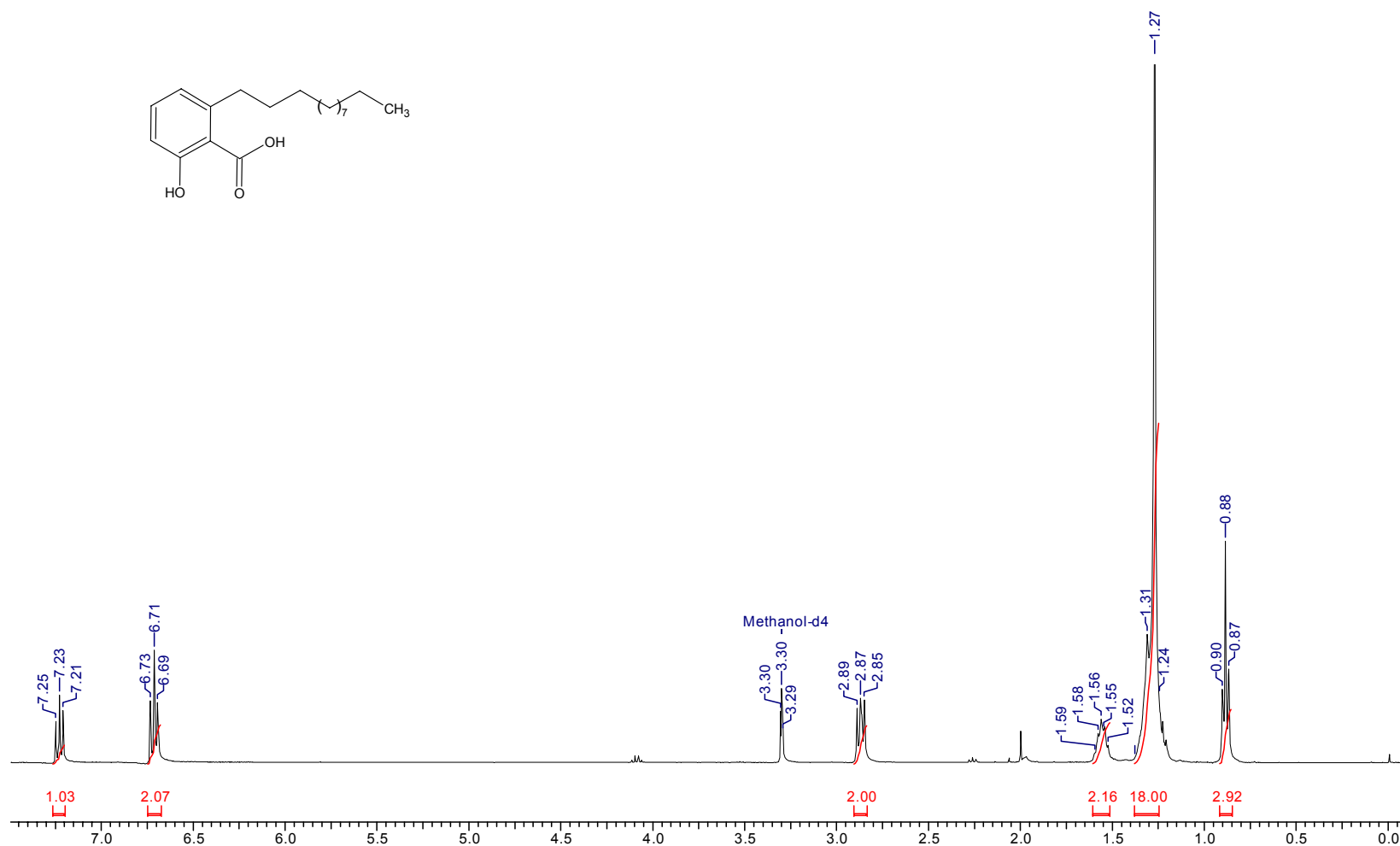
Espectro de RMN ^1\text{H} do ácido 2-dodecil-6-hidroxi-benzóico (24e)
