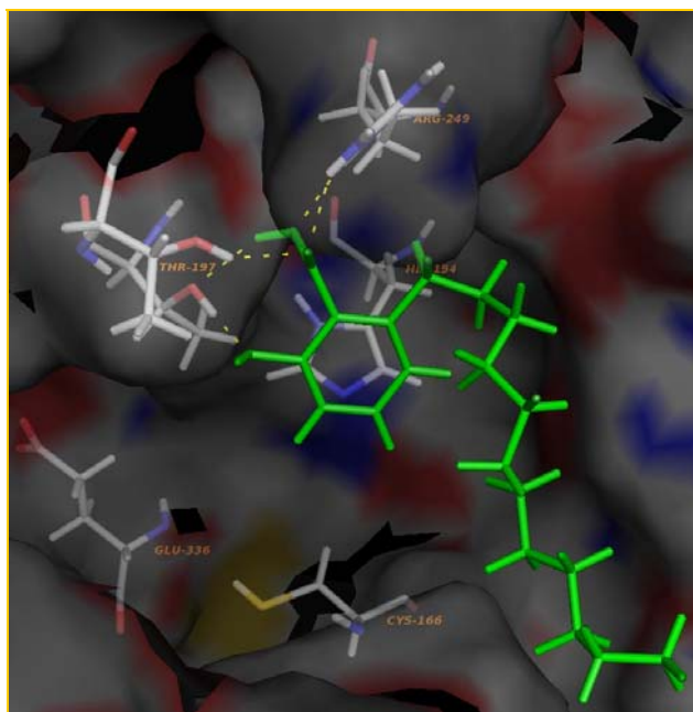
FIGURA 3.6 - Modelo de interação que melhor explica as possíveis interações entre o composto 24e e o sítio ativo da enzima gGAPDH.
