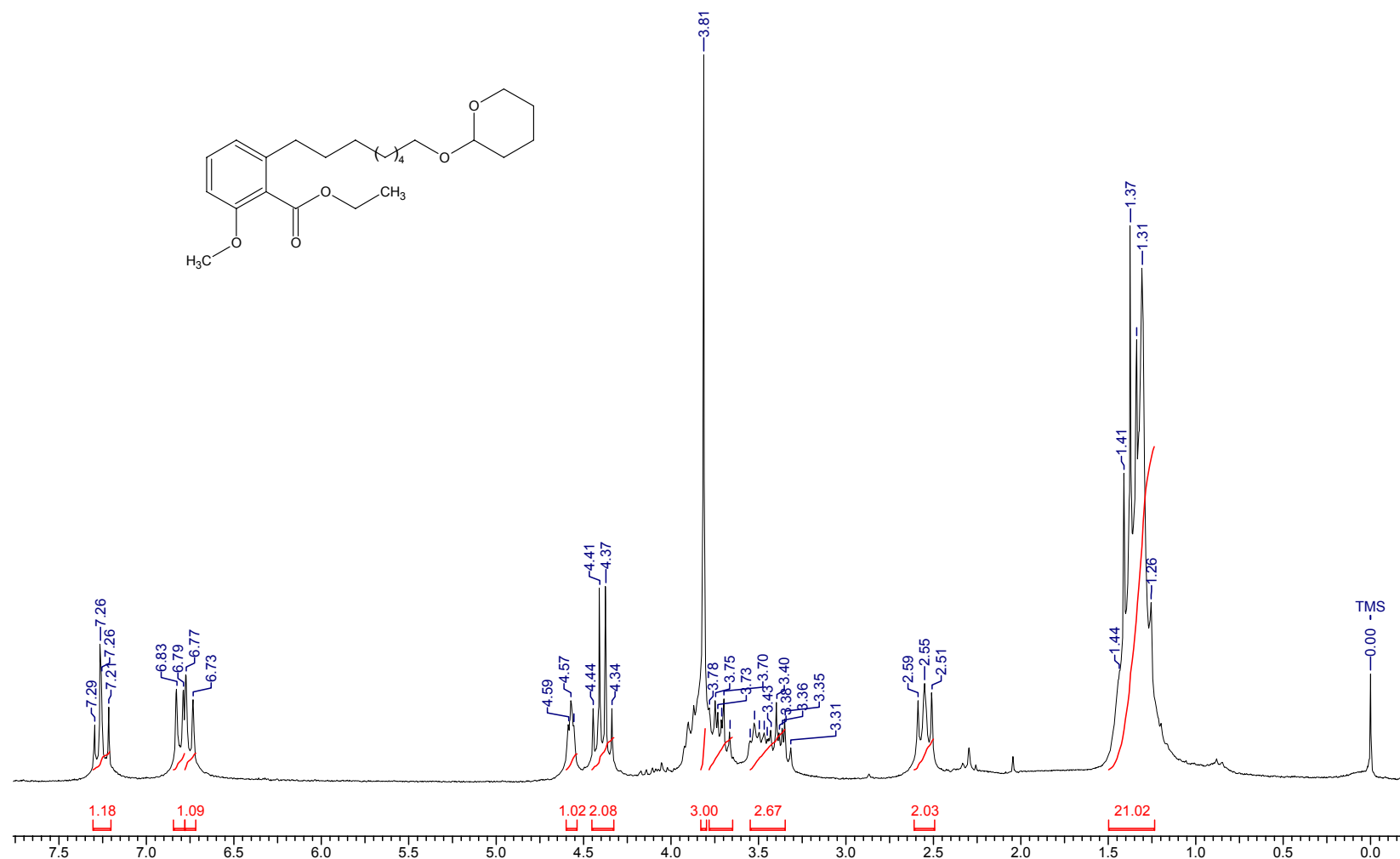
Espectro de RMN ^1\text{H} do 2-metoxi-6-[8-(tetraidro-piran-2-iloxi)-octil]-benzoato de etila ( 20b )
