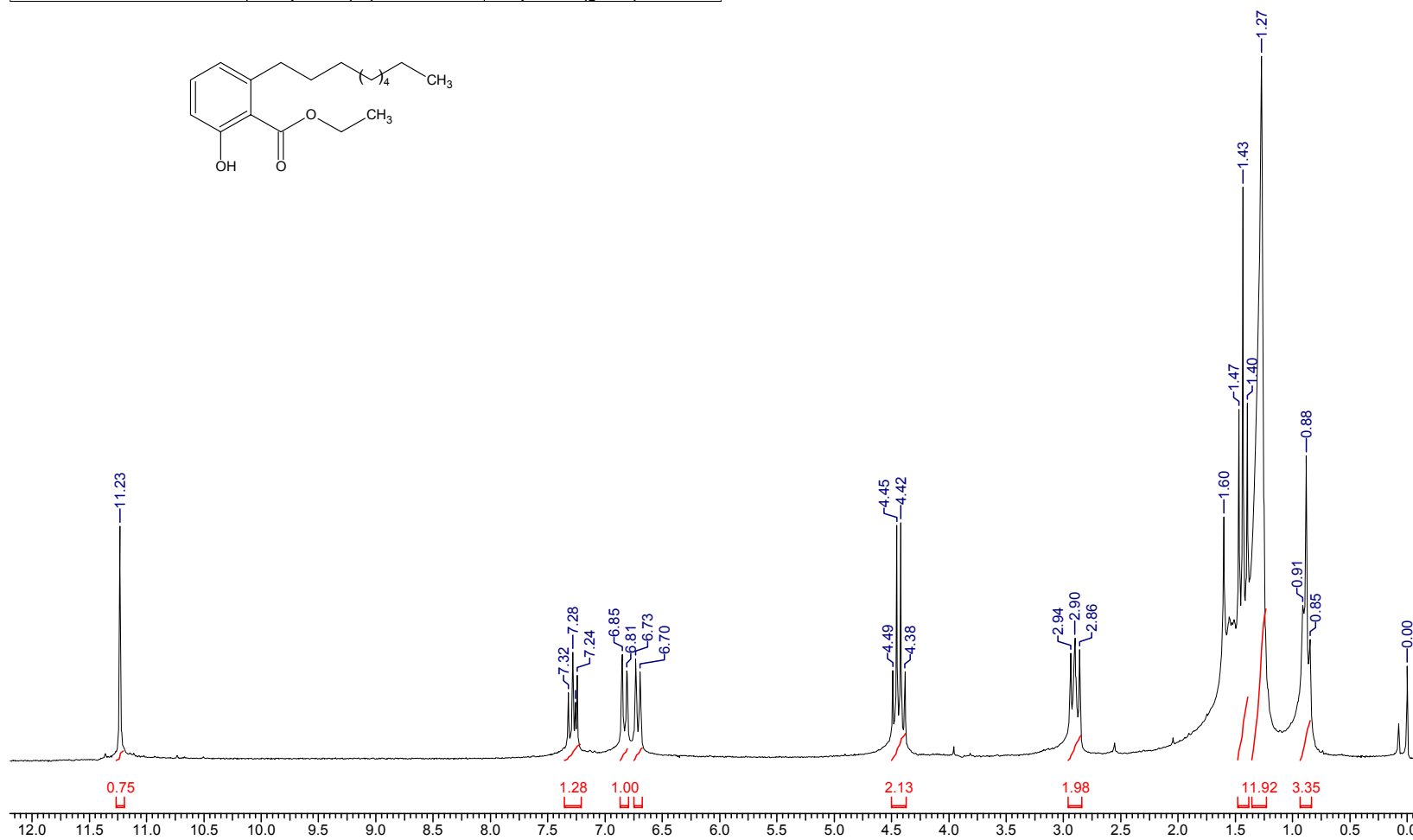
Espectro de RMN ^1\text{H} do 2-hidroxi-6-nonil-benzoato de etila ( 22d )
