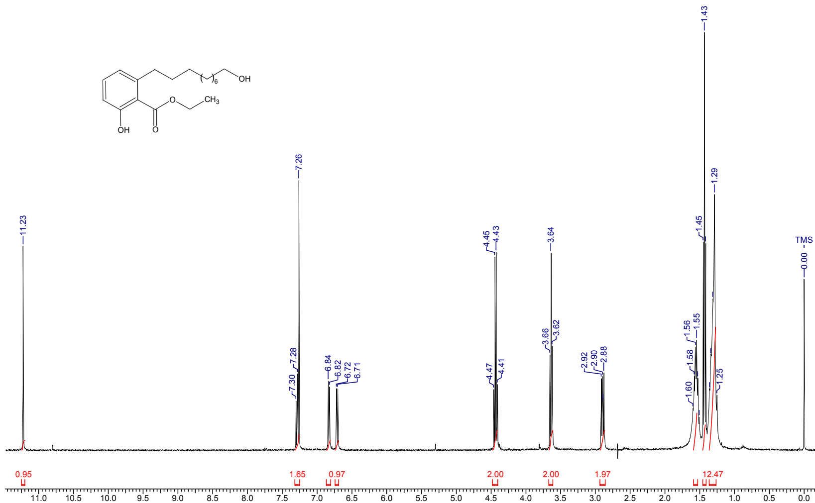
Espectro de RMN ^1\text{H} do 2-hidroxi-6-(10-hidroxi-decil)-benzoato de etila ( 22c )
