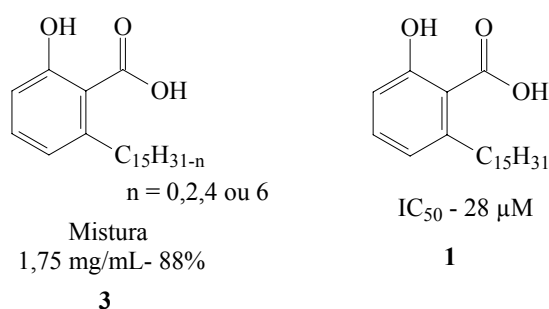
FIGURA 1.14 - Mistura de ácidos anacárdicos ( 3 ) e ácido anacárdico hidrogenado ( 1 )
