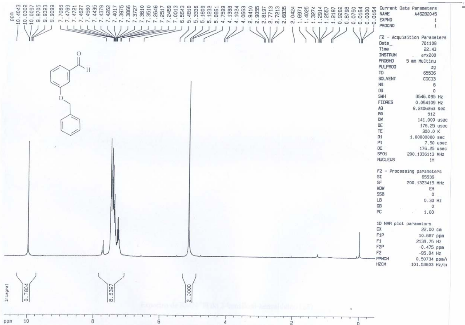
Espectro de RMN ^1\text{H} do 3-(benziloxi)-benzaléido (28)
