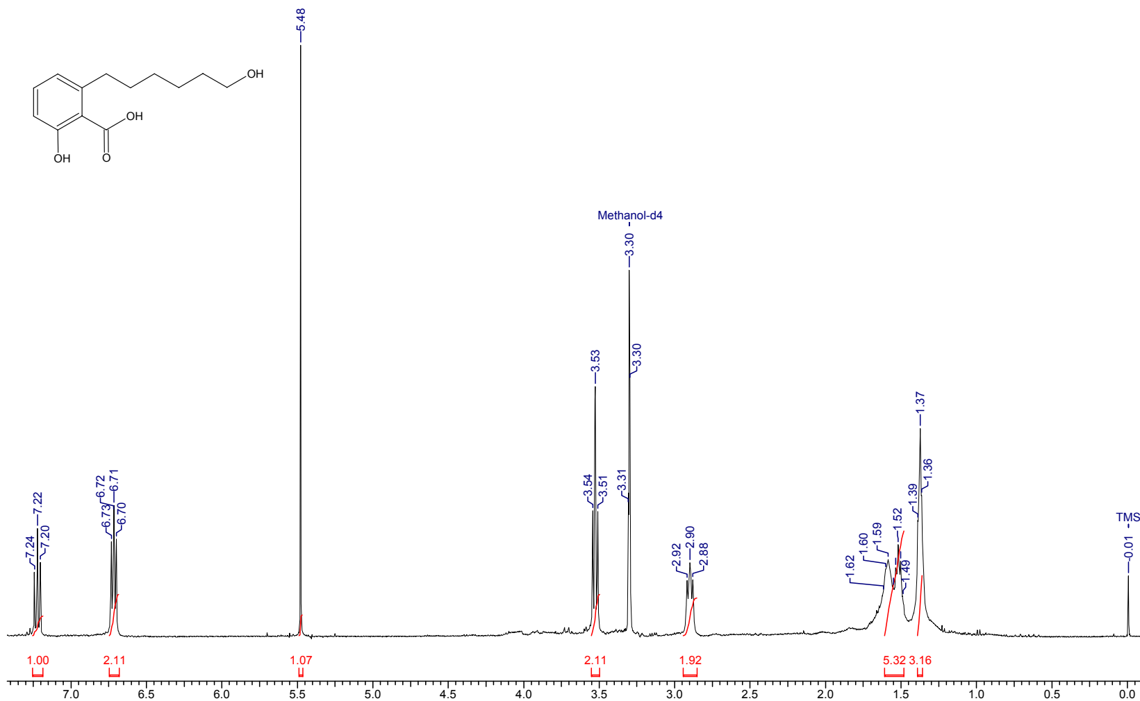
Espectro de RMN ^1\text{H} do ácido 2-hidroxi-6-(6-hidroxi-hexil)-benzóico (24a)
