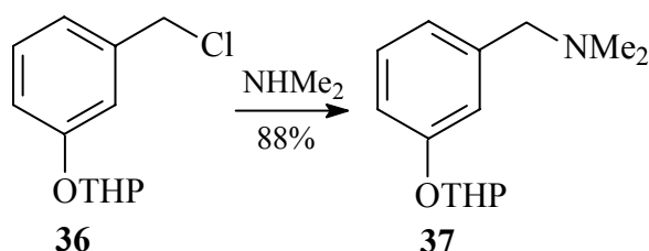
ESQUEMA 3.31- Obtenção da N,N-dimetil-1-[3-(tetraidro-2H-piran-2-iloxi)fenil]metanamina ( 37 )
