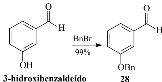
ESQUEMA 3.22 - Obtenção do 3-(benziloxi)-benzaldeído (28)
