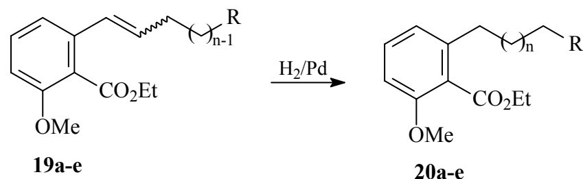
ESQUEMA 3.10 - Obtenção dos compostos 20a-e
