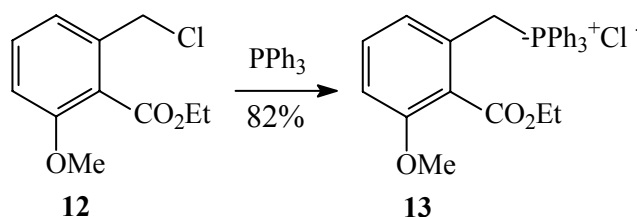
ESQUEMA 3.6 - Obtenção do cloreto de 2-(etoxicarbonil)-3-(metoxibenzil)trifenilfosfônio ( 13 )
