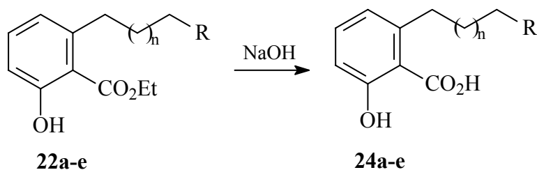
ESQUEMA 3.15 - Obtenção dos compostos 24a-e
