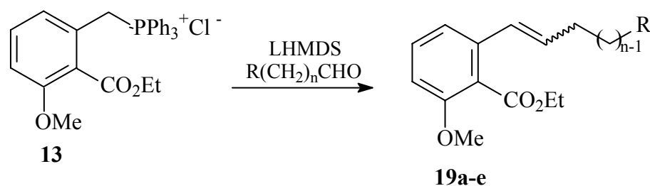
ESQUEMA 3.8 - Obtenção dos compostos 19a-e
