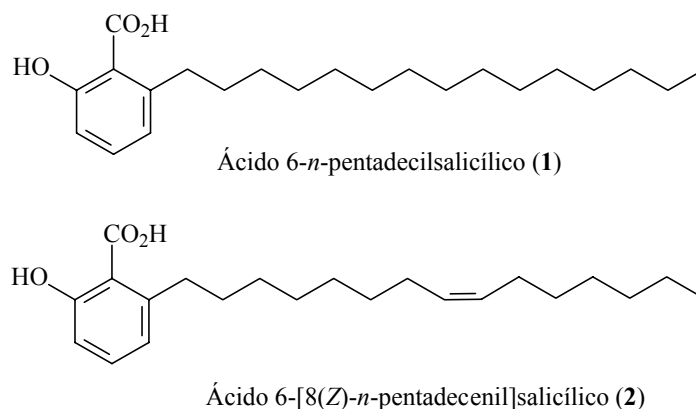
FIGURA 1.13 - Exemplos de ácidos anacárdicos
