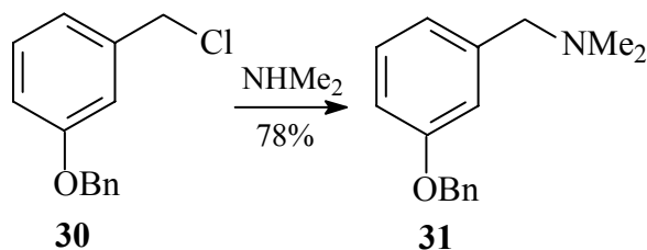
ESQUEMA 3.25 - Obtenção da 1-[3-(benziloxi)fenil]- N,N -dimetilmetanamina ( 31 )
