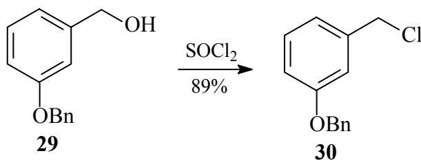
ESQUEMA 3.24 - Obtenção do 1-(benziloxi)-3-(clorometil)benzeno ( 30 )
