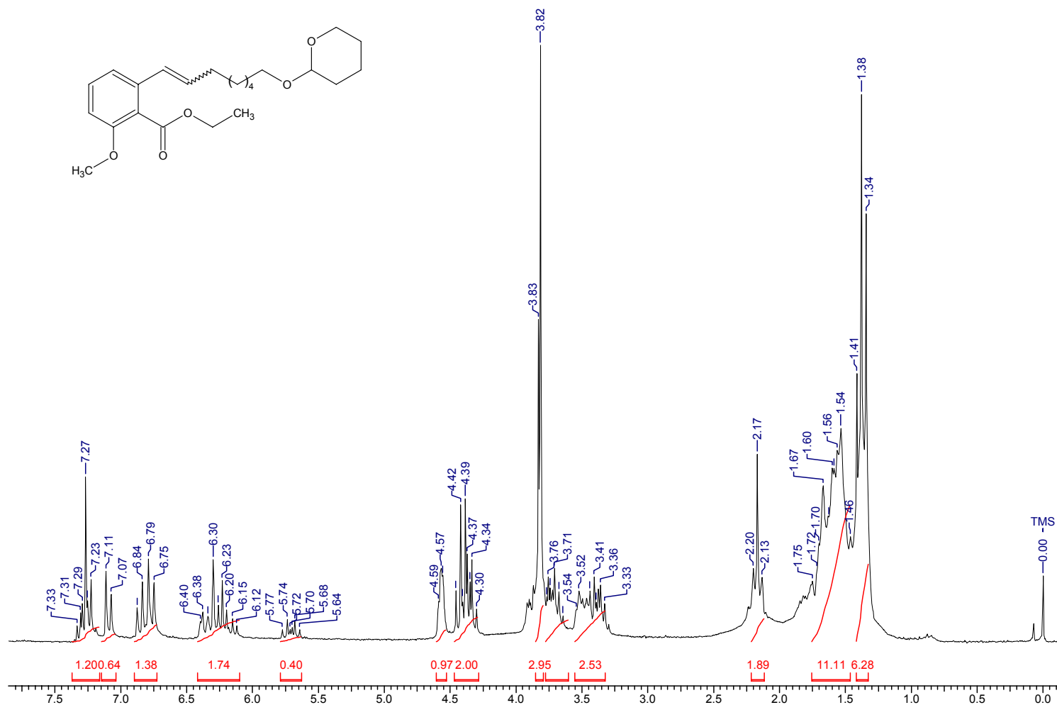
Espectro de RMN ^1\text{H} do 2-metoxi-6-[8-(tetraidro-piran-2-iloxi)-oct-1-enil]-benzoato de etila (19b)
