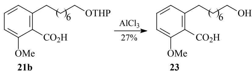
ESQUEMA 3.13 - Obtenção do ácido 2-(8-hidroxiocetil)-6-metoxibenzóico ( 23 )
