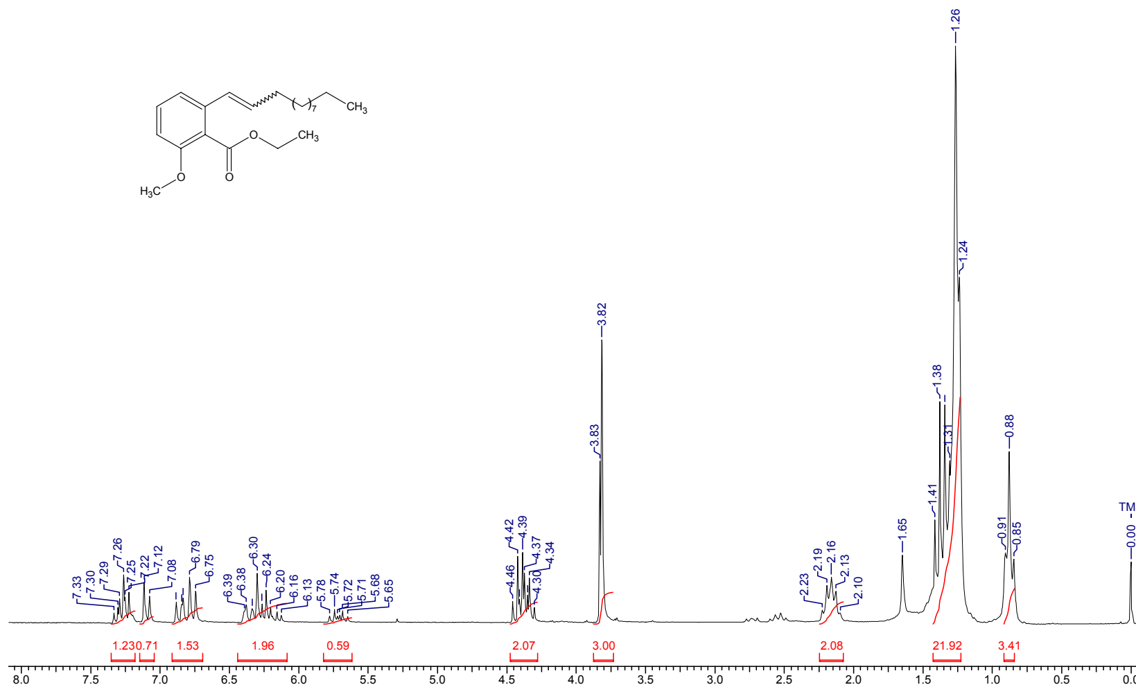
Espectro de RMN 1 H do 2-dodec-1-enil-6-metoxi-benzoato de etila (19e)
