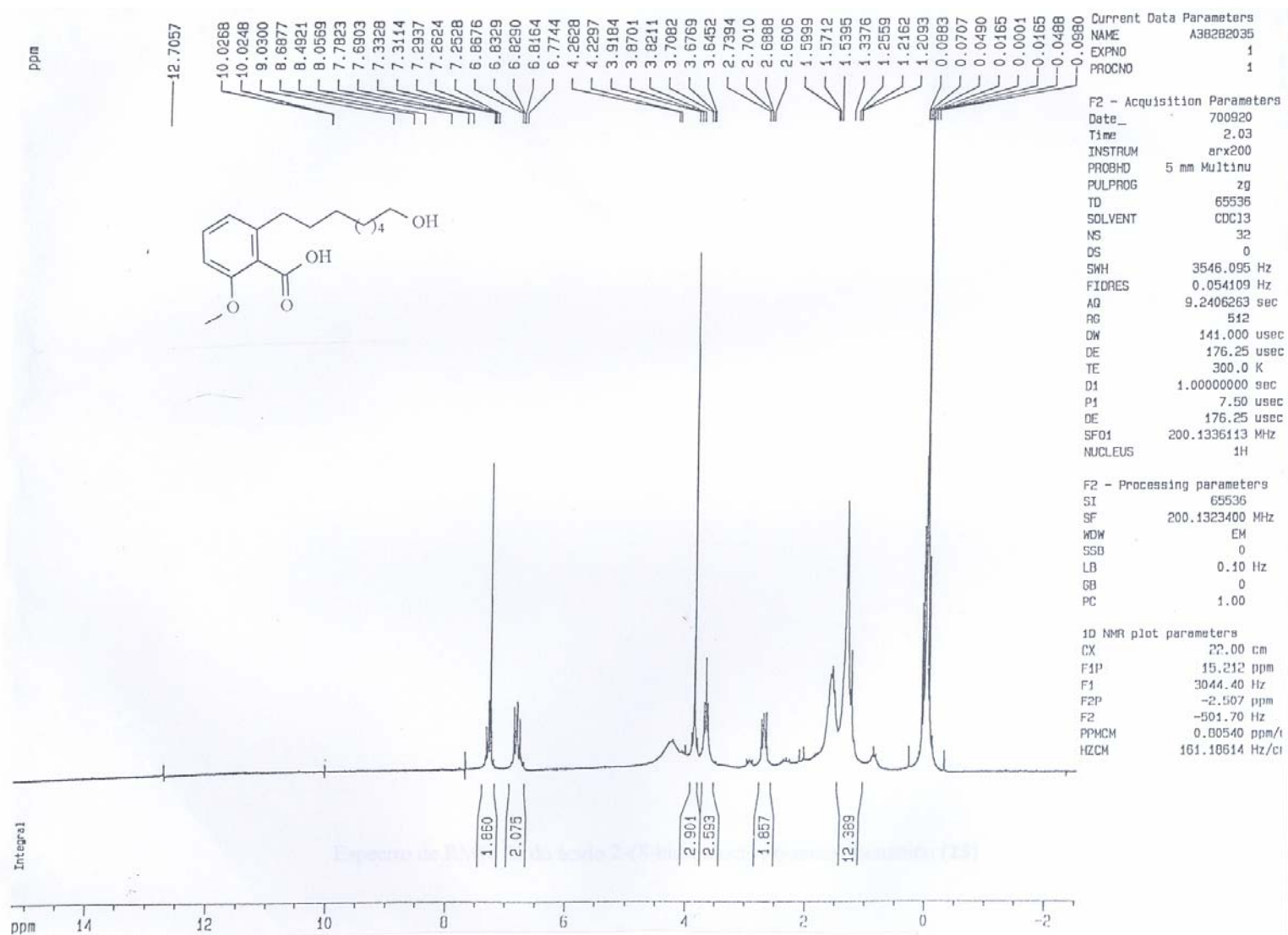
Espectro de RMN ^1\text{H} do ácido 2-(8-hidroxiocetil)-6-metoxibenzóico (23)
