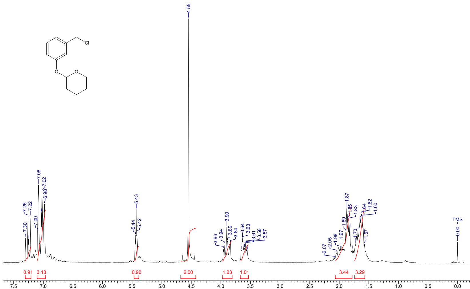
Espectro de RMN 1 H do 2-[3-(clorometil)fenoxi]tetraidro-2H-pirano (36)
