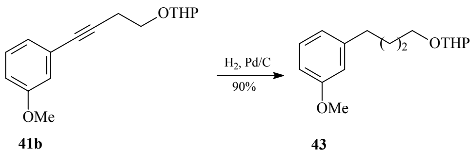
ESQUEMA 3.37 - Obtenção do 2-[4-(3-metoxifenil)butoxi]tetraidro-2H-pirano ( 43 ).
