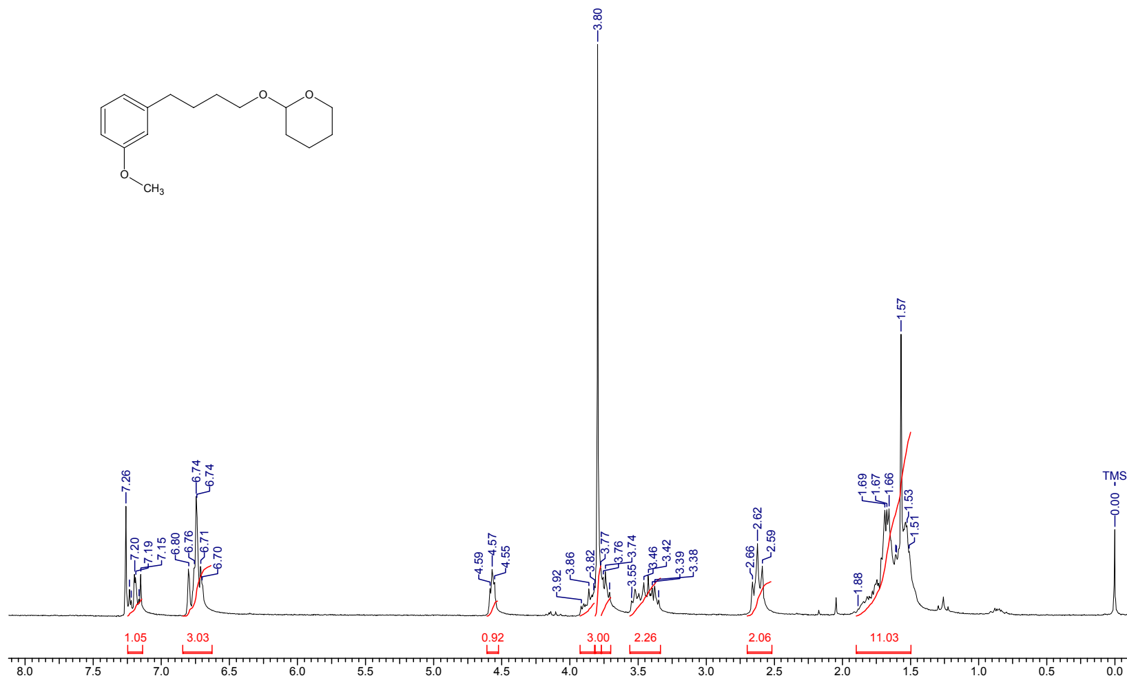
Espectro de RMN 1 H do 2-[4-(3-metoxifenil)butoxi]tetraidro-2H-pirano (43)
