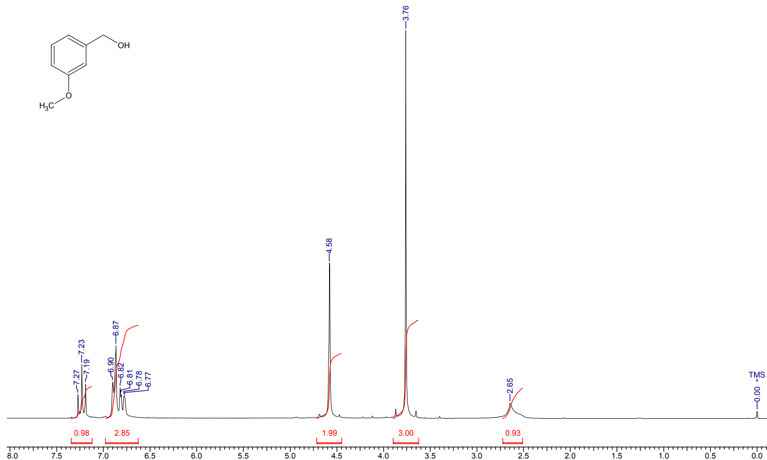
Espectro de RMN 1 H do (3-metoxifenil)metanol (9)
