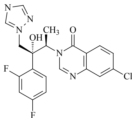
FIGURA 1.6 - Estrutura química do albaconazol
