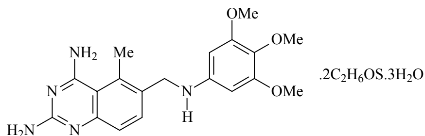
FIGURA 1.9 - Estrutura química do timetrexato antifolato lipofílico (TMQ)
