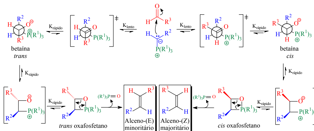
ESQUEMA 3.9 - Mecanismo para a reação de Wittig.
