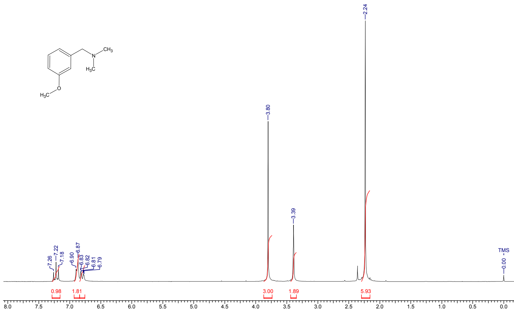
Espectro de RMN 1 H da 1-(3-metoxifenil)-N,N-dimetilmetanamina ( 11 )
