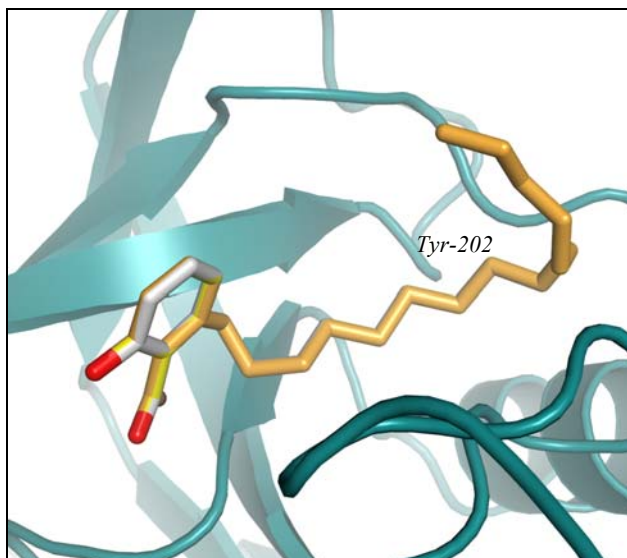
FIGURA 3.9 - Sobreposição dos modelos gerados para os compostos 1 (laranja), 24d (cinza) e 24e (amarelo) no sítio ativo da enzima PNP.
