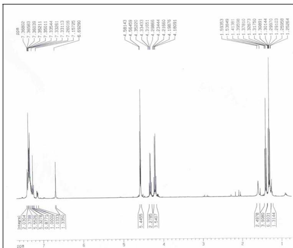
FIGURA 3.1- Espectro de RMN 1 H do composto 33
