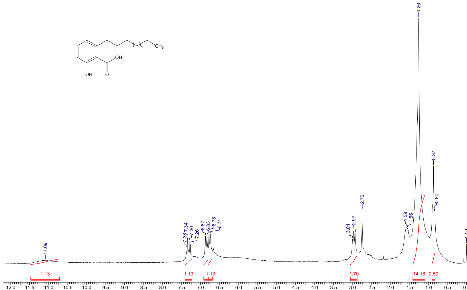
Espectro de RMN ^1\text{H} do ácido 2-hidroxi-6-nonil-benzóico ( 24d )
