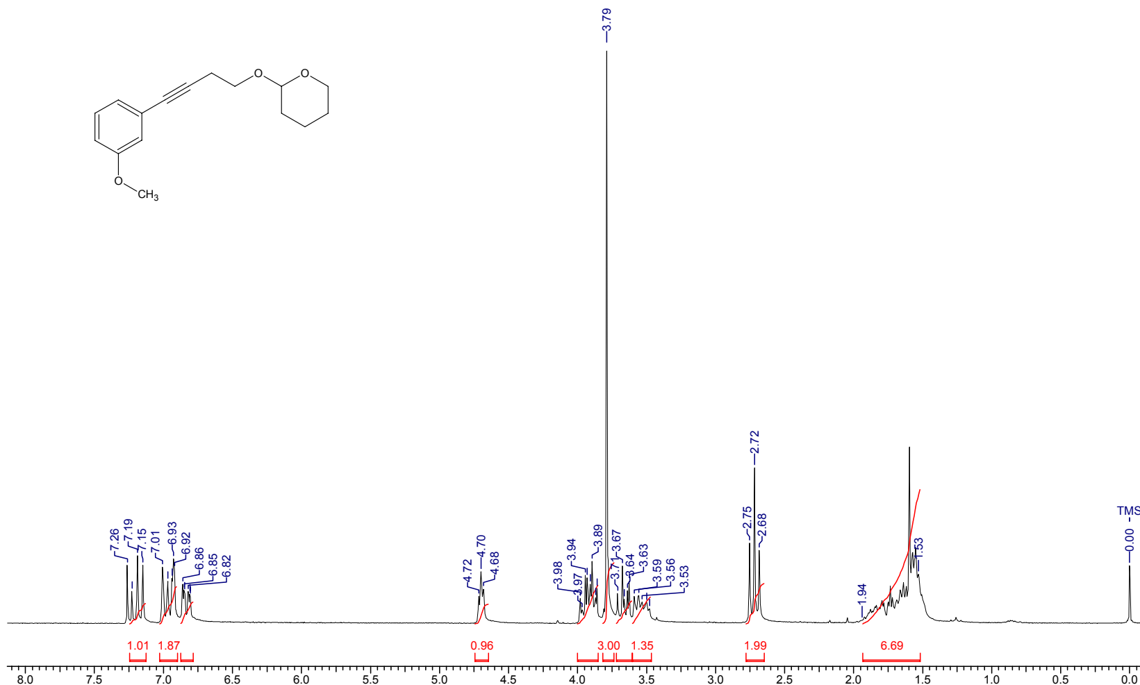
Espectro de RMN 1 H do 2-[4-(3-metoxi-fenil)-3-butini-oxi]-tetraidropirano ( 41b )
