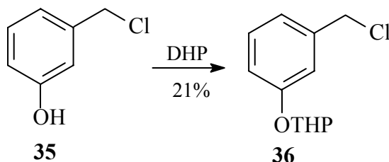
ESQUEMA 3.30- Obtenção do 2-[3-(clorometil)fenoxi]tetraidro-2 H -pirano ( 36 )
