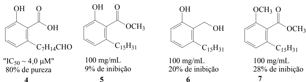
FIGURA 1.16 - Derivados de ácidos anacárdicos.
