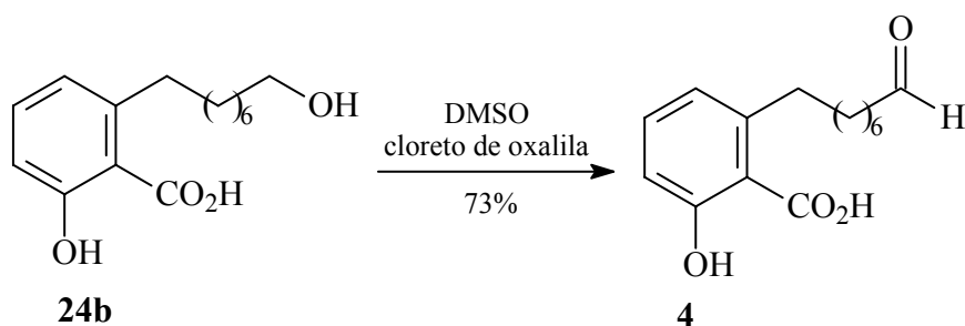
ESQUEMA 3.16 - Obtenção do ácido 2-hidroxi-6-(8-oxooctil) benzóico ( 4 )
