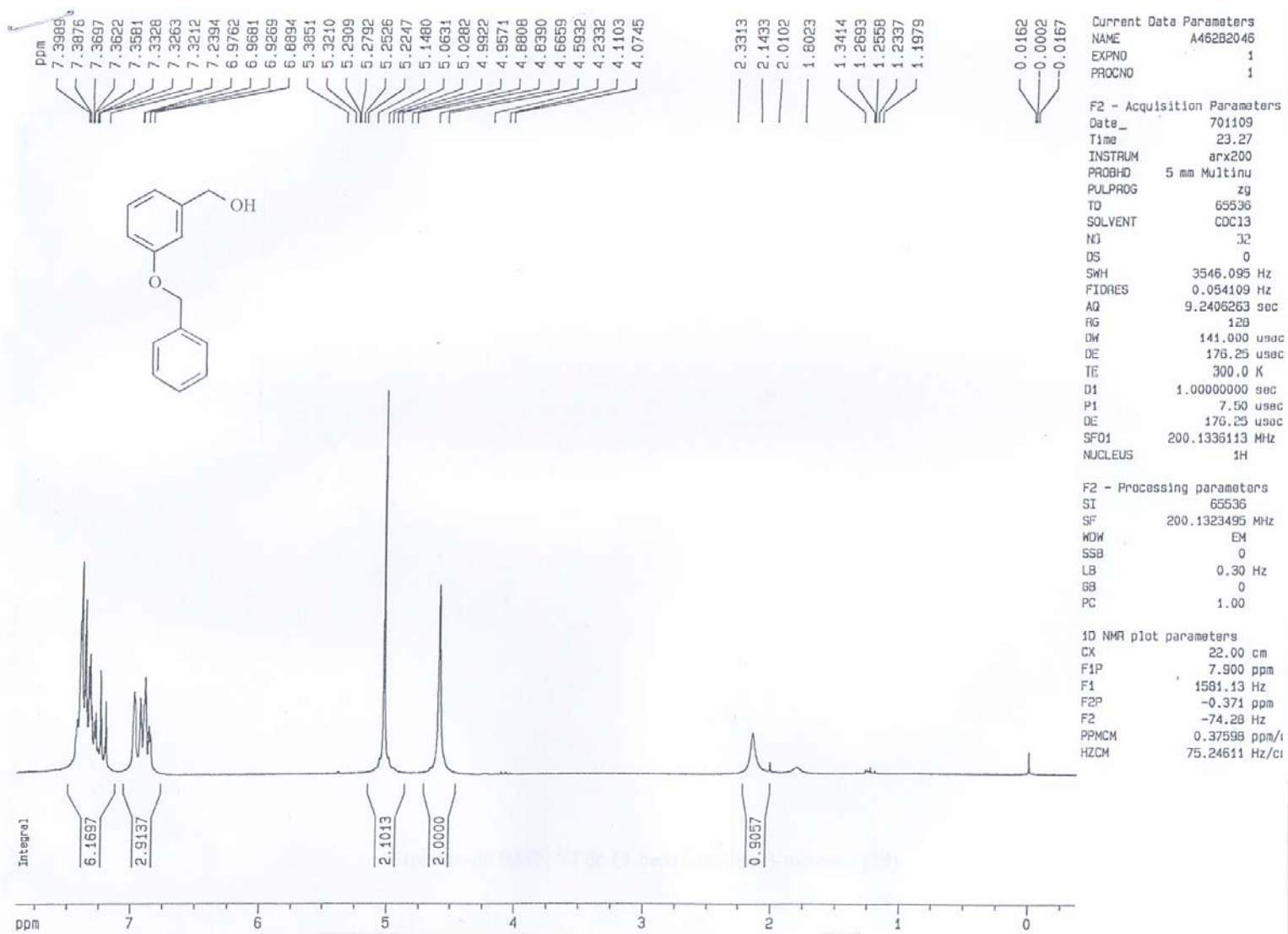
Espectro de RMN ^1\text{H} do [3-(benziloxi)fenil]metanol (29)
