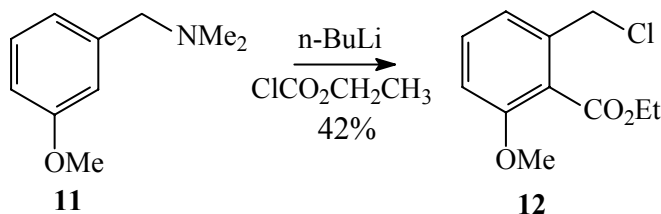
ESQUEMA 3.5 - Obtenção do 2-(clorometil)-6-metoxibenzoato de etila ( 12 )
