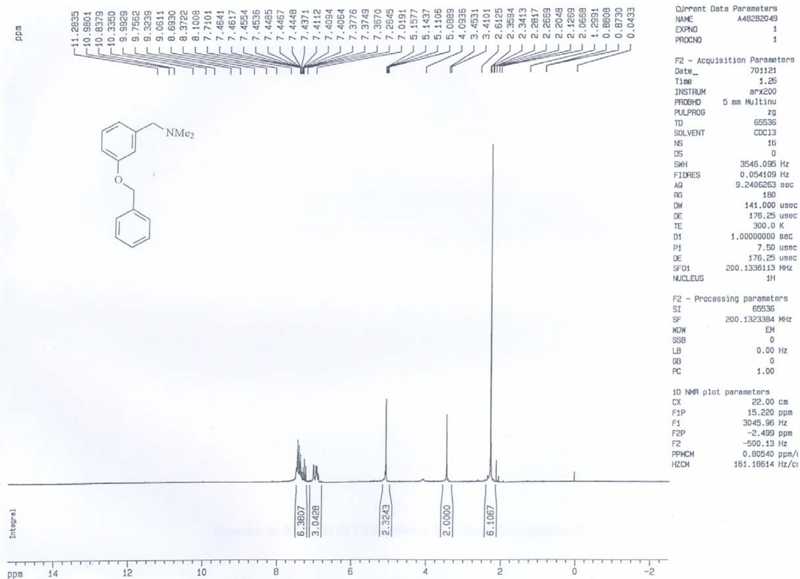
Espectro de RMN ^1\text{H} da 1-[3-(benziloxy)fenil]-N,N-dimetilmetanamina (31)
