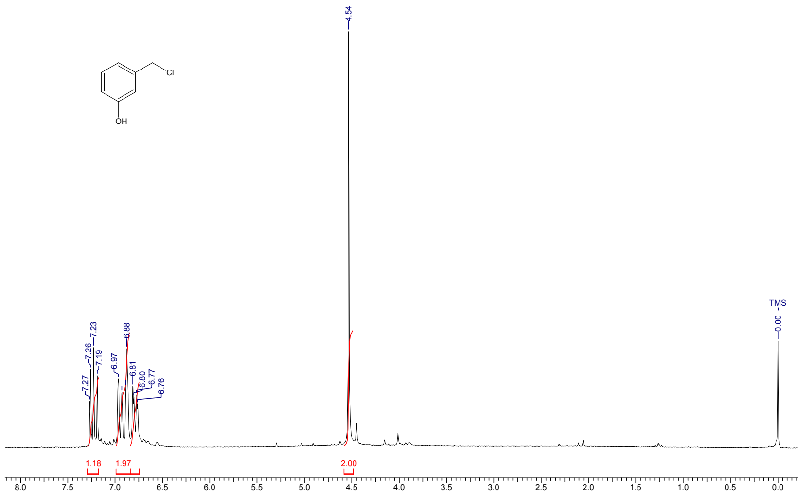
Espectro de RMN ^1\text{H} do 3-(clorometil)fenol (35)
