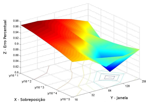
FIGURA 27: Erro Percentual Apresentado pela Rede Neural Sem Wavelets
