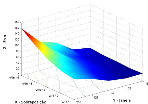
FIGURA 38: Erro Quadrático Médio – Redes Neurais – Wavelet Chma6 – Terceira Decomposição
