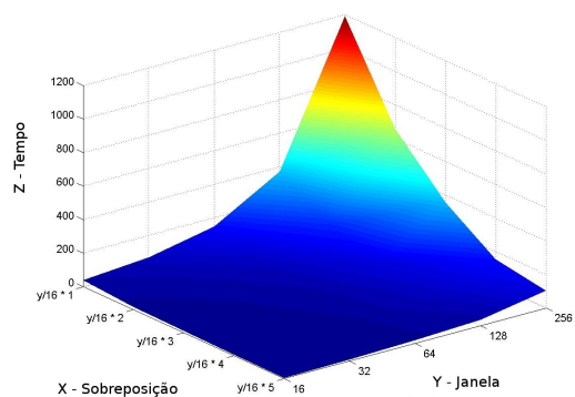
FIGURA 28: Tempo Médio (segundos) para Execução do Experimento
