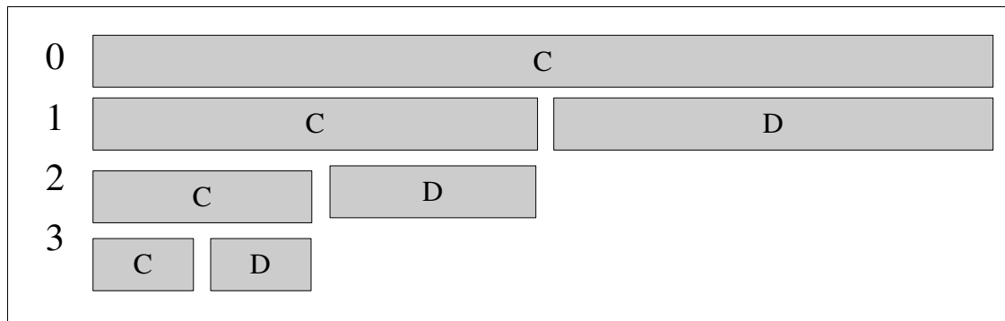
FIGURA 4: Decomposição de um sinal em várias escalas
