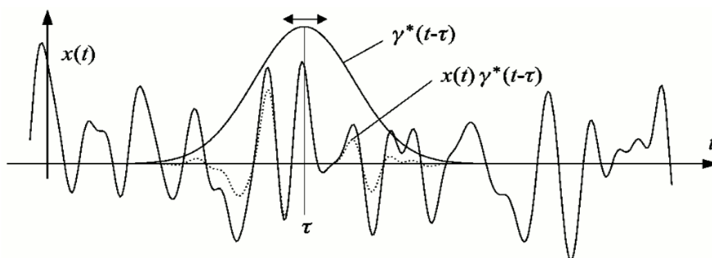
FIGURA 3: Transformada Breve de Fourier (utilizando função Gaussiana) Fonte: MERTINS 1999, p. 197
