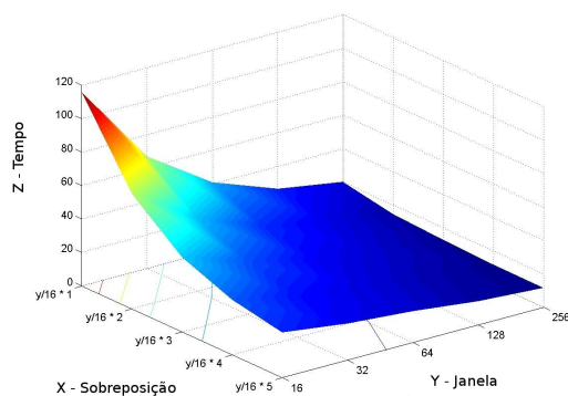
FIGURA 40: Tempo Médio (segundos) para Execução do Experimento
