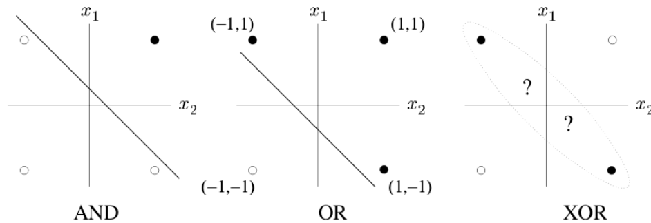
FIGURA 14: Representação geométrica do espaço de entrada Fonte: KRÖSE & VAN DER SMAGT (1996, p. 29)
