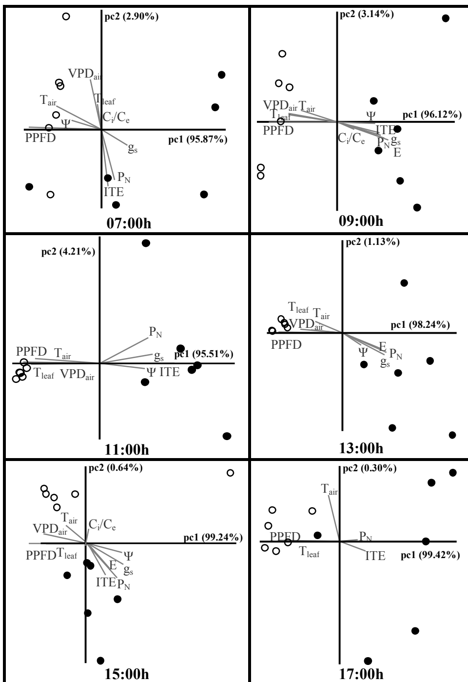
Figura 6. Análise dos componentes principais das trocas gasosas foliares e potencial hídrico foliar ( \Psi ) obtidos durante cursos diurnos em três cultivares de Coffea arabica . Cada painel representa um horário do dia. Dias claro e nublado estão representados por símbolos abertos (○) e sólidos (●), respectivamente. Cada símbolo indica um cultivar independente do tratamento (franco e enxertado). Os vetores (linhas retas de cor cinza) representam os parâmetros ambientais ou fisiológicos mais importantes. PPFD = densidade do fluxo de fótons fotossintéticos, T_{air} = temperatura do ar, VPD_{air} = déficit de pressão de vapor do ar, T_{leaf} = temperatura foliar, P_N = fotossíntese líquida, g_s = condutância estomática ao vapor d'água, E = transpiração foliar, ITE = eficiência instantânea da transpiração e C_i/C_e = concentração CO_2 intercelular ( C_i ) por externa ( C_e ) de CO_2 .
