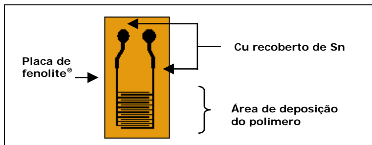
Figura 7.3.2: Esquema do sensor de gases.
