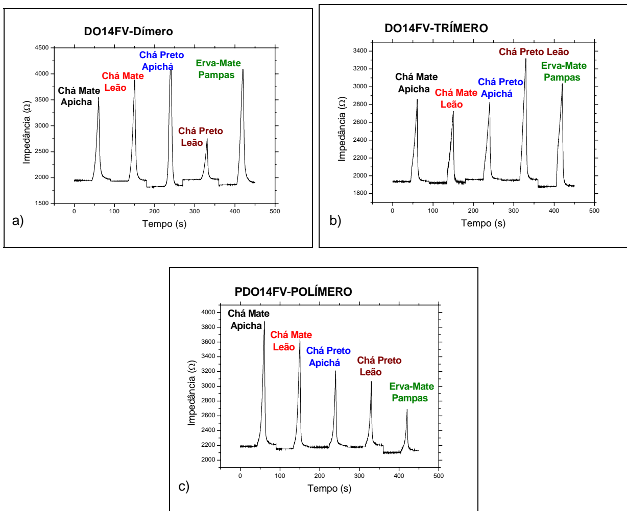
Figura 5.3.1: Gráficos de resposta ao longo do tempo: a) DO14FV-dímero, b) DO14FV-trímero e c) PDO14FV-polímero.
