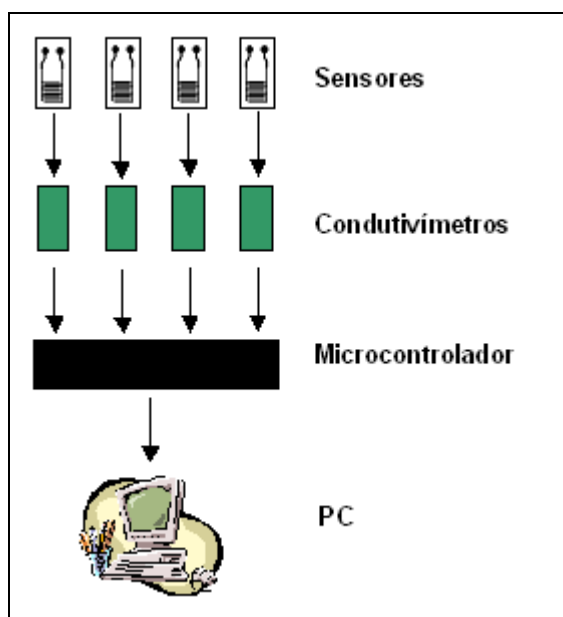
Figura 7.3.1: Esquema do equipamento utilizado na aquisição dos dados.
