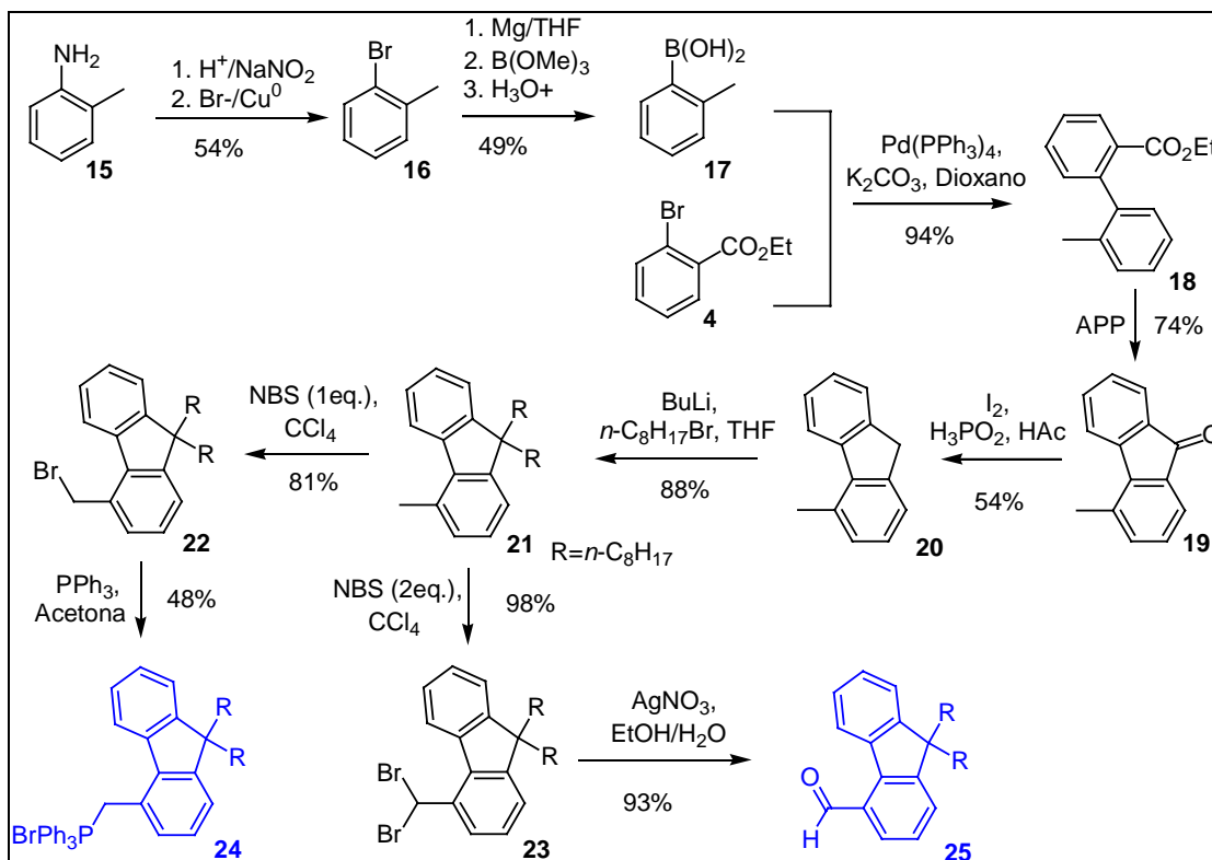
Esquema 5.1.15: Rota sintética para a preparação do sal de foscônio 24 e do aldeído 25 .
