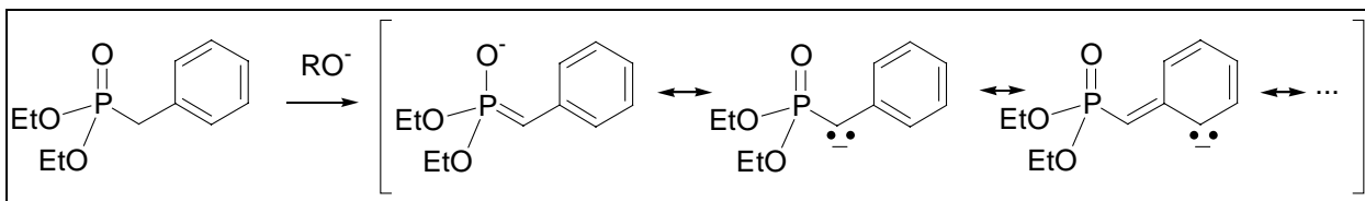
Esquema 1.7: Mecanismo de estabilização da ílida.
