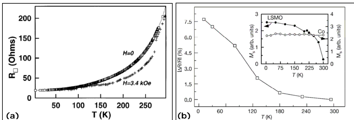
Figura 2.5: (a) Curva para T 6 13 ; (b) Curva para Alq 3 15 .
