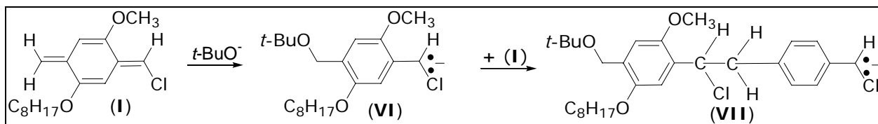
Esquema 1.3: Mecanismo aniônico da reação de Gilch.
