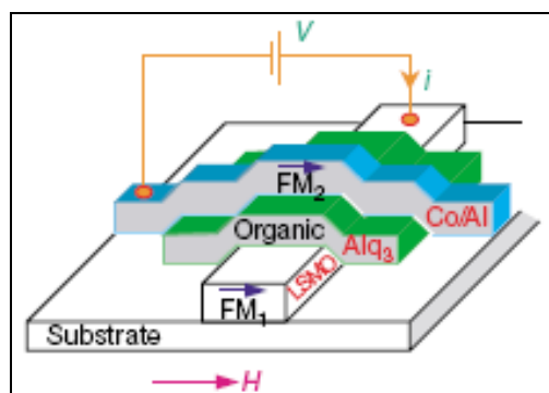
Figura 2.4: Esquema da válvula de spin contendo LSMO/ \text{Alq}_3 /Co 15 .
