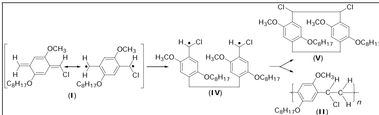
Esquema 1.2: Mecanismo radicalar da reação de Gilch.
