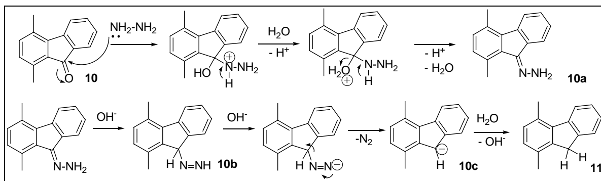
Esquema 5.1.9: Mecanismo da reação de preparação do composto 11 por Wolff-Kishner.
