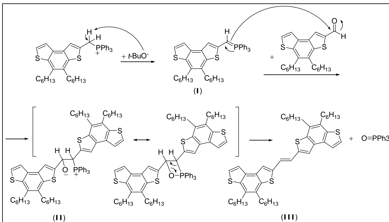
Esquema 1.6: Mecanismo da reação de Wittig.
