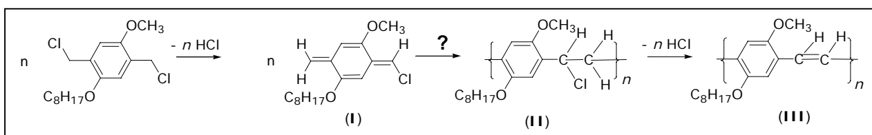
Esquema 1.1: Mecanismo da reação de Gilch.
