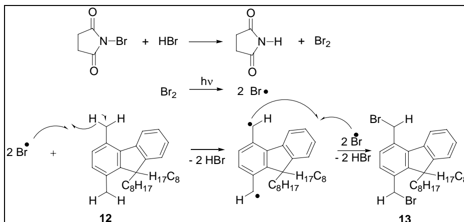
Esquema 5.1.13: Mecanismo da reação de preparação do composto 13 .
