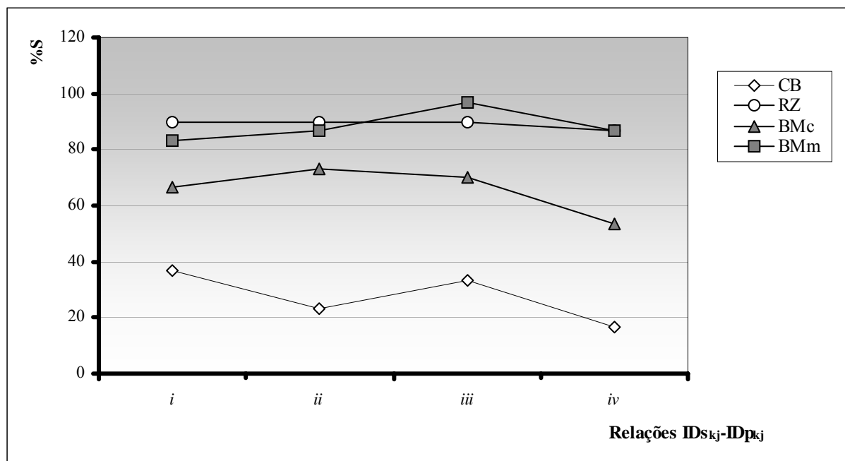
Gráfico 5.39. Porcentagem de sucesso para n = 20 e m = 20
