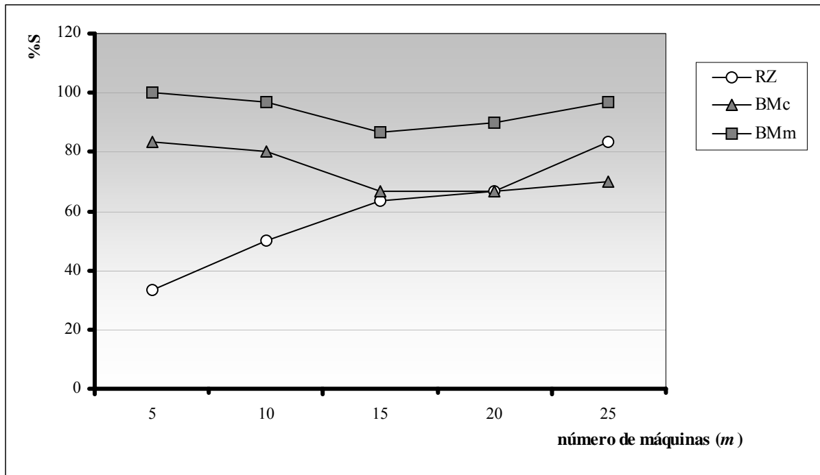
Gráfico 5.42. Porcentagem de sucesso para n = 40 – Relação i
