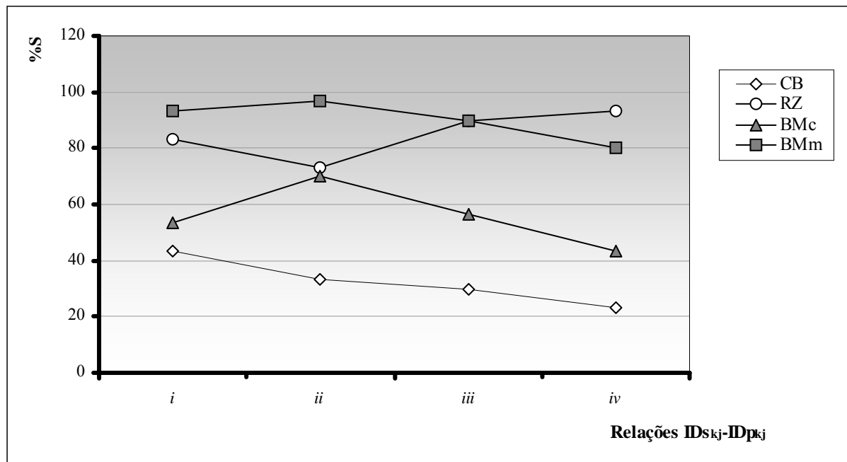
Gráfico 5.38. Porcentagem de sucesso para n = 20 e m = 15
