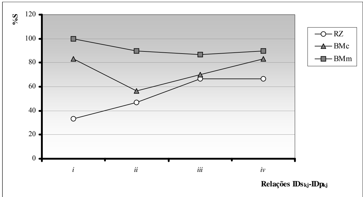
Gráfico 5.46. Porcentagem de sucesso para n = 40 e m = 5
