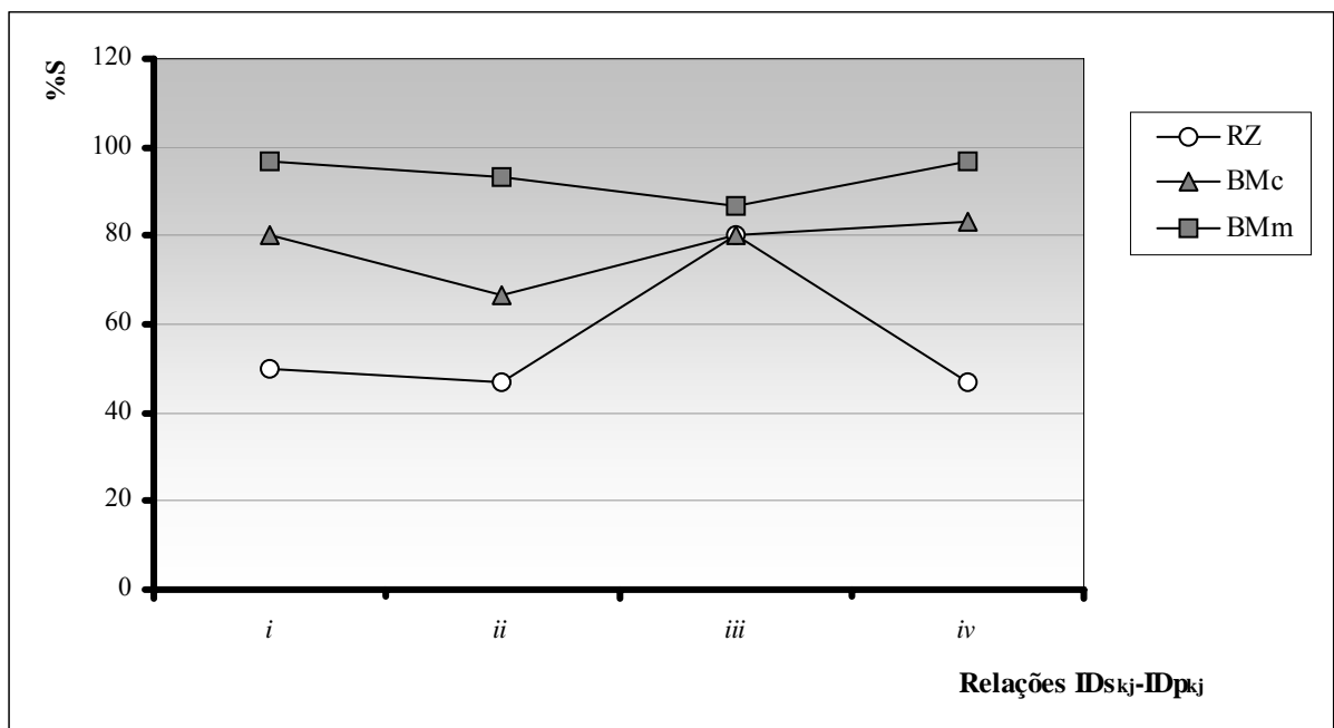
Gráfico 5.47. Porcentagem de sucesso para n = 40 e m = 10
