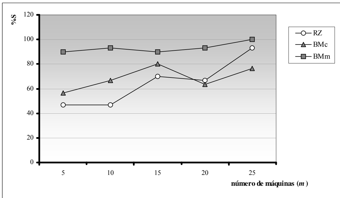
Gráfico 5.43. Porcentagem de sucesso para n = 40 – Relação ii
