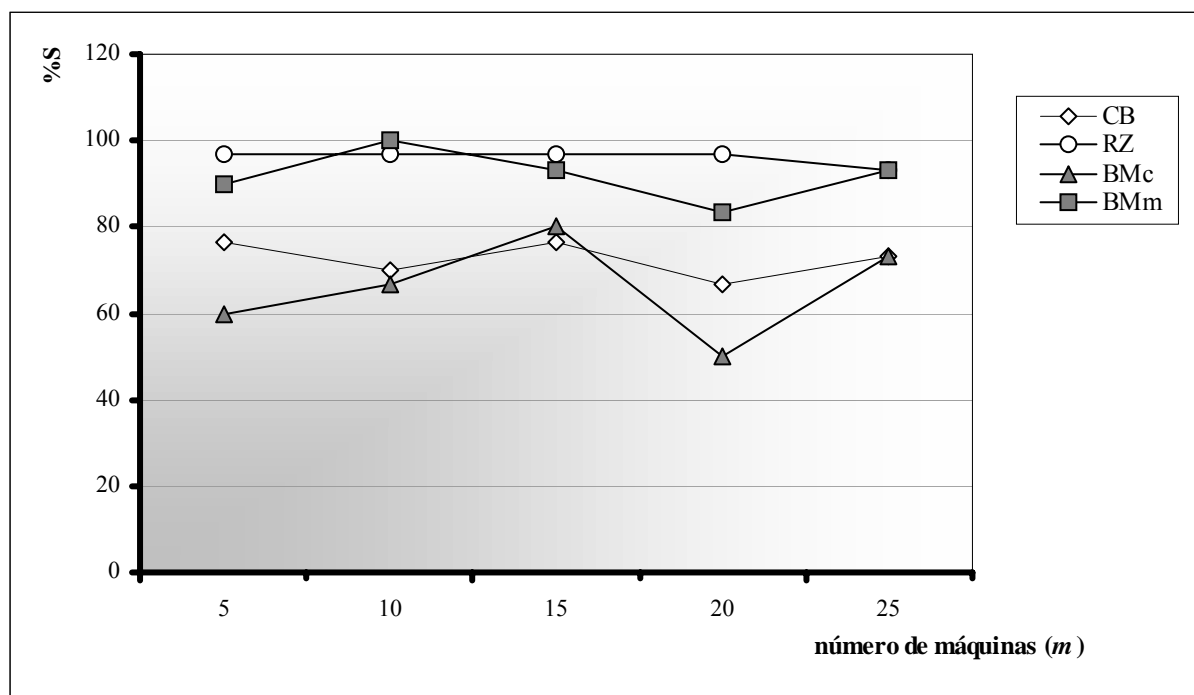
Gráfico 5.2. Porcentagem de sucesso para n = 4 – Relação ii
