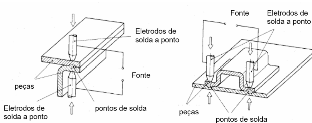
Figura 12 – Junção por solda a ponto dos dois lados e de um dos lados
