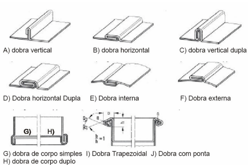
Figura 14 – Processos junção por conformação – tipos de dobras
