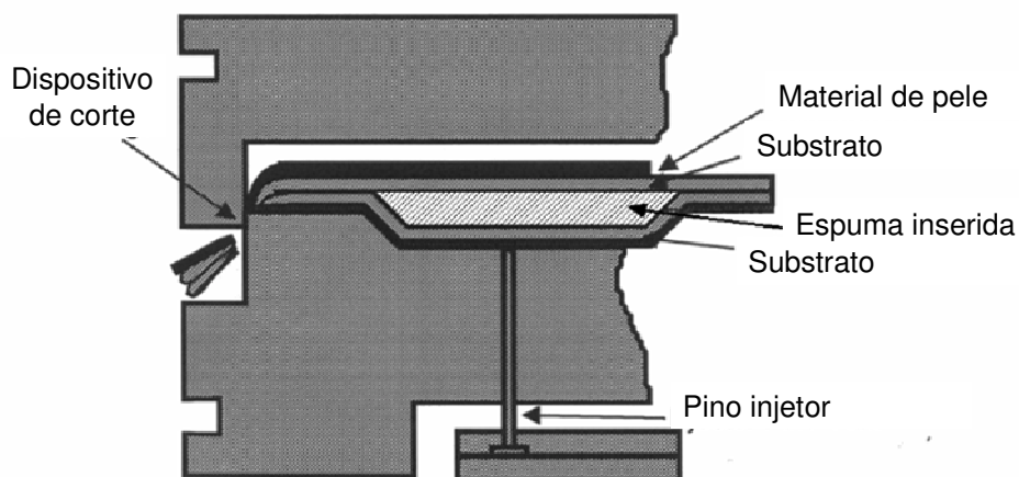
Figura 29. Tecnologia Stressed Skinned Sandwich.
