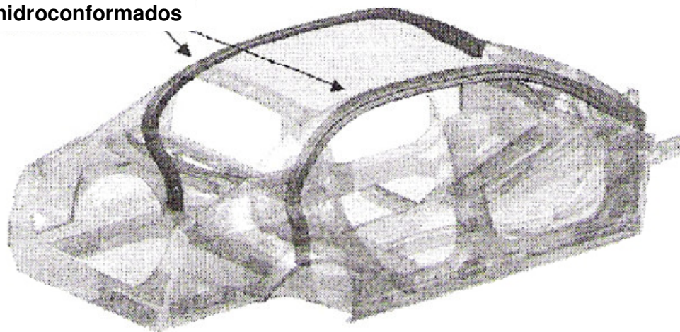
Figura 21 – Membro tubular lateral da carroceria (ULSAB-AVC Classe PNGV)
