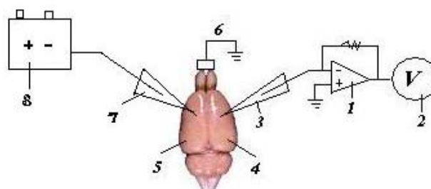
Figura 8. Esquema de registro do eletrocorticograma (ECoG). 1. Amplificador. 2. Sistema de registro e aquisição do ECoG. 3. Microeletrodo extracelular. 4. hemisfério cerebral direito e 5. esquerdo. 6. eletrodo de referência. 7. eletrodo de estimulação. 8. sistema de estimulação
