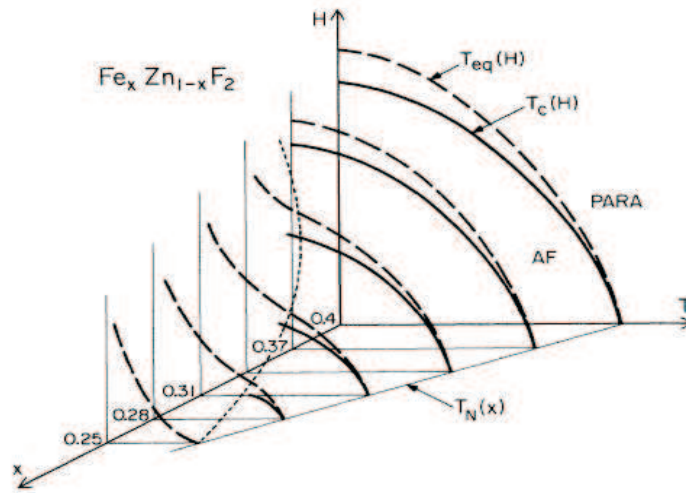
Figura 3.20: Diagrama de fases do composto Fe_x Zn_{1-x} F_2 , campo magnético contra temperatura, para diversos valores da concentração x . A linha T_c(H) representa a fronteira crítica entre as fases Paramagnética e Antiferromagnética. A linha T_{eq}(H) está associada a efeitos de irreversibilidade e é normalmente associada à linha AT. A linha T_N(H) representa a temperatura de Neil para diferentes valores de x (da Ref. [22]).
