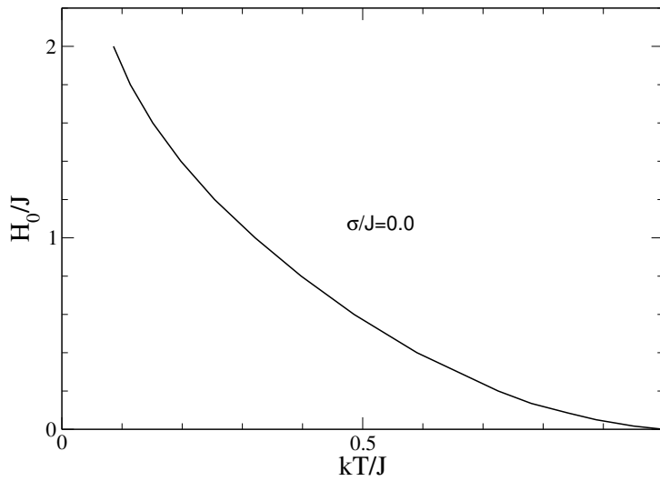
Figura 3.17: Linha de Almeida-Thouless no diagrama média do campo magnético contra temperatura ( J_o = 0 ). Para o valor de \sigma/J indicado, não observamos mudança na concavidade da curva.
