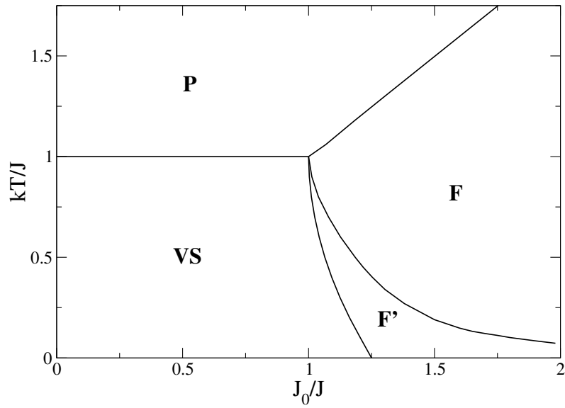
Figura 2.4: Diagrama de fases para o modelo de Sherrington-Kirkpatrick, no plano temperatura versus interação média (em unidades de J ), levando em conta a linha de Almeida-Thouless. As fases são: Paramagnética (P), Vidro de Spins (VS), Ferromagnética (F) e Ferromagnética mista (F').
