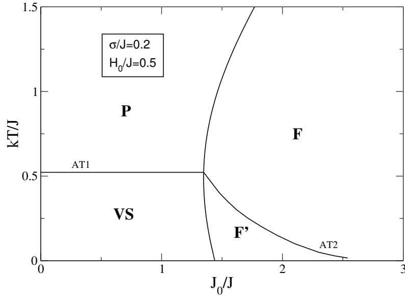
Figura 3.2: Diagrama de fases para o vidro de spins de Ising com favorecimento ferromagnético, na presença de campos magnéticos aleatórios obedecendo uma distribuição do tipo gaussiana dupla. O diagrama é exibido no plano temperatura versus média das interações (em unidades de J ). Os valores dos parâmetros \sigma e H_o estão indicados. As fases são: Paramagnética (P), Ferromagnética (F), Ferromagnética Mista (F') e Vidro de Spins (VS). As linhas de instabilidade de Almeida-Thouless estão indicadas por AT1 e AT2, sinalizando o limite de validade da solução com simetria de réplicas. Neste caso temos apenas fronteiras críticas contínuas.
