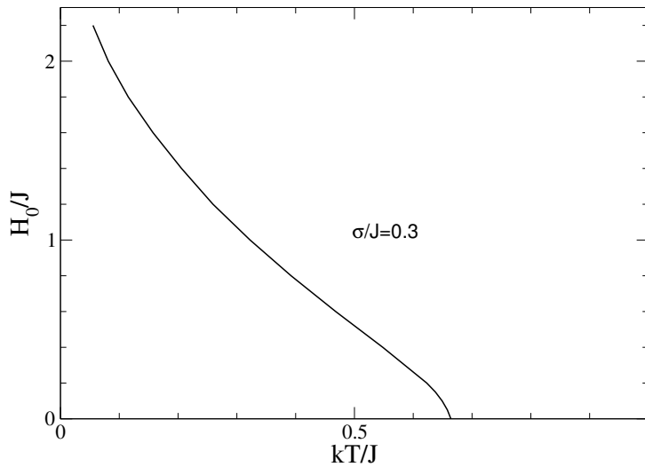
Figura 3.18: Linha de Almeida-Thouless no diagrama média do campo magnético contra temperatura ( J_o = 0 ). Para o valor de \sigma/J indicado, observamos a mudança na concavidade da curva.
