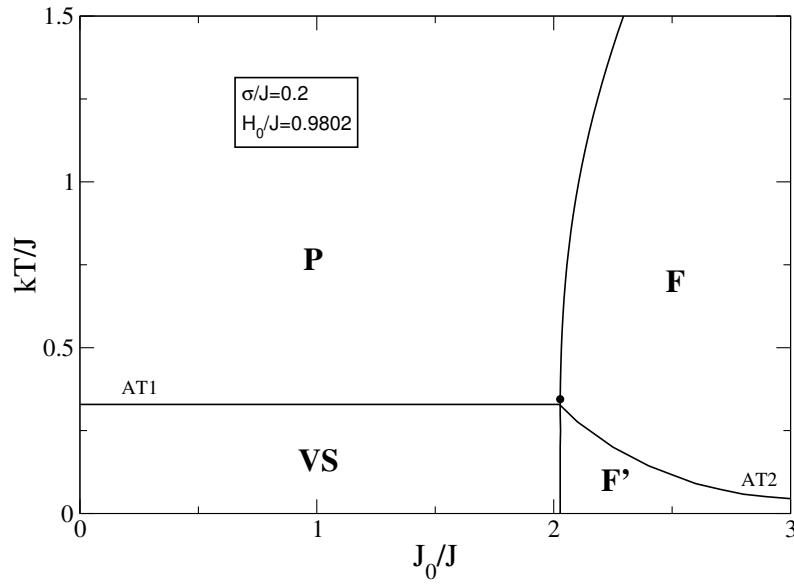
Figura 3.3: Diagrama de fases para o vidro de spins de Ising com favorecimento ferromagnético, na presença de campos magnéticos aleatórios obedecendo uma distribuição do tipo gaussiana dupla. O diagrama é exibido no plano temperatura versus média das interações (em unidades de J ). O ponto preto representa um ponto especial, um colapso de dois pontos tricríticos. A nomenclatura utilizada é a mesma da figura 3.2.
