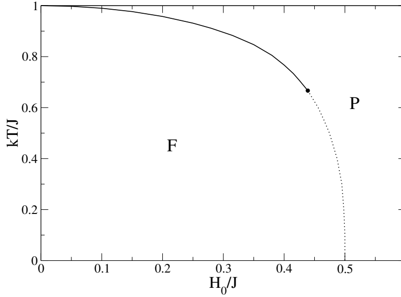
Figura 2.2: Diagrama de fases para o modelo de Ising ferromagnético sob a ação de um campo magnético aleatório obedecendo uma distribuição bimodal, no plano temperatura versus intensidade do campo magnético (em unidades de J ). As fases são: Paramagnética (P) e Ferromagnética (F). A linha pontilhada representa a fronteira crítica de primeira ordem e a linha contínua representa a fronteira crítica contínua, enquanto o ponto preto é um ponto tricrítico.
