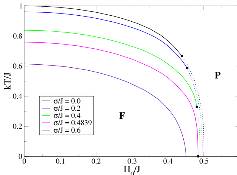
Figura 3.1: Diagrama de fases para o modelo de Ising ferromagnético sob a ação de um campo aleatório obedecendo uma distribuição do tipo gaussiana dupla, no plano temperatura versus campo magnético (em unidades de J). Os valores do parâmetro \sigma estão indicados. As fases são: Paramagnética (P) e Ferromagnética (F). Os pontos pretos representam pontos tricríticos.
