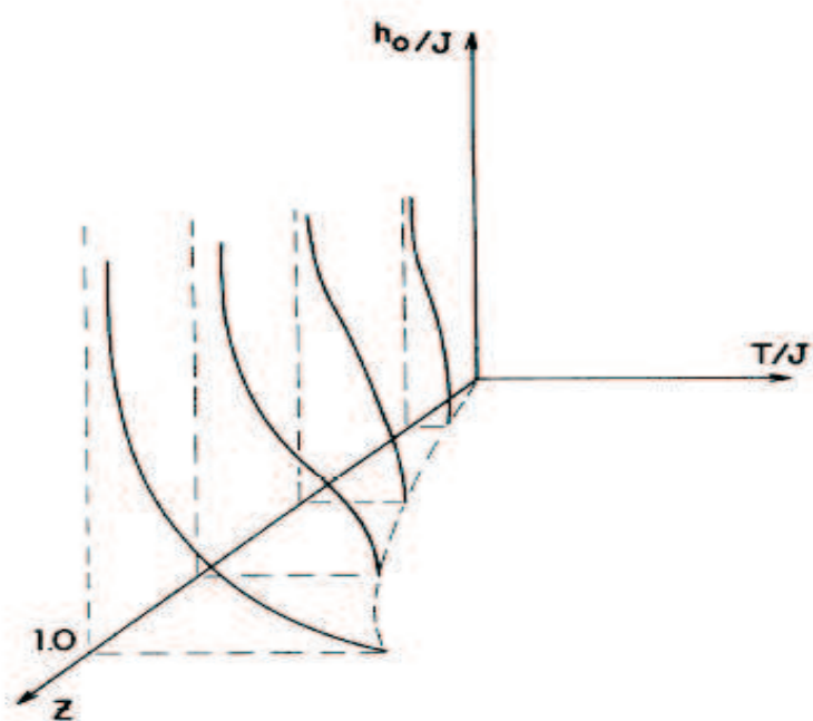
Figura 3.21: Evolução da linha de Almeida-Thouless com a variação de \sigma/J [ z = 1/(1+\sigma/J) ]. A região de instabilidade é reduzida com o aumento de \sigma/J (da Ref. [38]). As variáveis da figura apresentam a seguinte correspondência com as nossas: h_o \rightarrow H_o e k = 1 .
