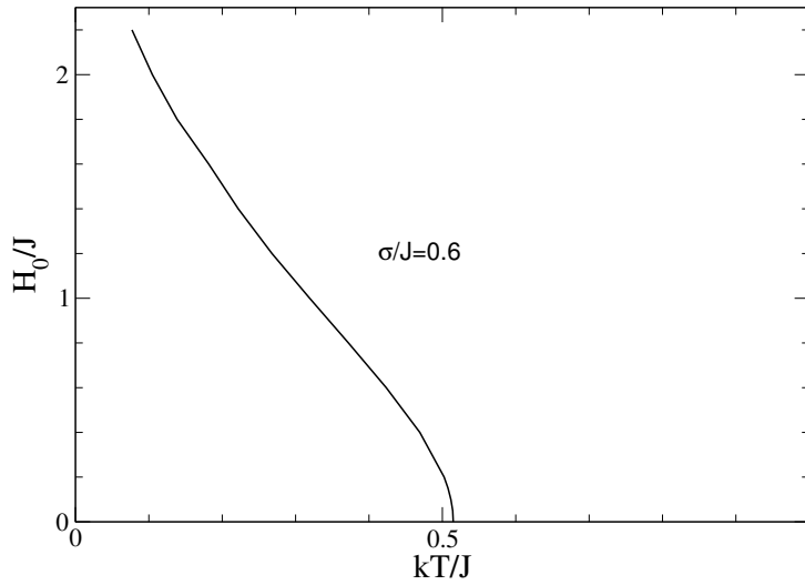
Figura 3.19: Linha de Almeida-Thouless no diagrama média do campo magnético contra temperatura ( J_o = 0 ). Para o valor de \sigma/J indicado, observamos uma mudança ainda maior na concavidade da curva.
