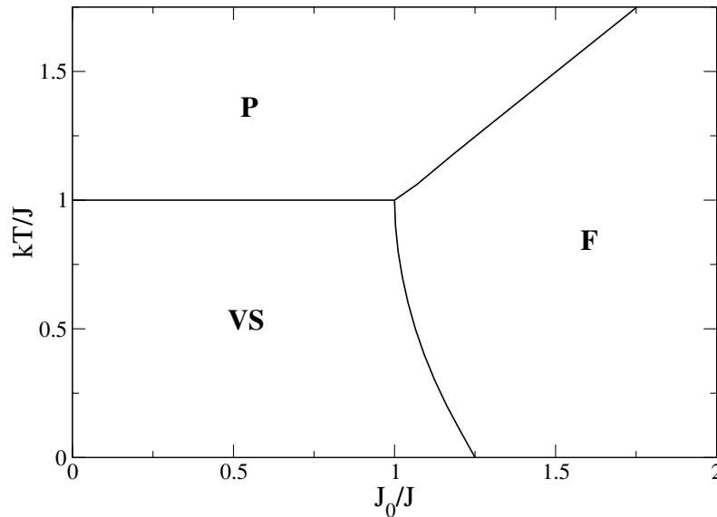
Figura 2.3: Diagrama de fases para o modelo de Sherrington-Kirkpatrick, no plano temperatura versus média das interações (em unidades de J). As fases são: Paramagnética (P), Vidro de Spins (VS) e Ferromagnética (F).
