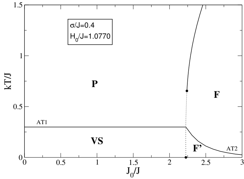
Figura 3.10: Diagrama de fases para o vidro de spins de Ising com favorecimento ferromagnético, na presença de campos magnéticos aleatórios obedecendo uma distribuição do tipo gaussiana dupla. O diagrama é exibido no plano temperatura versus média das interações (em unidades de J ). Para os valores de \sigma/J e H_o/J mostrados, temos a existência de dois pontos tricríticos, sendo que um deles colapsa com o eixo kT/J = 0 . A nomenclatura utilizada é a mesma das figuras 3.2 e 3.4.
