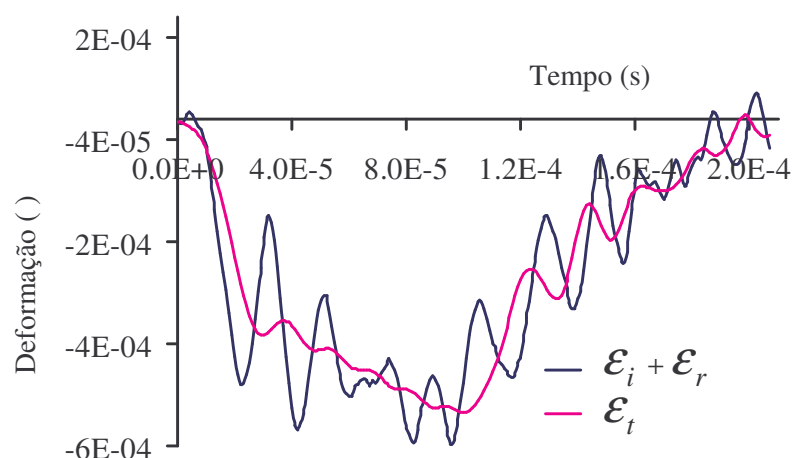
Fig. 6.3.13 –equilíbrio de deformações nas faces do corpo de prova da modelo nº2 com modulador de aço.
