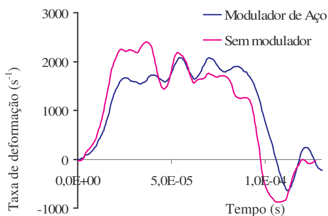
Fig. 6.3.14.- taxa de deformação de engenharia do corpo de prova da modelo nº2 sem e com modulador de aço.
