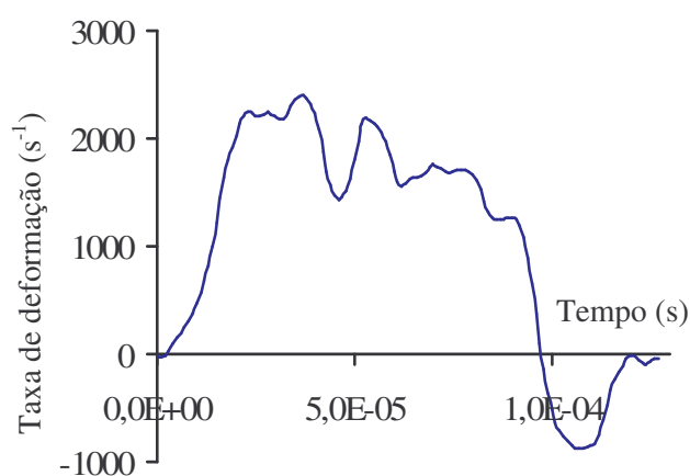
Fig. 6.3.7 – taxa de deformação de engenharia do corpo de prova
