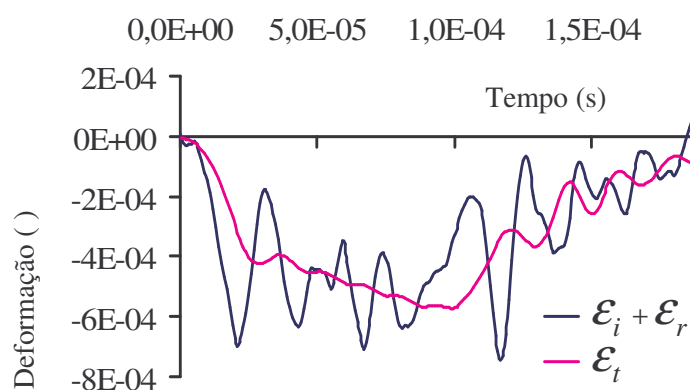
Fig. 6.3.10 – equilíbrio de deformações nas faces do corpo de prova da modelo nº2 com modulador de Cobre.
