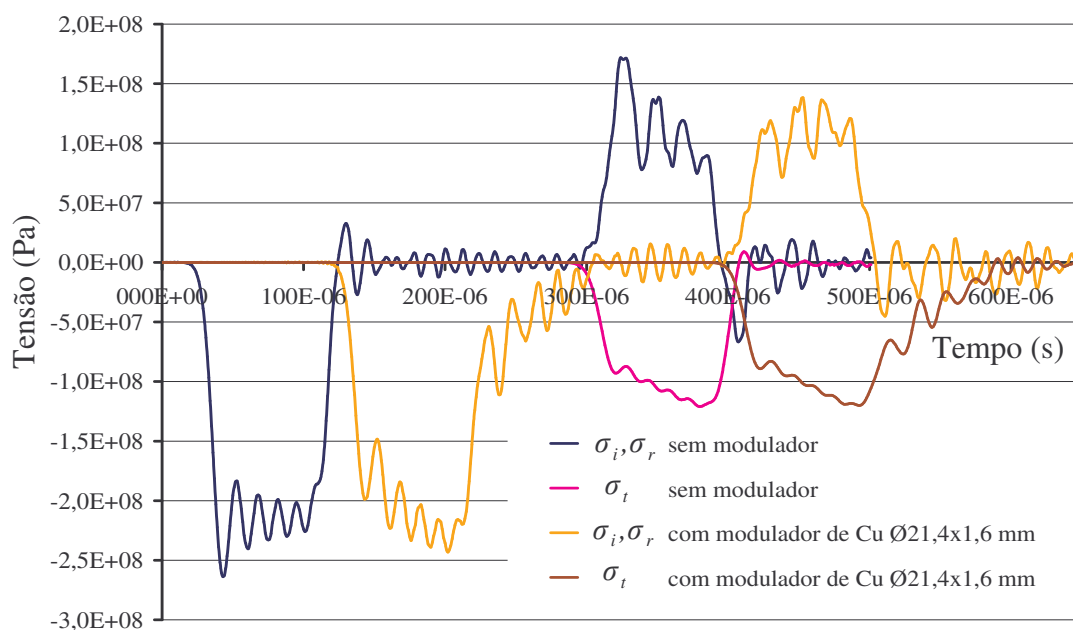
Fig. 6.3.9 – pulsos de tensão simulados para modelo nº2 sem e com modulador. Os pulsos sem modulador encontram-se 100 ms adiantados para melhor comparação.
