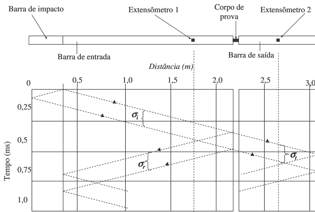
Fig. 3.1.2: Propagação de ondas na barra de Hopkinson de compressão
