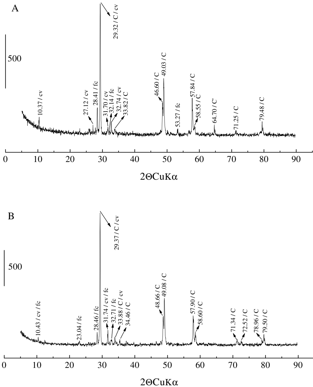
Figura 35: Difrátogramas de Raios X dos resíduos sólidos de biolixiviação dos experimentos em que as células bacterianas não adaptadas (A) e adaptadas (B) foram adicionadas anteriormente aos íons \text{Cl}^- . Símbolos: C – calcopirita; cv – covelita; fc – compostos fosfatados de calcio.
