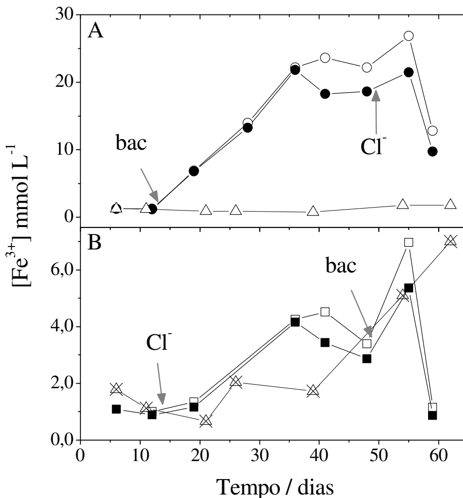
Figura 29: Variação da concentração de Fe^{3+} nos ensaios de lixiviação da calcopirita da primeira (A) e segunda (B) séries utilizando-se bactéria adaptada (símbolos fechados) e não adaptada (símbolos abertos). Além de ensaios controles que continham solução A do meio T&K sem (8) e com (:) 200 mmol L^{-1} de íons Cl^{-} . As setas indicam o momento das adições.
