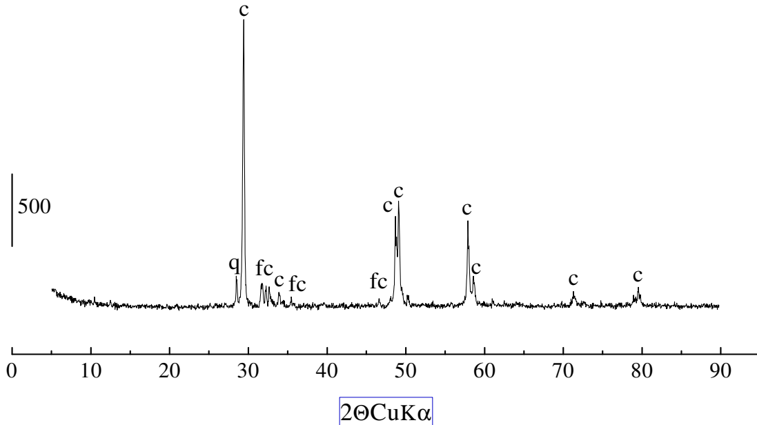
Figura 6: difratograma de raios X do concentrado de calcopirita utilizado. A barra lateral indica a intensidade dos picos e os símbolos indicam c - calcopirita ( \text{CuFeS}_2 ), q - quartzo ( \text{SiO}_2 ) e fc – compostos fosfatados de cálcio.
