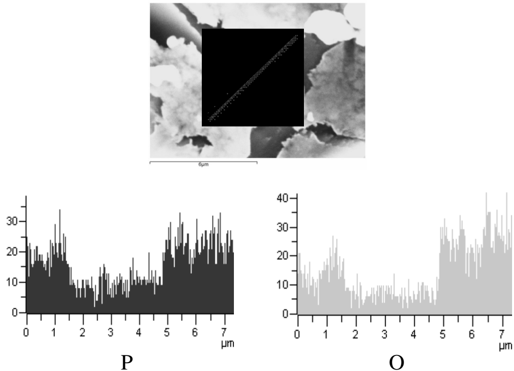
Figura 32: Análise linear SEM-EDS para os elementos fósforo e oxigênio nos resíduos sólidos dos ensaios em que células bacterianas adaptadas foram adicionadas na ausência de íons \text{Cl}^- (primeira série). A linha sobre a qual foi realizada a análise EDS está ilustrada na imagem.
