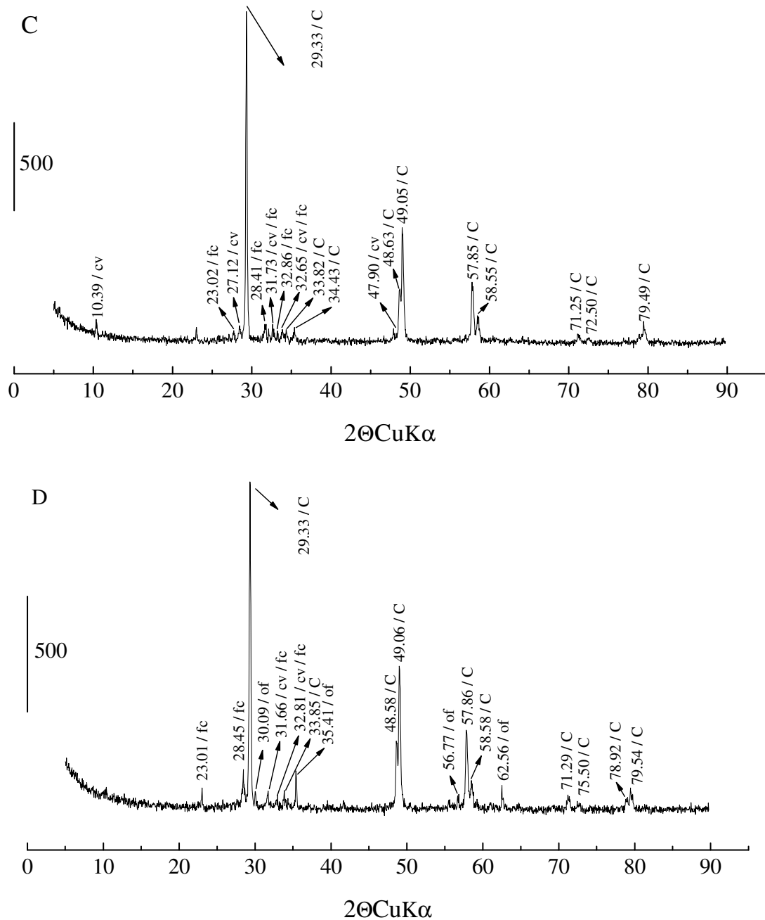
Figura 36: Difractogramas de Raios X dos resíduos sólidos de biolixiviação dos experimentos em que os íons \text{Cl}^- foram adicionados anteriormente às células bacterianas não adaptadas (C) e adaptadas (D). Símbolos: C – calcopirita; cv – covelita; fc – compostos fosfatados de cálcio; of – óxido de ferro, \text{Fe}_3\text{O}_4 .
