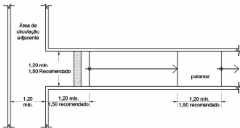
Vista superior
