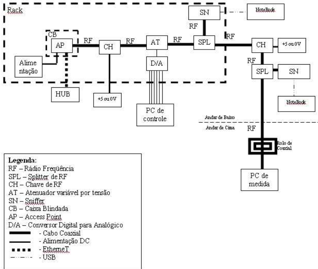
Figura 1: Diagrama em blocos da bancada de emulação.
