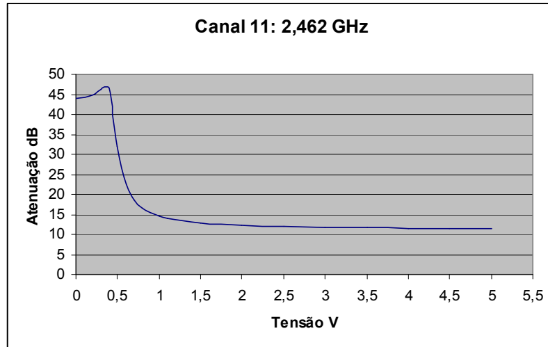
Figura 11: Atenuação da chave 1 no canal 11.
