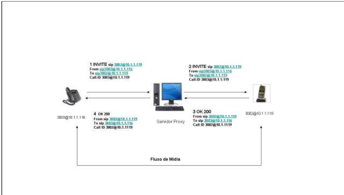
Figura 8: Troca de mensagens com um Proxy Server
