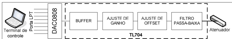
FIGURA 7 – Bloco de controle
