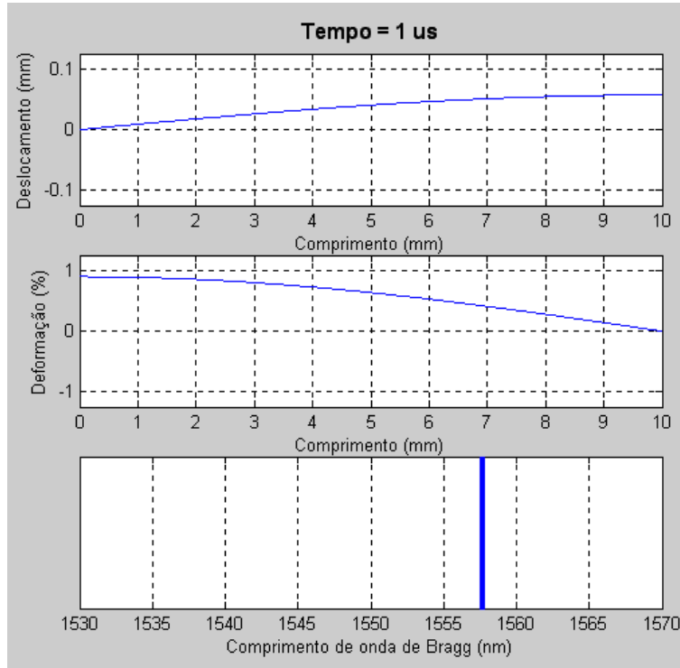
Figura 3.16: Deslocamento, deformação e comprimento de onda de Bragg no instante t = 1 \mu\text{s} considerando o amortecimento.
