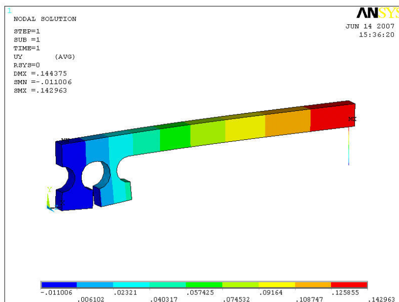
Figura 5.9: Simulação da mola de entalhe com a fibra colada a 5 mm da sua extremidade e uma força de 100 N aplicada na base do suporte livre.
