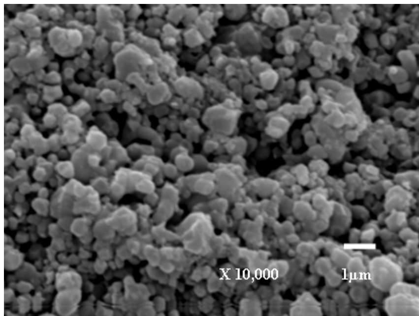
FIG. 4.32 Micrografia do compósito Al 2 O 3 -YAG sinterizado a 1400 °C, por 4h, cortado, com 3 min de deposição de Au e aumento de 10.000 X
