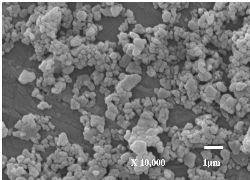
FIG. 4.2 Micrografia do Al 2 O 3 como recebido, com a região central da FIG. 4.1 em destaque, com aumento de 10.000X
