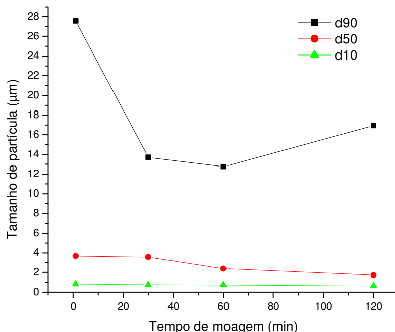
FIG. 4.12 Tamanho de partícula em função do tempo de moagem da mistura Al_2O_3 - Y_2O_3
