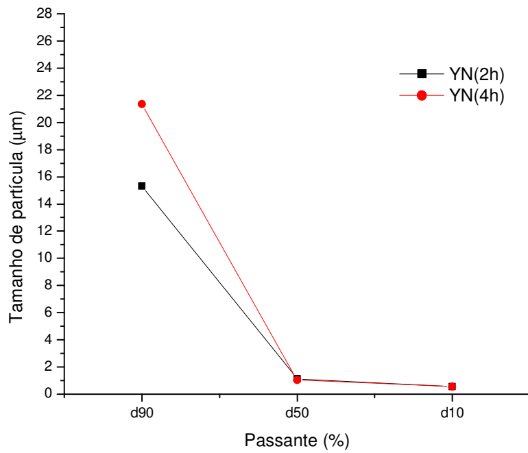
FIG. 4.14 Tamanho de partícula em função do percentual passante para o composto \text{Al}_2\text{O}_3\text{-YAG} com \text{Nb}_2\text{O}_5
