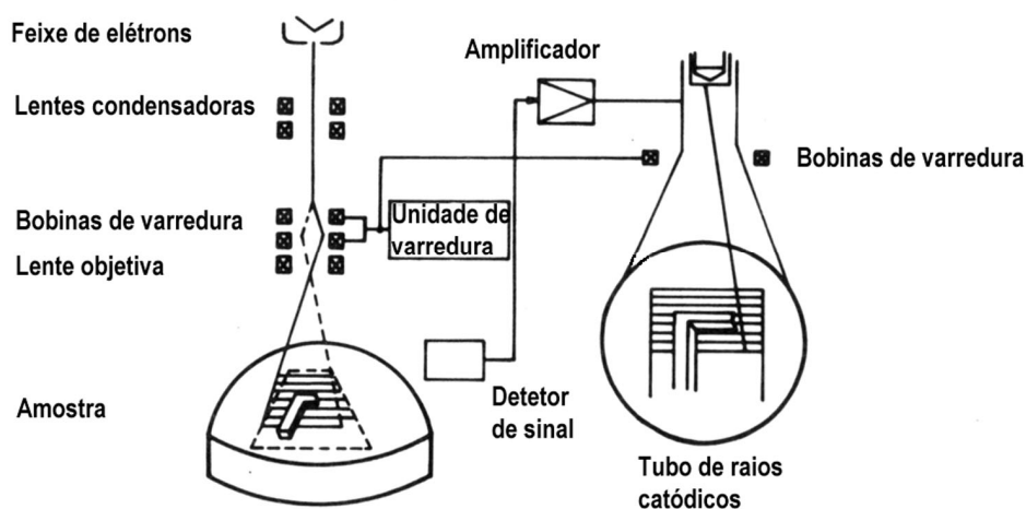
FIG. 3.1 Representação esquemática dos componentes do MEV (MANNHEIMER, 2002)
