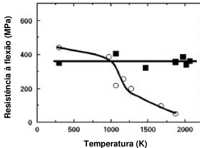
FIG. 2.11 Dependência com a temperatura da resistência à flexão do compósito eutético (■) e do compósito policristalino (○) (WAKU, 1998, p. 1217-25)
