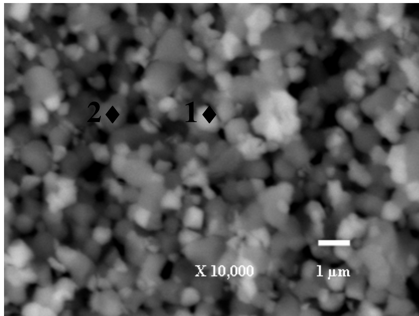
FIG. 4.38 Microestrutura do compósito \text{Al}_2\text{O}_3 -YAG sinterizado a 1450\text{ }^\circ\text{C} , por 2h, cortado, observado por BSE, sem deposição de Au, com os pontos indicativos do EDS
