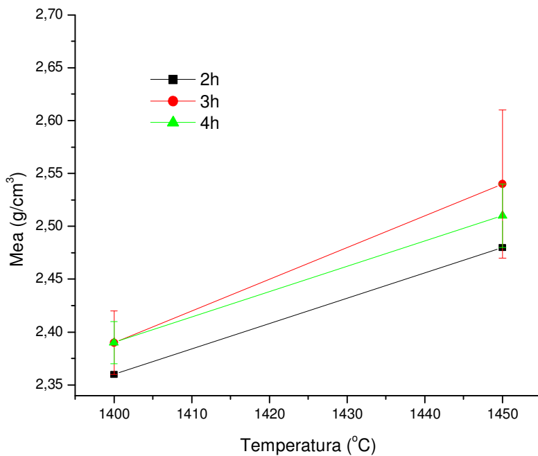
FIG. 4.19 Valores de densidade do compósito sinterizado \text{Al}_2\text{O}_3 -YAG com \text{Nb}_2\text{O}_5
