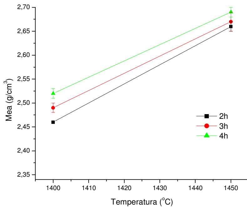
FIG. 4.18 Valores de densidade do compósito sinterizado \text{Al}_2\text{O}_3 -YAG
