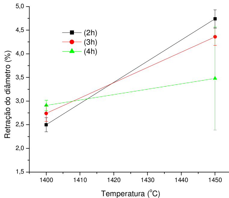
FIG. 4.22 Retração do diâmetro do compósito sinterizado \text{Al}_2\text{O}_3 -YAG
