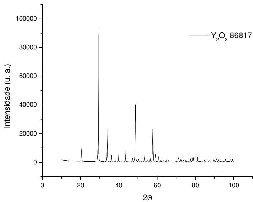
FIG. 4.16 Difratoograma do Y 2 O 3
