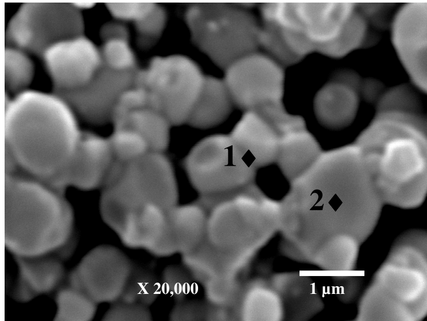
FIG. 4.41 Microestrutura do compósito \text{Al}_2\text{O}_3 -YAG com \text{Nb}_2\text{O}_5 sinterizado a 1450\text{ }^\circ\text{C} , por 2h, lixado e polido, observado por SE, com as regiões indicativas do EDS, com aumento de 20.000 X
