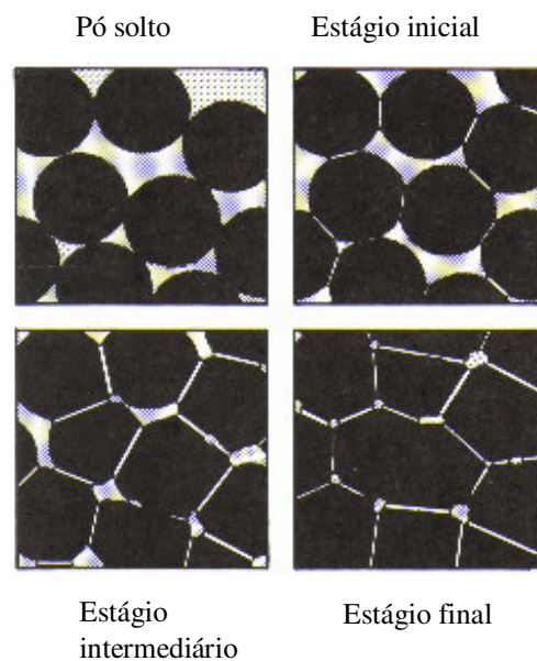
FIG. 2.6 Estágios de sinterização em estado sólido (GERMAN, 1996)
