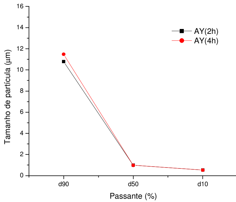
FIG. 4.13 Tamanho de partícula em função do percentual passante para o composto \text{Al}_2\text{O}_3\text{-YAG}
