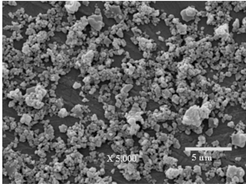
FIG. 4.1 Micrografia do Al 2 O 3 como recebido, com aumento de 5.000X
