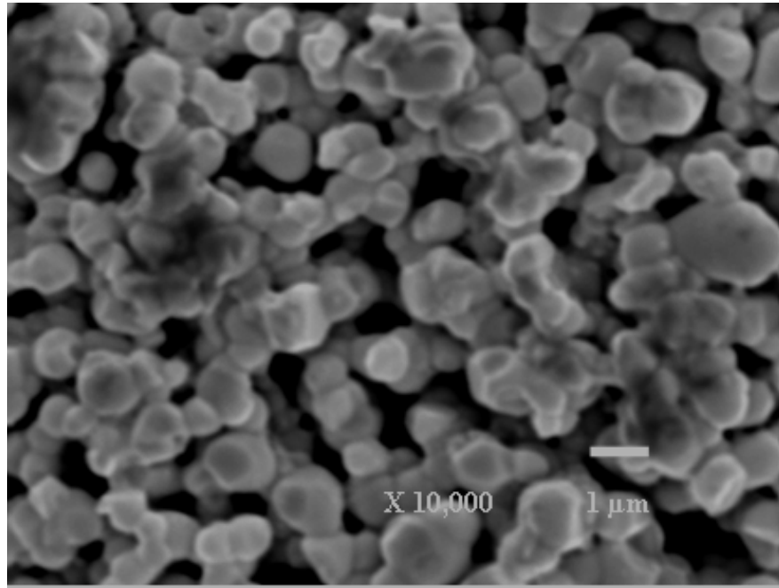
FIG. 4.35 Microestrutura do compósito \text{Al}_2\text{O}_3 -YAG com \text{Nb}_2\text{O}_5 sinterizado a 1450\text{ }^\circ\text{C} , por 3h, lixado e embutido em baquelite, com 3 min de deposição de Au, com 10.000 X
