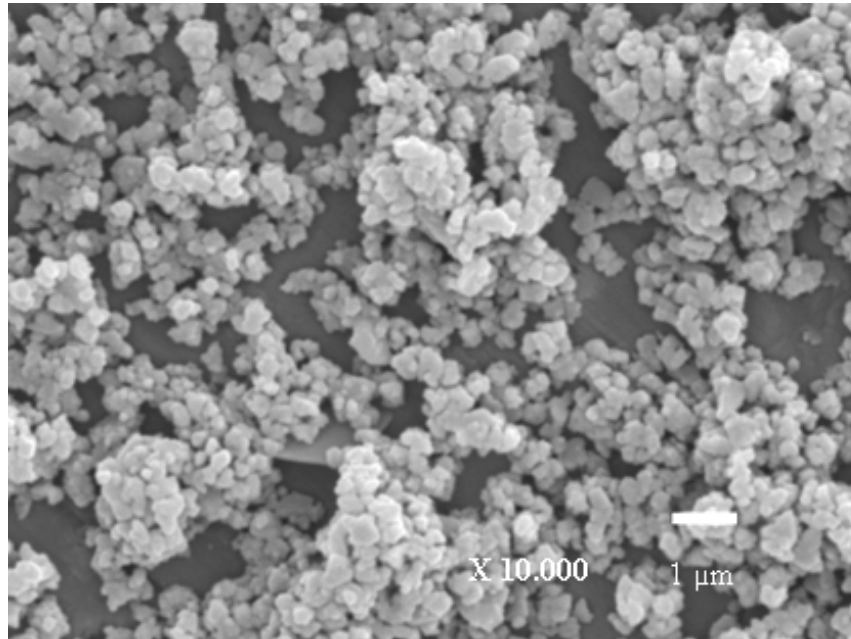
FIG. 4.9 Micrografia da mistura \text{Al}_2\text{O}_3\text{-Y}_2\text{O}_3 com 120 min de moagem, com a região central da FIG.4.8 em destaque e aumento de 10.000X
