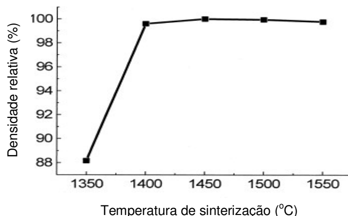
FIG. 2.17 Densidade relativa x temperatura de sinterização do compósito \text{Al}_2\text{O}_3\text{-25\% vol YAG} por HP (LI, 1999, p. 1073-1080)
