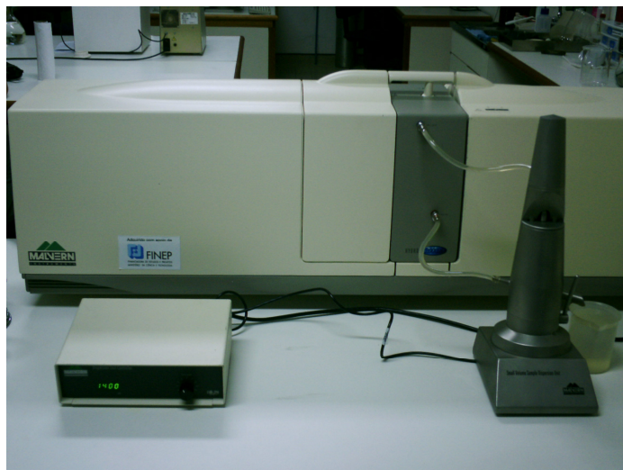
FIG. 3.3 Equipamento de granulometria a laser da MALVERN
