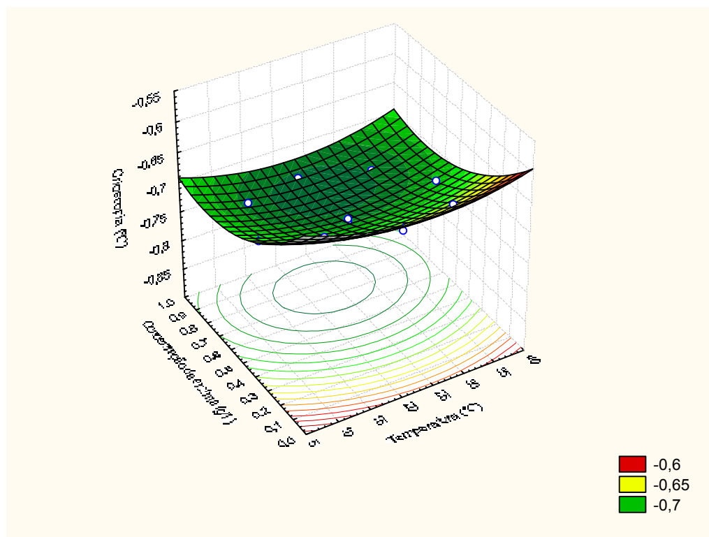
Figura 9 – Crioscopia do leite conforme temperatura e concentração da enzima lactase
