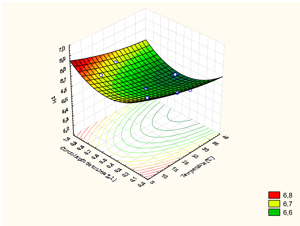
Figura 4 – pH do leite conforme temperatura e concentração da enzima lactase 1.
