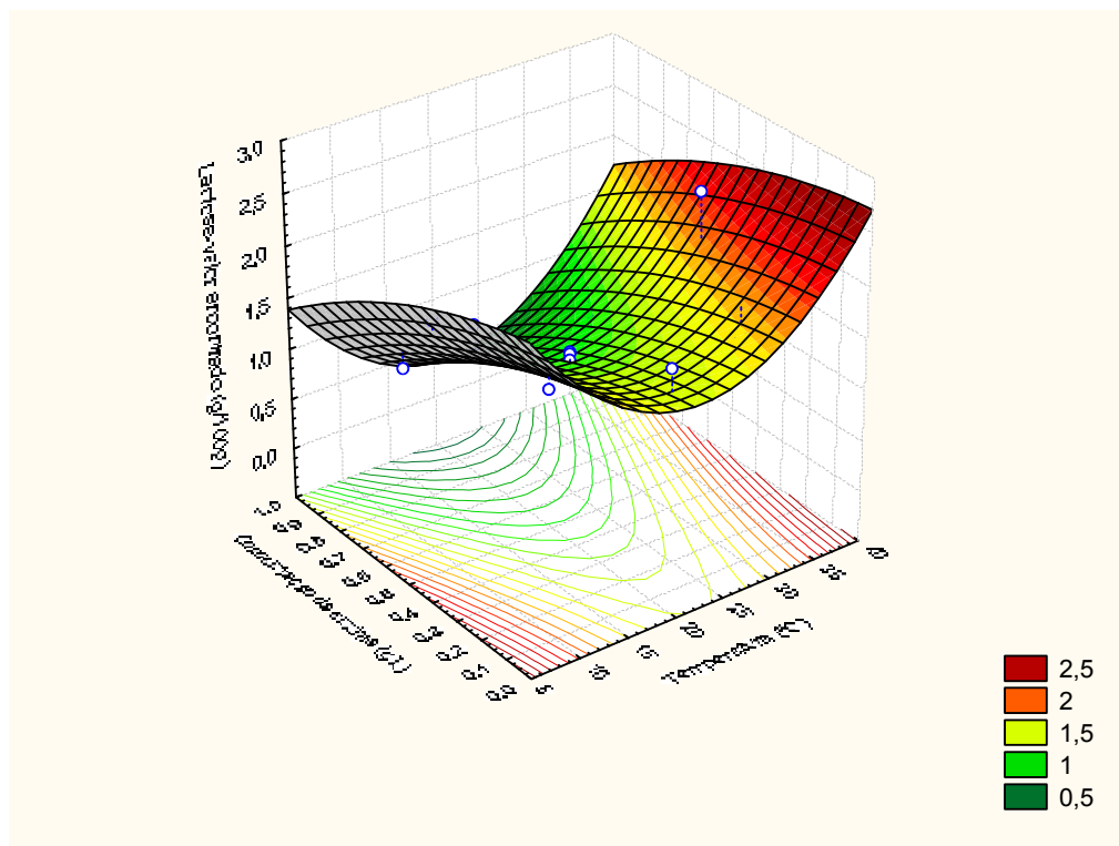
Figura 16 – Valor encontrado de lactose, conforme temperatura e concentração da enzima lactase 1.
