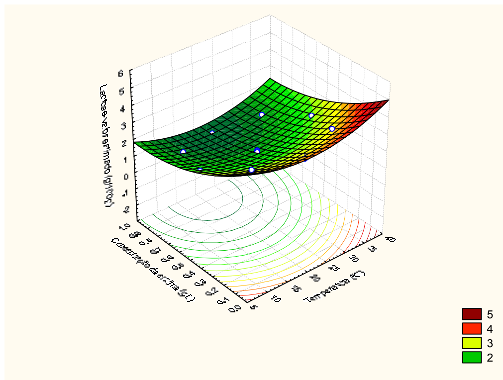
Figura 12 – Valor estimado de lactose final conforme temperatura e concentração da enzima lactase 1.
