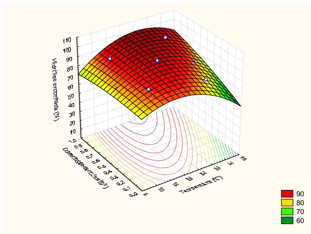
Figura 15 – Percentual de hidrólise encontrada, conforme temperatura e concentração da enzima lactase 2.
