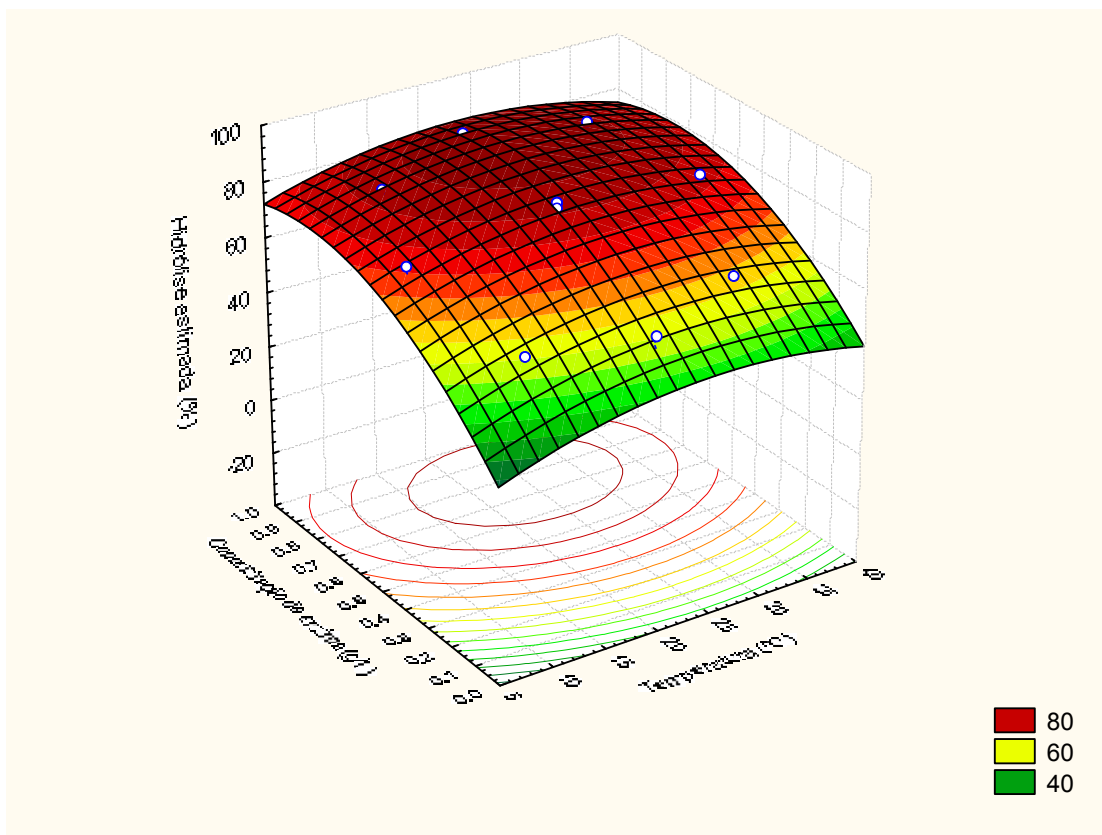
Figura 11 – Percentual de hidrólise estimada, conforme temperatura e concentração da enzima lactase 2.
