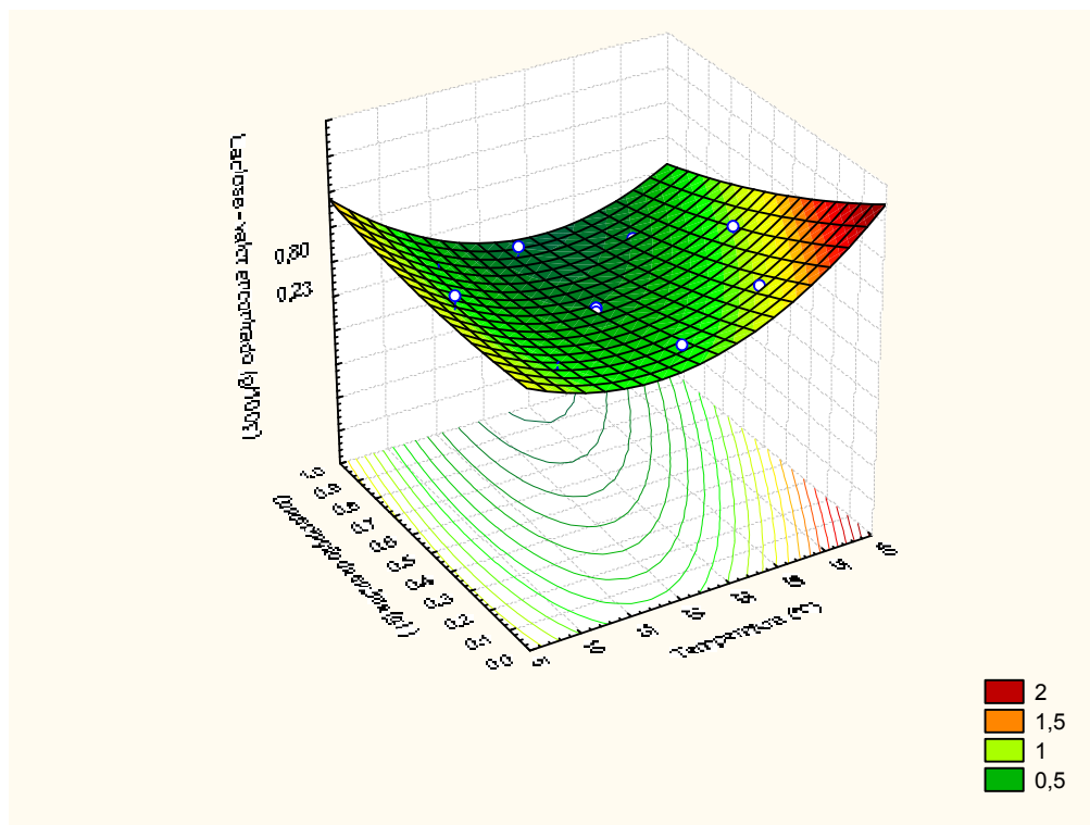
Figura 17 – Valor encontrado de lactose, conforme temperatura e concentração da enzima lactase 2.
