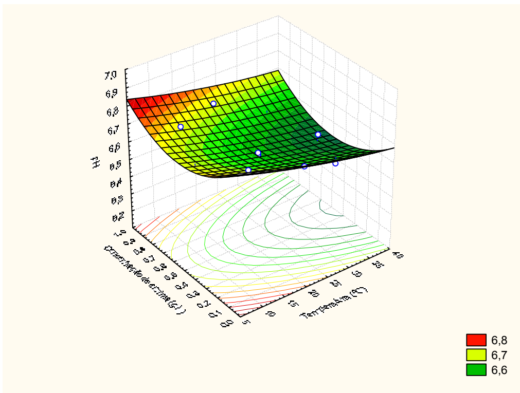
Figura 5 – pH do leite conforme temperatura e concentração da enzima lactase 2.
