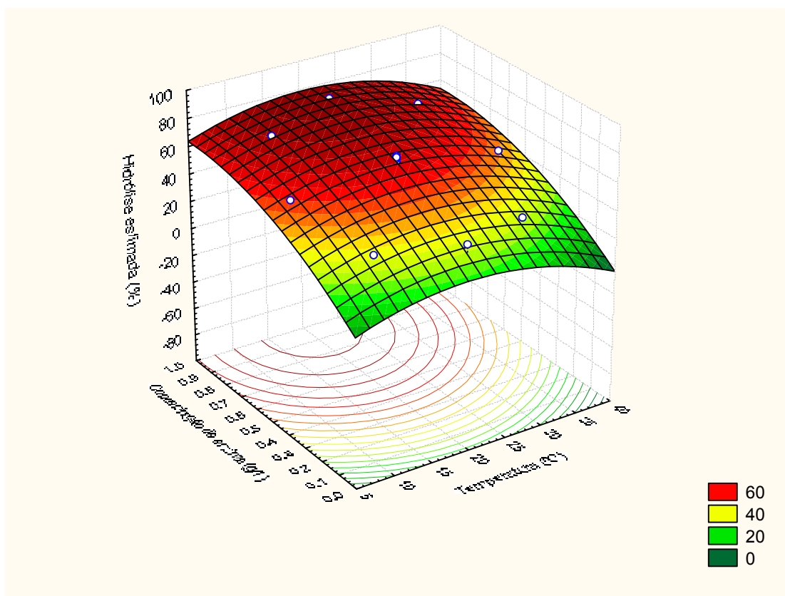
Figura 10 – Percentual de hidrólise estimada, conforme temperatura e concentração da enzima lactase 1.
