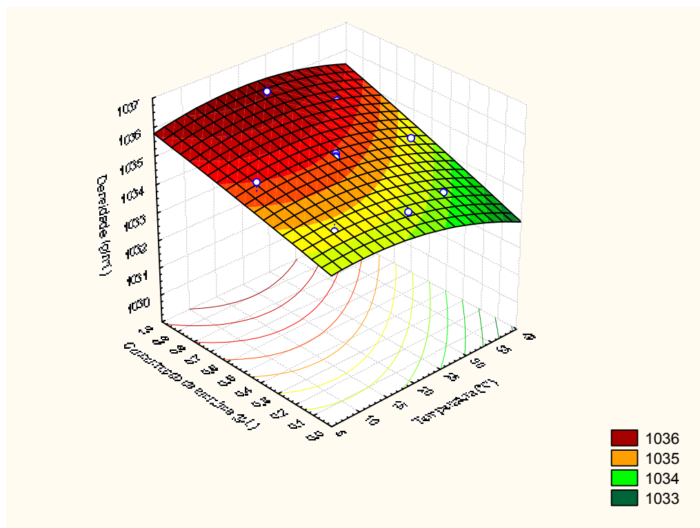
Figura 6 – Densidade do leite conforme temperatura e concentração da enzima lactase1.
