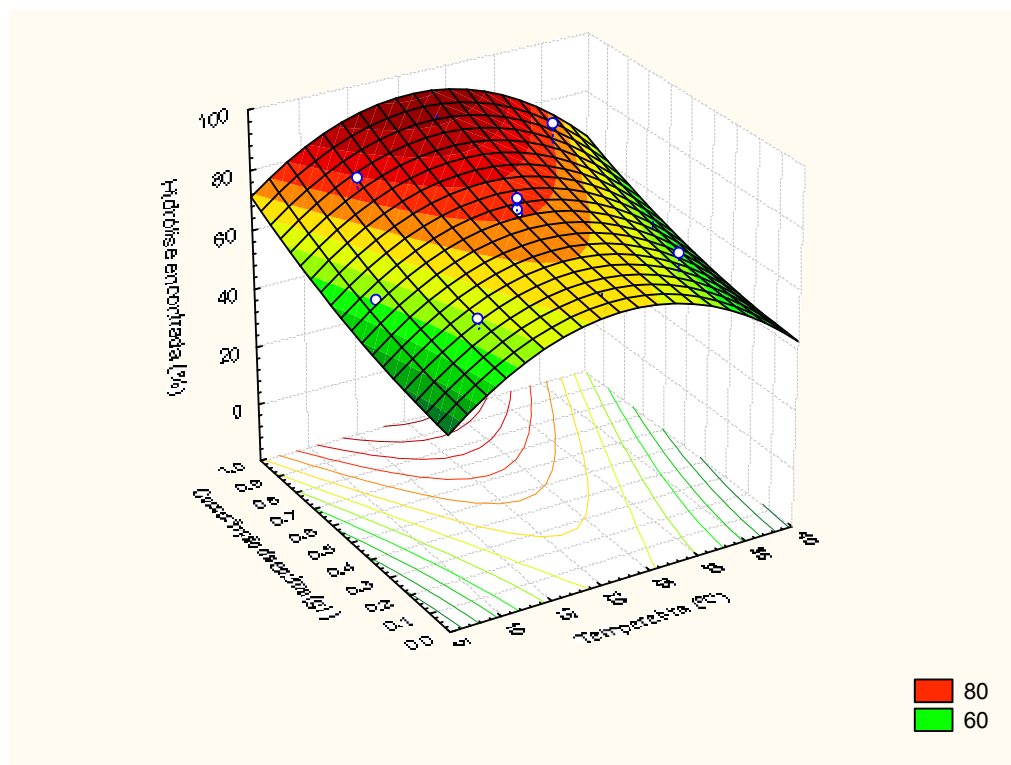
Figura 14 – Percentual de hidrólise encontrada, conforme temperatura e concentração da enzima lactase 1.
