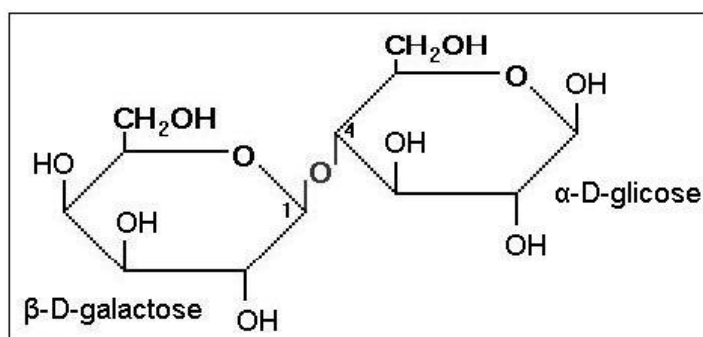
Figura 1 – Estrutura química da lactose.
