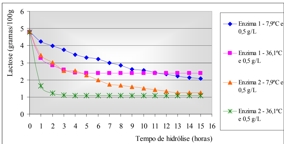
Figura 21 – Valor estimado de lactose durante a hidrólise, para as enzimas 1 e 2, nas temperaturas de 7,9 e 36,1 °C e na concentração de enzima de 0,5 g/L.
