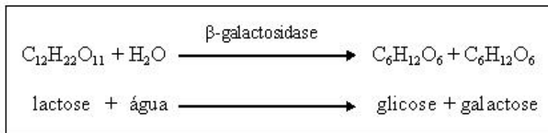
Figura 2 – Hidrólise da lactose.
