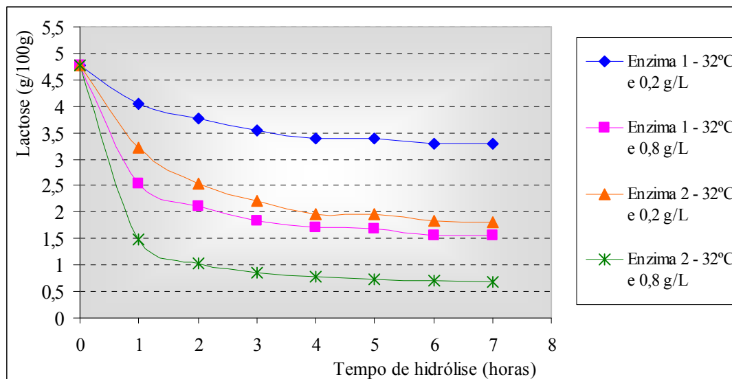
Figura 20 – Valor estimado de lactose durante a hidrólise, para as enzimas 1 e 2, na temperatura de 32 °C e nas concentrações de enzima de 0,2 e 0,8 g/L.
