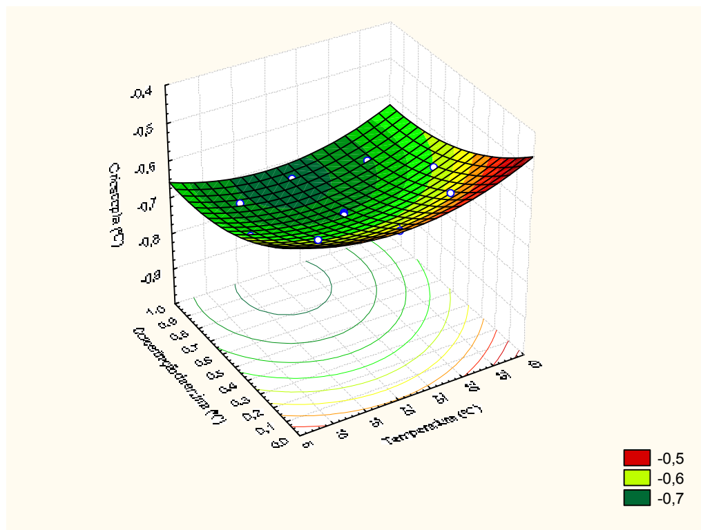
Figura 8 – Crioscopia do leite conforme temperatura e concentração da enzima lactase
