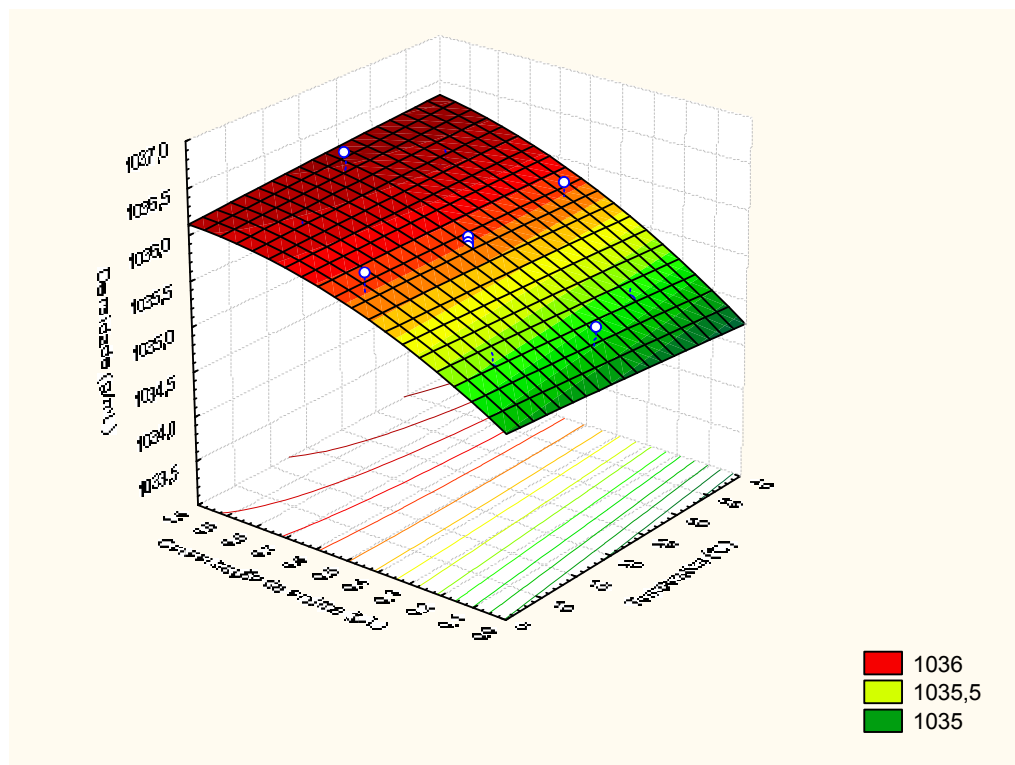
Figura 7 – Densidade do leite conforme temperatura e concentração da enzima lactase
