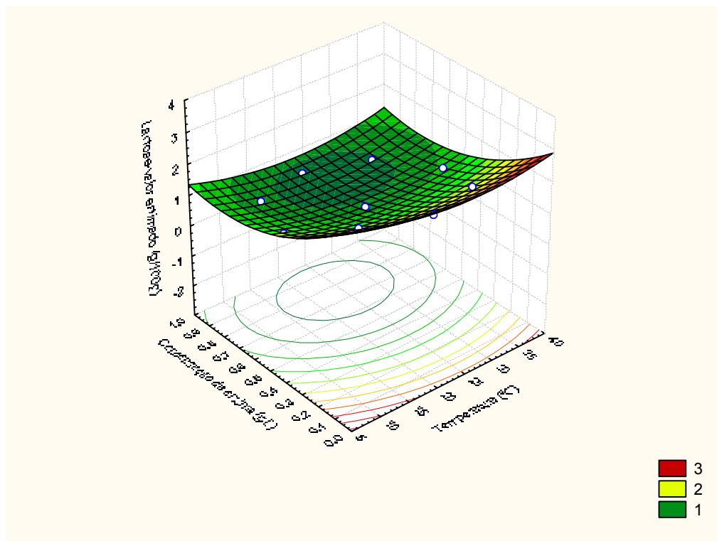
Figura 13 – Valor estimado de lactose final conforme temperatura e concentração da enzima lactase 2.
