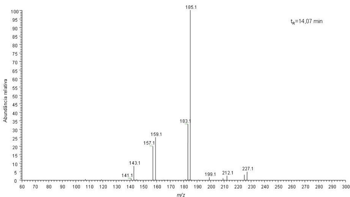
Figura 28. Espectro de massas (MS/MS) do composto no tempo de retenção 14,07 min para ser comparado com o espectro de massas do padrão de resveratrol (Figura 26)
