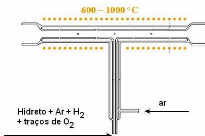
Figura 7. Segundo modelo proposto para o multiatomizador de quartzo (MMQTA). 41
