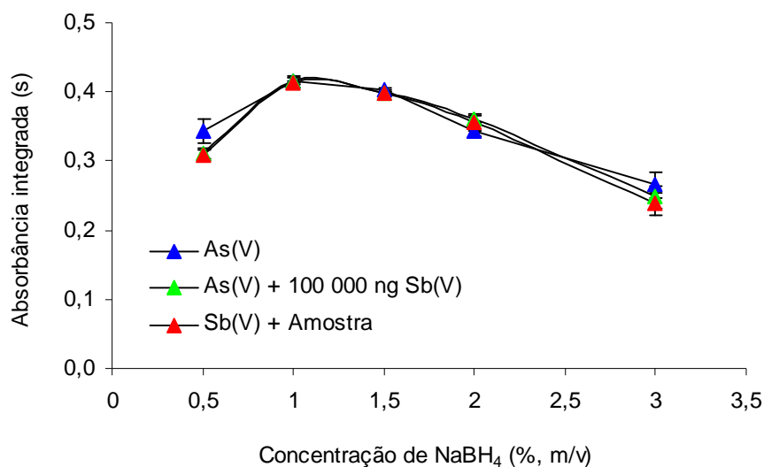
Figura 27. Influência da concentração de NaBH 4 na geração de hidretos de As(V), As(V) + Sb(V) e As(V) + solução da amostra previamente oxidada (solução de ácido cítrico 10% (m/v); tempo de purga de 10 s; tempo de contato de 1 h), utilizando o QTA como atomizador.
