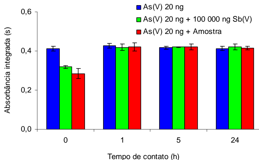
Figura 25. Influência do tempo de contato da solução analítica de As(V), As(V) + Sb(V) e As(V) + solução da amostra previamente oxidada (solução de ácido cítrico 10% (m/v); NaBH 4 1% (m/v); tempo de purga de 10 s), utilizando o QTA como atomizador.
