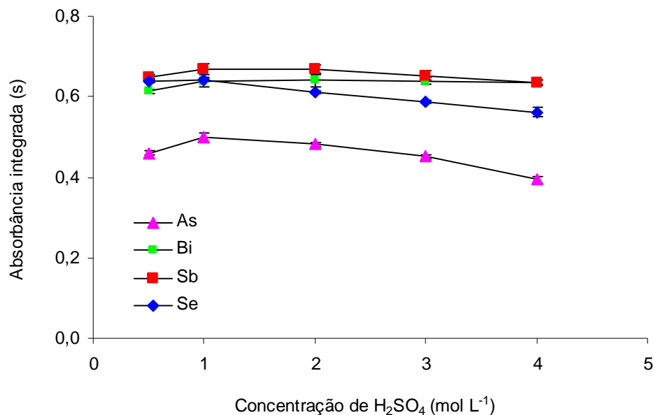
Figura 10. Influência da concentração de ácido sulfúrico na intensidade do sinal analítico de As(III), Bi(III), Sb(III) e Se(IV) (20 ng de cada elemento, NaBH 4 1,5% (m/v) e tempo de purga de 20 s), utilizando o QTA como atomizador.
