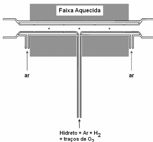
Figura 6. Primeiro modelo proposto para o multiatomizador de quartzo (MMQTA). 14
