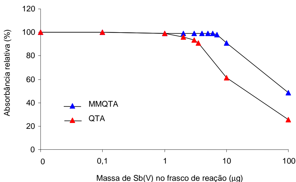
Figura 24. Interferências de Sb(V) na intensidade do sinal analítico do As(V) ( 20 \text{ ng} em 10 \text{ mL} de \text{HCl } 1 \text{ mol L}^{-1} ), utilizando ambos atomizadores.
