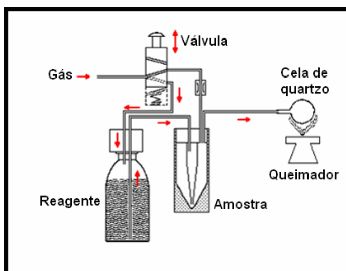
Figura 2. Sistema de geração de hidretos em batelada (Mod. MHS 10, Perkin-Elmer, adaptado de Welz e Melcher, 1983).
