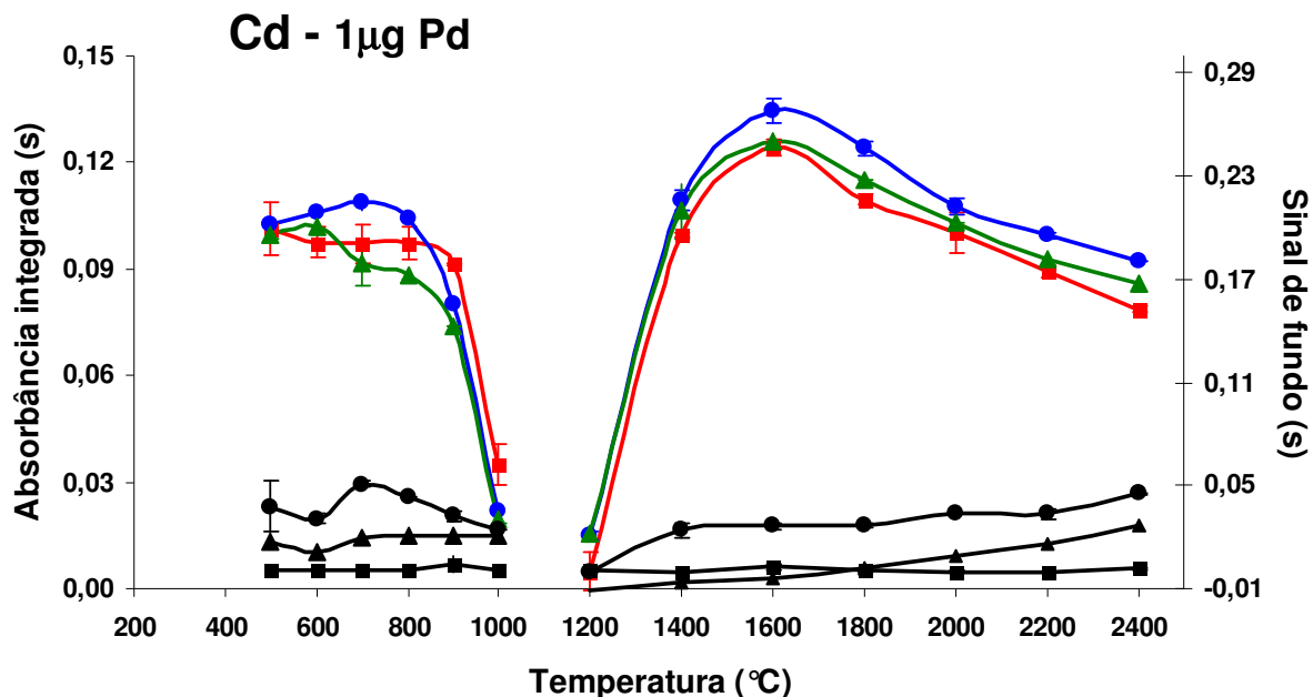
Figura 9. Curvas de pirólise e atomização obtidas com 1 µg de Pd para solução analítica de Cd (■), cloridrato de amitriptilina (●), cloridrato de imipramina (▲) na concentração de 10% (m/v). O sinal de fundo está representado pelos mesmos símbolos, porém, em preto. Cada ponto representa a média e as barras de erro representam o desvio padrão observado (n=3). A quantidade de Cd adicionada nas amostras é equivalente à concentração de 0,0125 µg g -1 .
