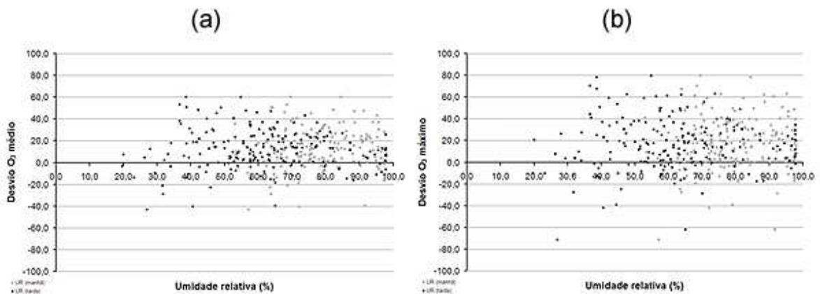
Figura 93: Relação entre os desvios das saídas de concentrações médias (a) e máximas (b) de ozônio e as médias de umidade relativa (manhã e tarde) para a RNA ajustada com dados da estação de monitoramento de qualidade do ar em Mauá.
