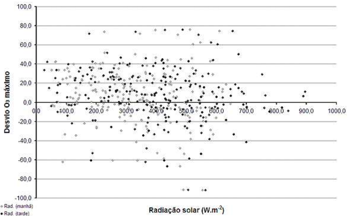
Figura 74: Relação entre os desvios (simulação-observação) das concentrações máximas de ozônio e a radiação solar de manhã e de tarde.
