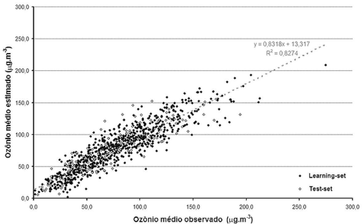
Figura 56: Relação entre valores calculados e medidos da concentração média de ozônio.
