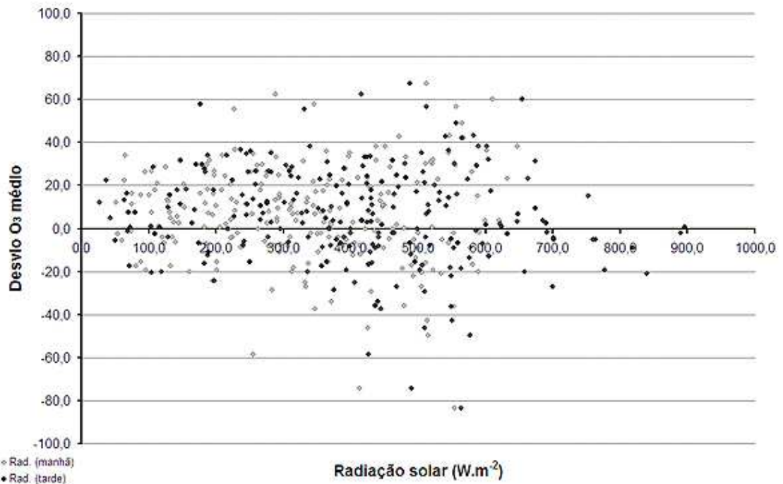
Figura 73: Relação entre os desvios (simulação-observação) das concentrações médias de ozônio e a radiação solar de manhã e de tarde.
