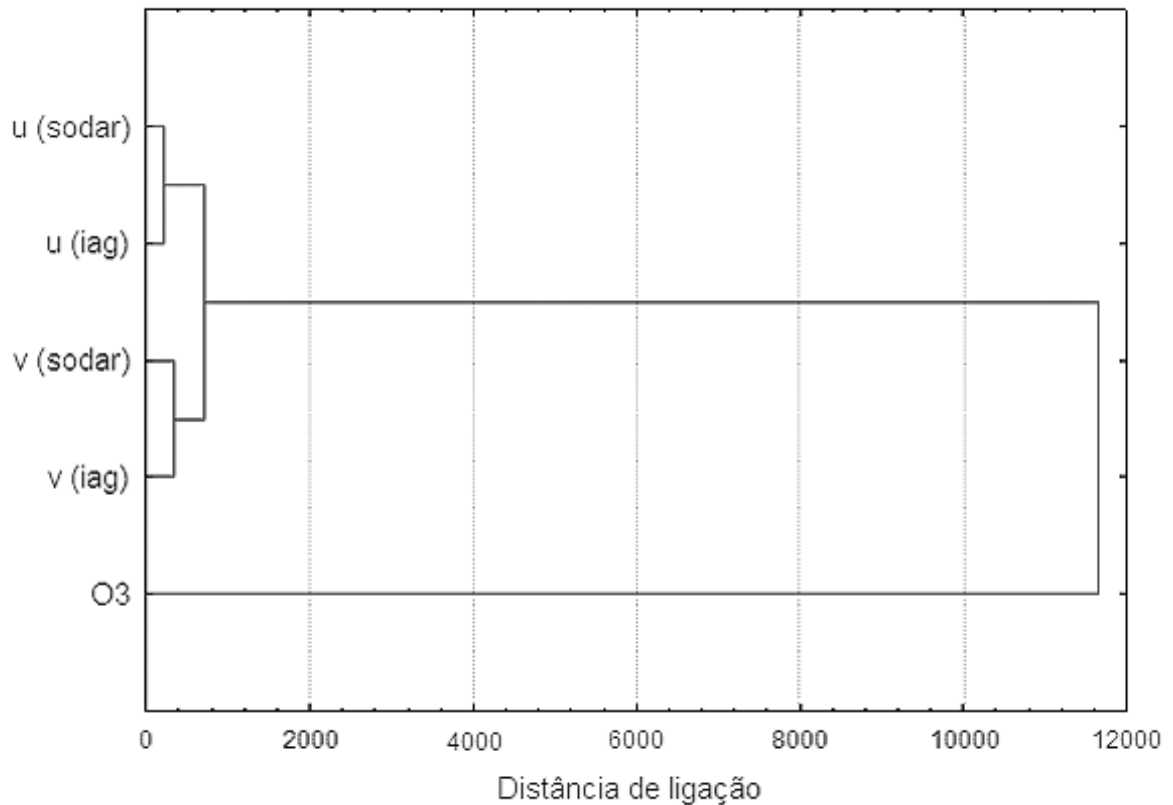
Figura 43: Dendrograma obtido da análise de agrupamento de dados de vento, considerando o método de Ward e a medida de distância euclidiana.
