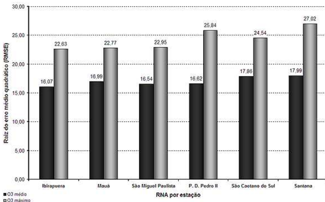
Figura 145: Raiz do erro médio quadrático ( RMSE ) para concentrações médias (preto) e máximas (cinza) de ozônio em cada rede neural artificial de cada estação de qualidade do ar.
