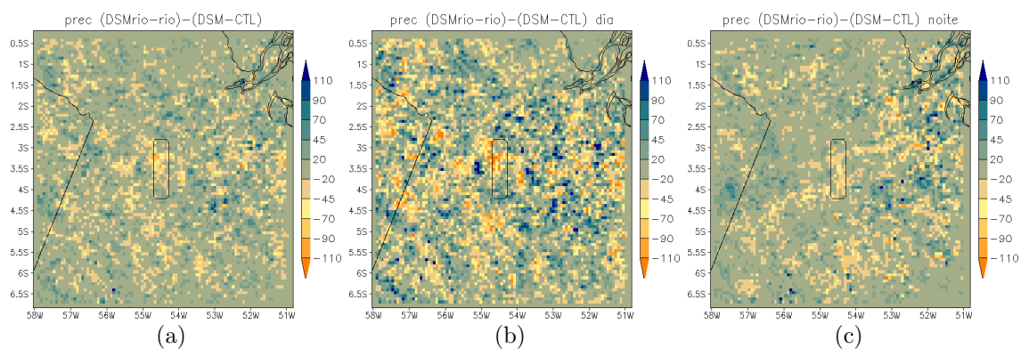
Figura 3.18: Diferença (DSM - CTL) da precipitação ( \text{mm mês}^{-1} ) para a expressão ((DSMrío-rio)-(DSM-CTL)), que corresponde a f'_{12} na Equação 3.2, (a) total, (b) para o período diurno, e (c) para o período noturno.
