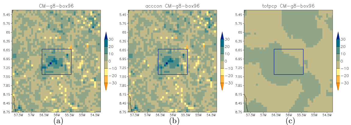
Figura 3.11: Diferença (DSM - CTL) da simulação CM-g8-box96 (com parametrização e com microfísica), de (a) precipitação total ( prec ), (b) precipitação da parametrização ( acccon ), e (c) precipitação da microfísica de nuvens ( totpcp ).
